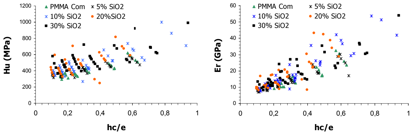
Figure III-12 : Influence de la composition sur a) la dureté, b) le module d'indentation pour des matériaux hybrides de classe I. Les propriétés mécaniques sont tracées en fonction de la profondeur de pénétration normalisée par l'épaisseur des couches minces
