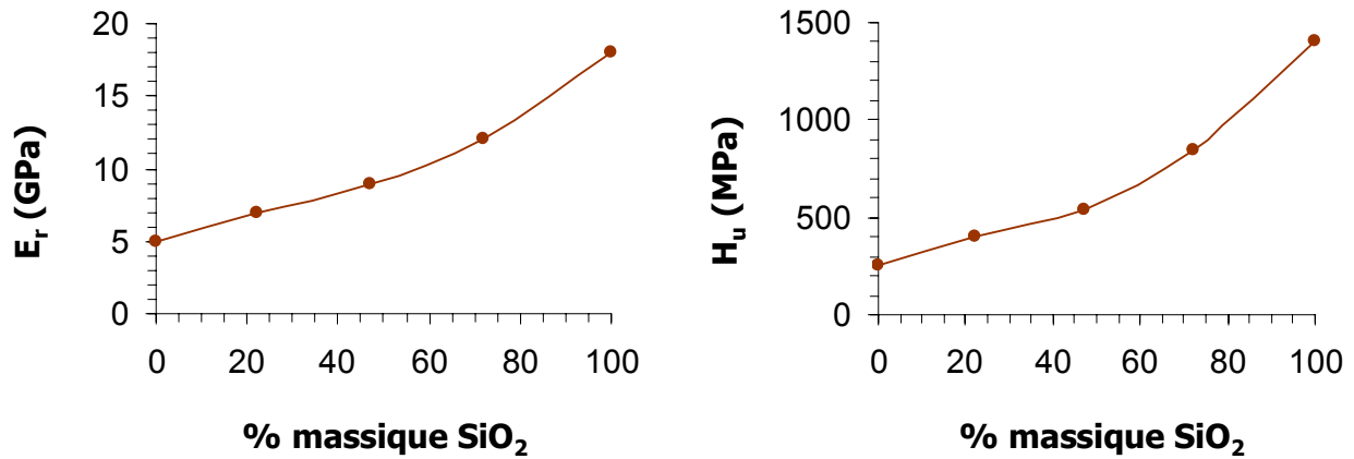
Figure II-24 : Evolution a) du module d'indentation, b) de la dureté en fonction de la fraction massique de PMMA fonctionnalisé à partir des valeurs extrapolées.
