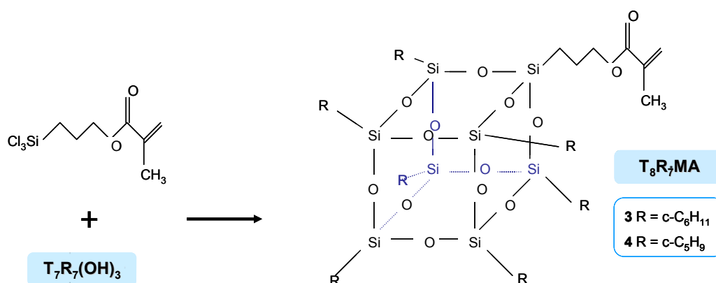
Figure III-23 : Schéma de synthèse du POSS méthacrylate (T 8 R 7 MA) à partir du POSS trisilanol incomplet T 7 R 7 (OH) 3
