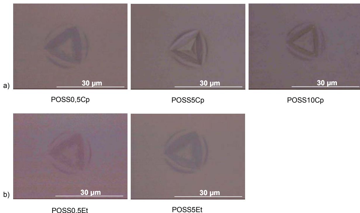
Figure III-30 : Observation, par microscopie optique, des empreintes résiduelles des copolymères PMMA-POSS après l'application d'une charge de 300 mN : a) POSS0,5Cp, POSS5Cp, POSS10Cp et b) POSS0,5Et, POSS5Et
