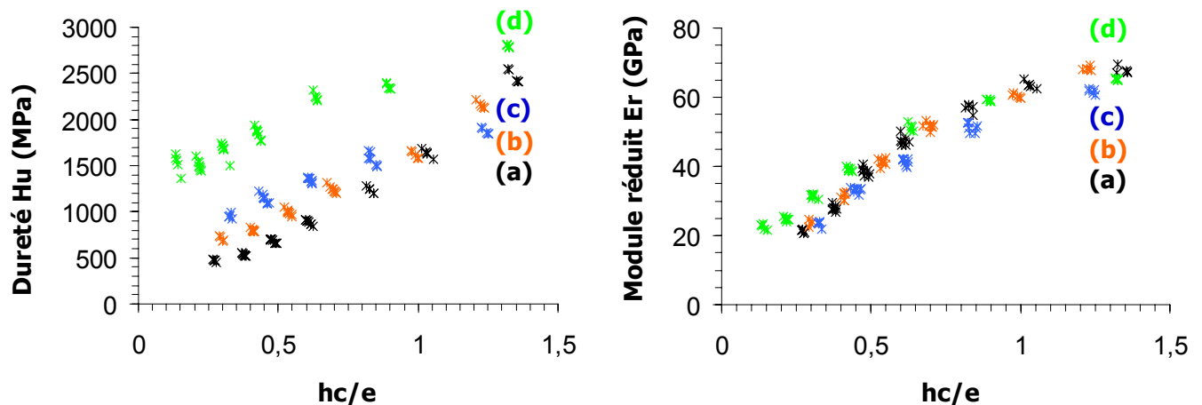
Figure II-35 : Influence de la composition sur la dureté et le module d'indentation pour des matériaux hybrides de classe II (préparés pour le test Taber) : a) PMMA fc , b) PMMA75, c) PMMA50, d) PMMA25.
