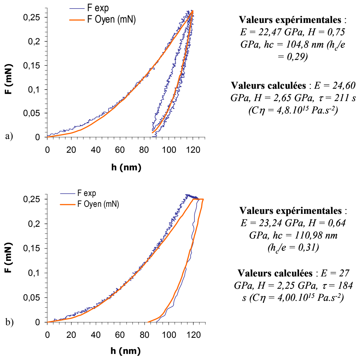
Figure II-31 : Courbes d'indentation de PMMA75 (SGR) obtenues par a) la procédure charge-recharge et b) par la procédure palier-décharge rapide. F_{\text{exp}} représente la courbe expérimentale et F_{\text{Oyen}} représente la courbe calculée par le modèle VEP.
