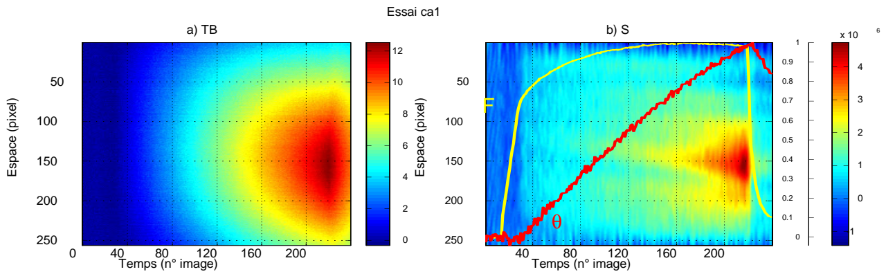
FIG. 1.12 – Essai ca1 (Acier DD14 - \dot{U}_{imp} = 0.15 \text{ mm.s}^{-1} ). Evolution au cours du temps (numéro d’image) d’un profil axial (numéro de pixel le long de la colonne centrale de la zone utile) : a) de l’écart de température ( ^{\circ}\text{C} ), b) des sources de chaleur ( \text{W.m}^{-3} ), F_{max} = 13.5 \text{ kN} , \theta_{max} = 13.1 \text{ K} .
