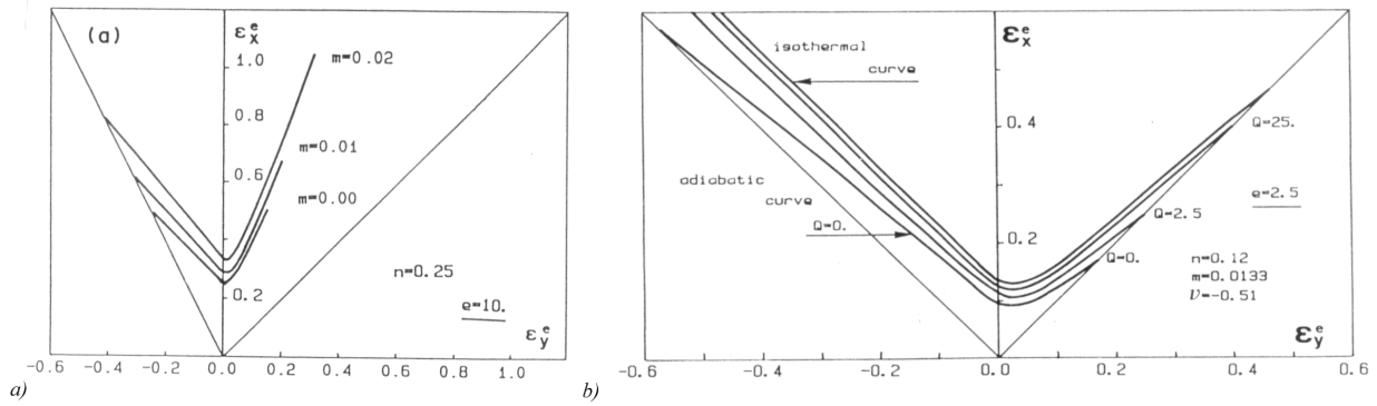
FIG. 3.3 – Tracé de CLF à partir d'une analyse de stabilité effective; effets stabilisants de : a) la sensibilité à la vitesse de déformation, b) la conduction thermique (figures extraites de [Dudzinski and Molinari 91]).
