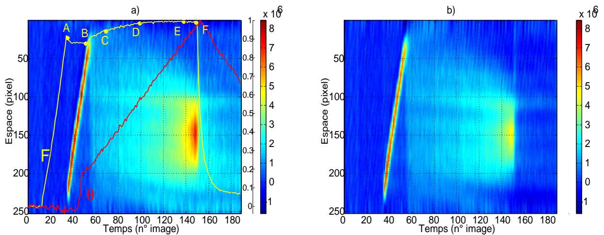
FIG. 1.6 – Essai aa6 (Acier S355MC - \dot{U}_{imp} = 0.15 \text{ mm.s}^{-1} ). Résultats du traitement: a) 2D (présenté sous la forme 1D), b) 1D. Image en arrière plan: évolution temporelle d'un profil axial de sources de chaleur; les couleurs jaune et rouge représentent des valeurs élevées des sources. Pour la figure a) les courbes en surimpression représentent: l'évolution de la charge et de la température (pixel 100) rapportée à une échelle normée par les valeurs maximales F_{max} et \theta_{max} données ci-après: F_{max} = 16.2 \text{ kN} \theta_{max} = 13.6 \text{ K} . Les points A,..., F correspondent aux images 36, 52, 70, 100, 139 et 150.
