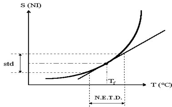
FIG. D.4 – Calcul du N.E.T.D. à partir de la mesure de l'écart-type std du bruit et de la courbe d'étalonnage.
