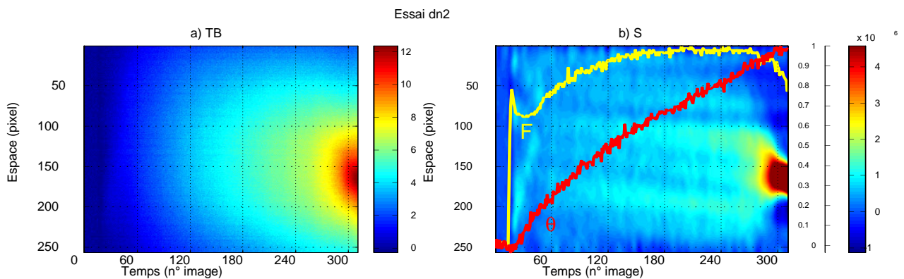
FIG. 1.13 – Essai dn2 (Acier M323brut - \dot{U}_{imp} = 0.15 \text{ mm.s}^{-1} ). Evolution au cours du temps (numéro d’image) d’un profil axial (numéro de pixel le long de la colonne centrale de la zone utile) : a) de l’écart de température ( ^{\circ}\text{C} ), b) des sources de chaleur ( \text{W.m}^{-3} ), F_{max} = 2.48 \text{ kN} , \theta_{max} = 7.2 \text{ K} ; seuillage des niveaux de couleurs à 35% de \text{Max}(w'_{ch}) .
