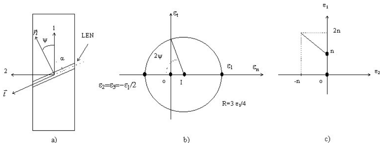
FIG. 4.2 – Etablissement du critère de Hill: a) schéma de l'éprouvette, b) cercle de Mohr des déformations, c) CLF obtenue avec le critère de Hill.
