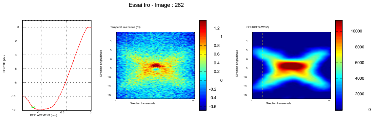
FIG. 4.10 – Essai tro (PVC - \dot{U}_{imp} = -0.003 \text{ mm.s}^{-1} ), d'une plaque de PVC trouée, de gauche à droite: réponse mécanique globale, image thermique et image des sources de chaleur à un instant du chargement (image n°262) correspondant à la phase d'adoucissement (marque '*' sur la réponse mécanique). Les effets thermiques et les sources de chaleur se distribuent dans des bandes inclinées ( \simeq 45^{\circ} ) issues du trou. La ligne en pointillé désigne la colonne 10.
