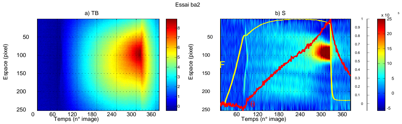
FIG. 1.11 – Essai ba2 (Acier HR55 - \dot{U}_{imp} = 0.04 \text{ mm.s}^{-1} ). Evolution au cours du temps (numéro d’image) d’un profil axial (numéro de pixel le long de la colonne centrale de la zone utile) : a) de l’écart de température ( ^{\circ}\text{C} ), b) des sources de chaleur ( \text{W.m}^{-3} ), F_{max} = 24.5 \text{ kN} , \theta_{max} = 9.0 \text{ K} , seuillage des niveaux de couleurs à 50% de \text{Max}(w'_{ch}) .
