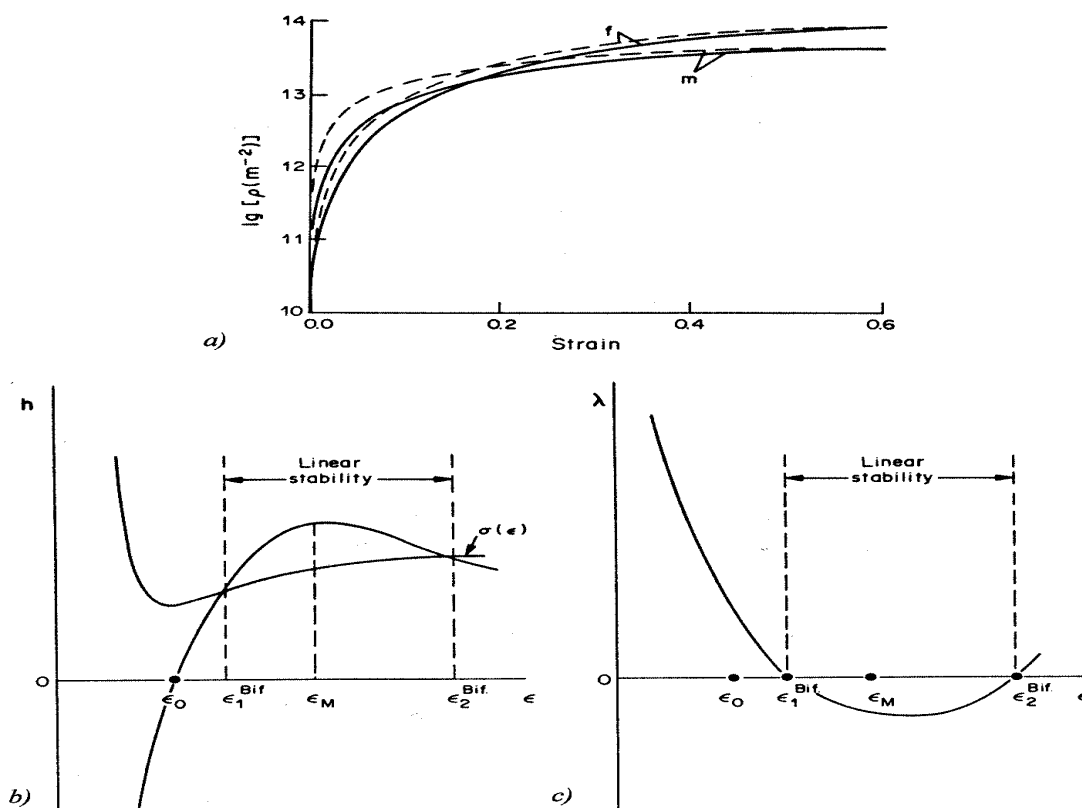
FIG. 5.2 – a) Evolutions (trais épais) des densités de dislocations mobiles \rho_m et fixes \rho_f au cours de la déformation, b) Evolution du module d'écrouissage h et de la contrainte \sigma , c) Evolution du paramètre \lambda indicateur de stabilité/instabilité, (figures extraites de [Estrin and Kubin 86]).
