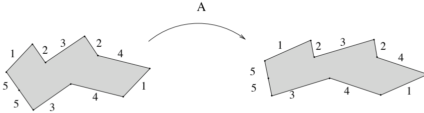
FIG. 4 – Action de SL_2(\mathbb{R}) sur une surface plate.
