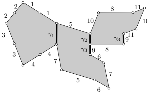
FIG. 6 – Connexions de selles deux à deux \hat{h} omologues sur une surface plate.
