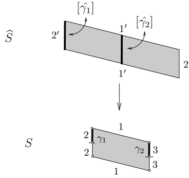
FIG. 5 – Deux connexions de selles \hat{\gamma} homologues sur une surface plate.
