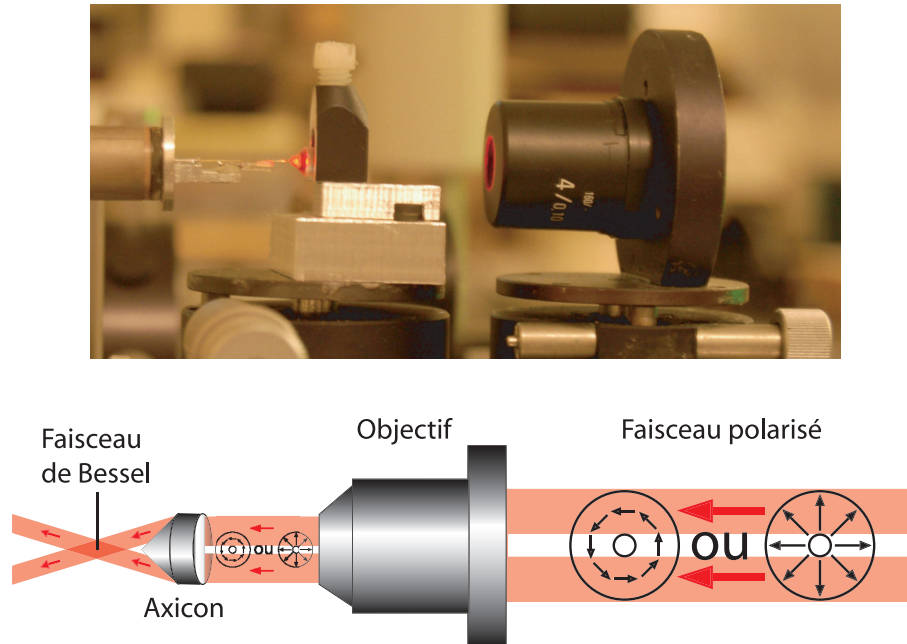
FIG. 6. Création d'un faisceau de Bessel polarisé.
