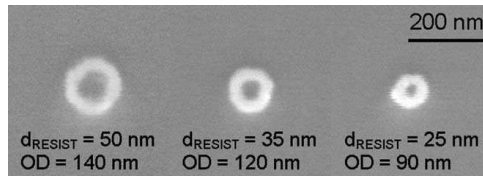
FIG. 18. Anneaux en Permalloy (épaisseur 10 nm) fabriqués par lithographie e-beam [76]. Les diamètres externes (OD), dépendant de l'épaisseur de résine PMMA avant l'insolation ( d_{resist} ), sont donnés pour chaque figure.
