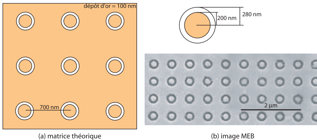
FIG. 17. (a) Représentation schématique de la matrice de coaxes et dimensions caractéristiques.
