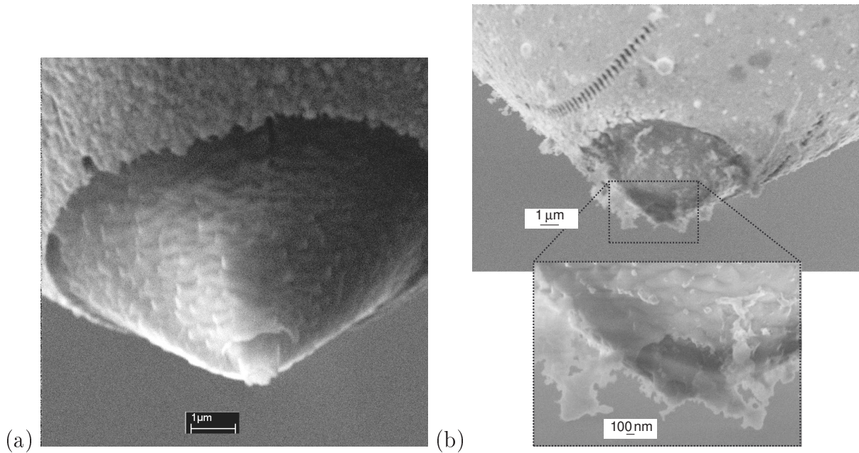
FIG. 12. Détérioration d'une nano-antenne (pointe 1) : (a) avant utilisation (jour 1) ; (b) après utilisation (jour 3).
