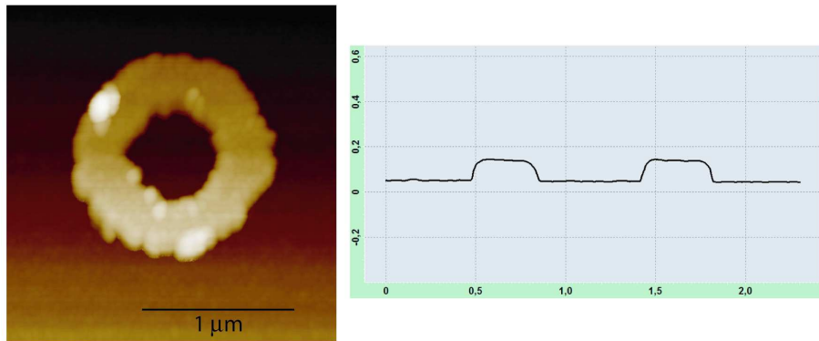
FIG. 16. Image AFM et coupe d'un anneau obtenu par lithographie e-beam.
