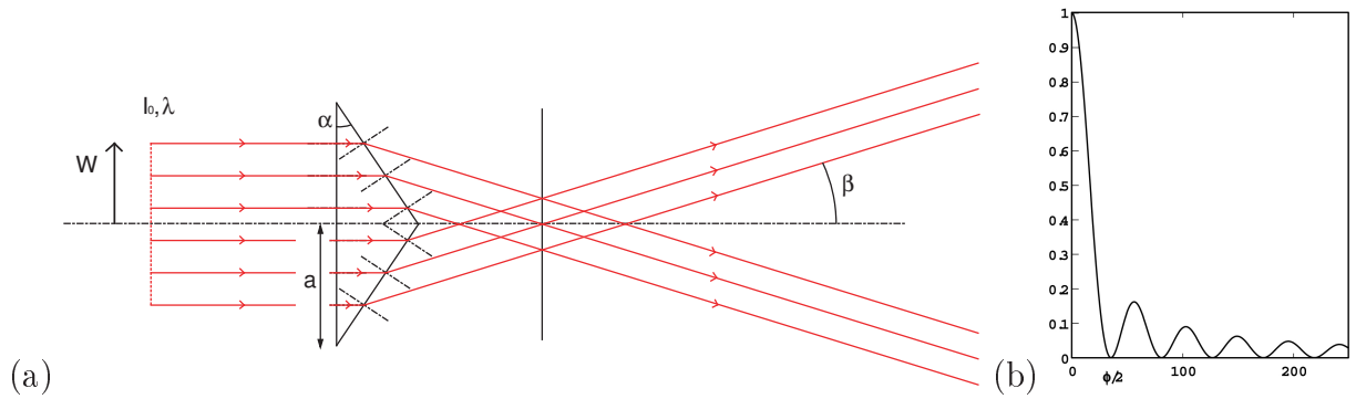
FIG. 9. (a) Recouvrement des faisceaux à la sortie d'un axicon. (b) Coupe d'un faisceau de Bessel.
