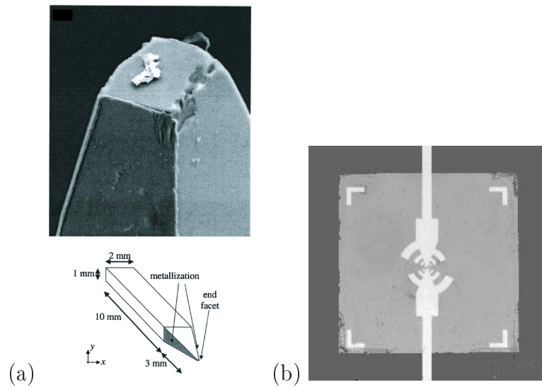
FIG. 6. Antennes pour la microscopie TéraHertz : (a) pointe pyramidale [90], (b) AMCB sur une membrane de Si_3N_4 d'épaisseur 500 nm et 2 \mu m de côtés [64].
