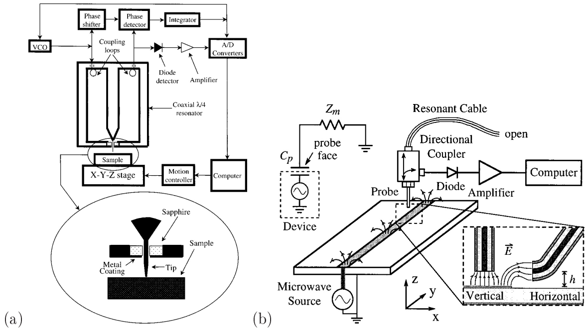
FIG. 4. Exemples de sondes adaptées à la microscopie micro-onde en champ proche :
