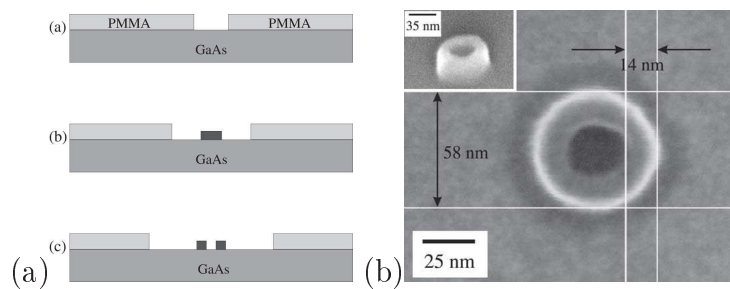
FIG. 17. Anneaux de résine fabriqués par lithographie e-beam [22]. (a) Processus de fabrication et (b) image MEB.
