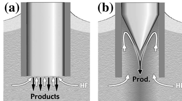
FIG. 3. Principe du tube etching [140] :
