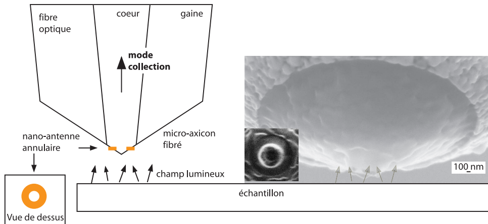
FIG. 15. Principe de la sonde collectrice munie d'une nano-antenne annulaire (SNOM).
