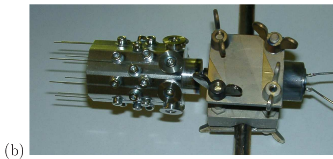
FIG. 20. Procédé de métallisation des pointes :
