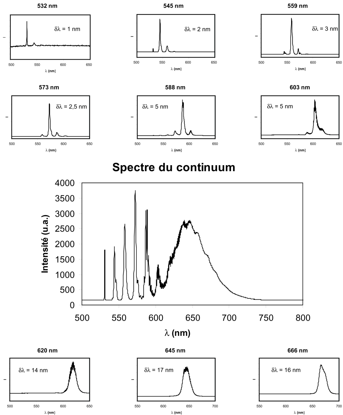
FIG. 3. Spectres relevés.
