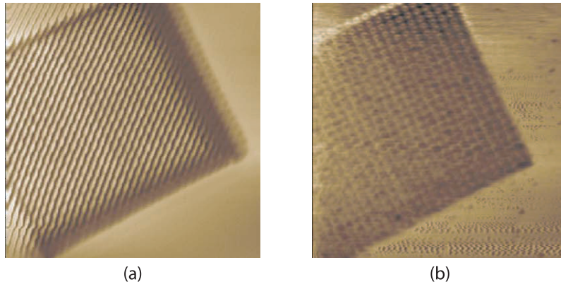
FIG. 16. Images ( 13 \mu\text{m} \times 13 \mu\text{m} ) optique (a) et topographique (b) d'une matrice de coaxes obtenues avec une pointe diélectrique étirée [125].
