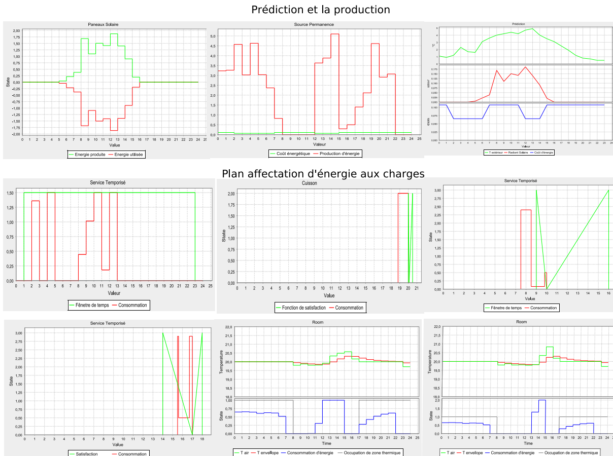
FIG. 10.5 – Résultats d'affectation des ressources d'énergie dans le mode de confort avec la stratégie de consommation locale de l'énergie produite
