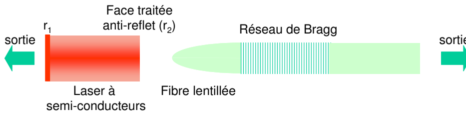
FIG. 8.1 – Représentation schématique d'une cavité étendue
