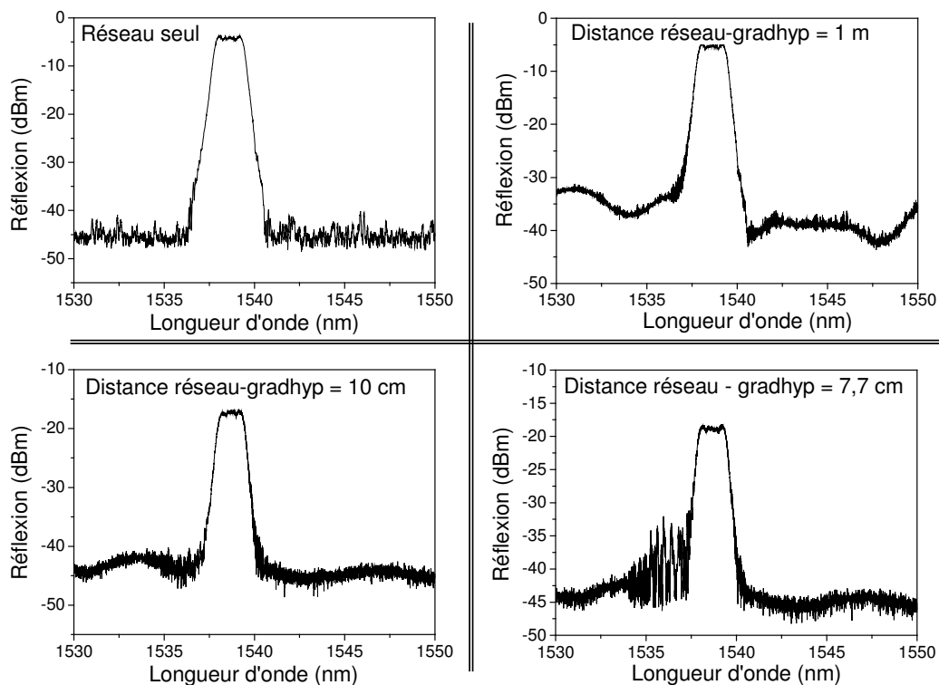
FIG. 6.30 – Evolution de l’allure de la courbe de réflexion d’un réseau de Bragg associé à une micro-lentille lorsque la taille de la cavité externe diminue.
