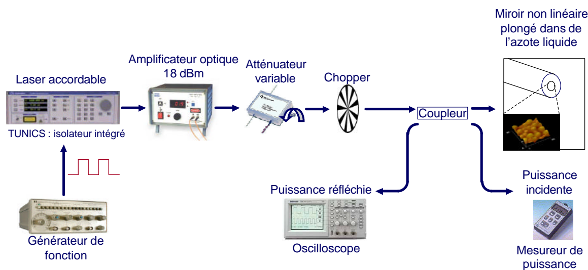
FIG. 4.10 – Montage expérimental utilisé pour la caractérisation de la réponse des miroirs de gallium déposés en bout de fibre optique.
