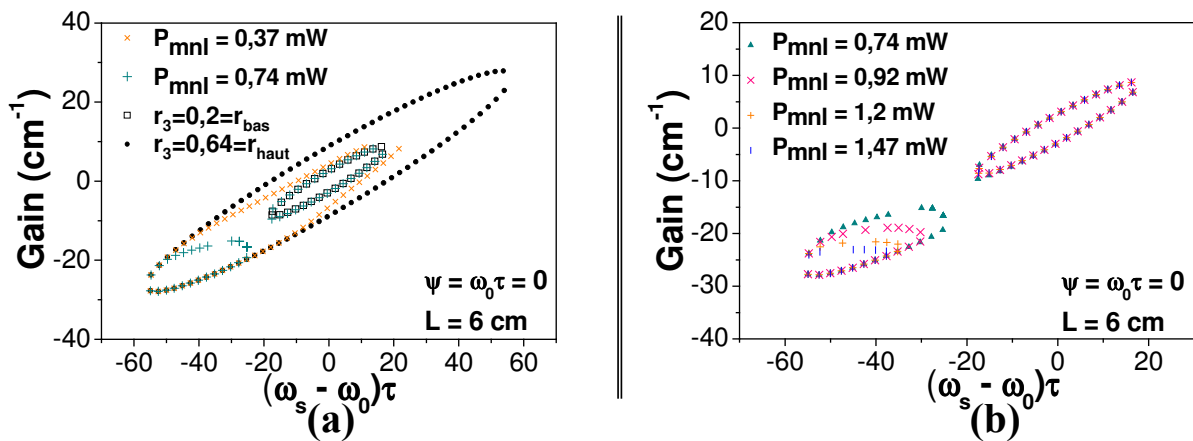
FIG. 5.3 – Répartition des solutions stationnaires dans le plan (fréquence, gain). (a) Laser contre-réactionné par un miroir classique ( r_3 = 0,64 et 0,2 ) et un miroir non linéaire ( r_{bas} = 0,2 et r_{haut} = 0,64 ). (b) Influence de la puissance de seuil d'un miroir non linéaire ( r_{bas} = 0,2 et r_{haut} = 0,64 ) sur la répartition des modes de la cavité externe.
