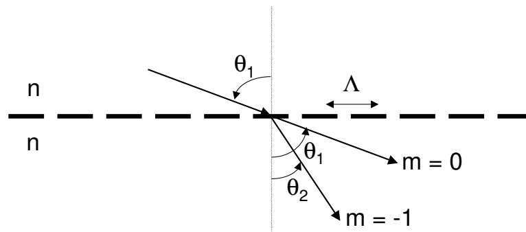
FIG. 8.3 – Diffraction d'une onde par un réseau.
