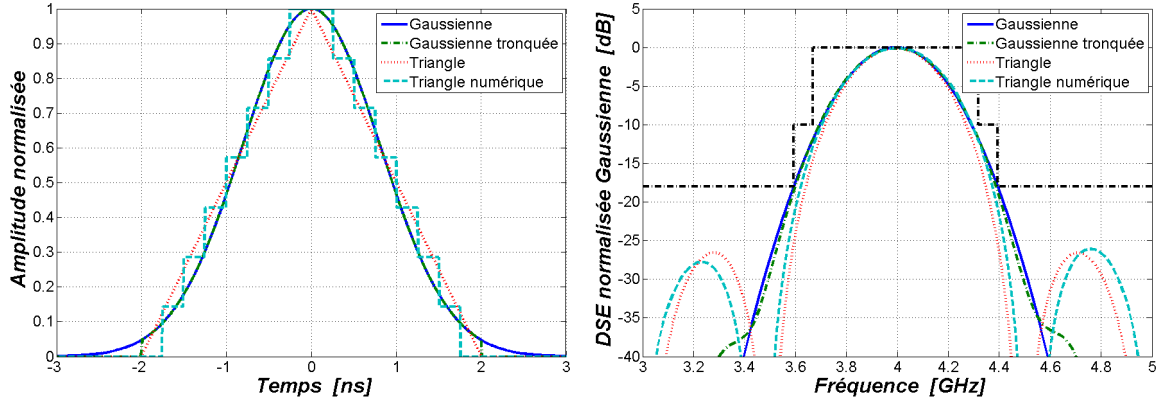
FIG. II.14: Processus d'adaptation de la Gaussienne vers l'implémentation
