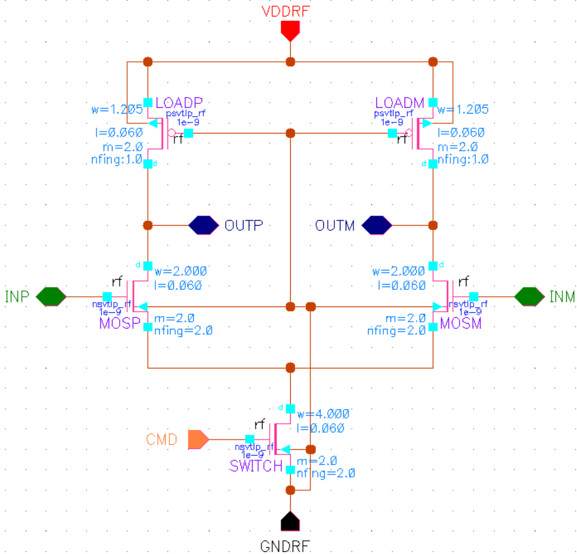
FIG. III.5: Schéma électrique d'une cellule élémentaire du DAC RF
