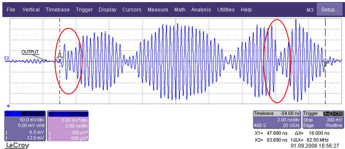
FIG. III.19: Mesure à l'oscilloscope d'un burst codé [-1\ 0\ +1\ +1\ 0\ -1\ +1\ 0] – F_{DIG} = 4\text{ GHz}
