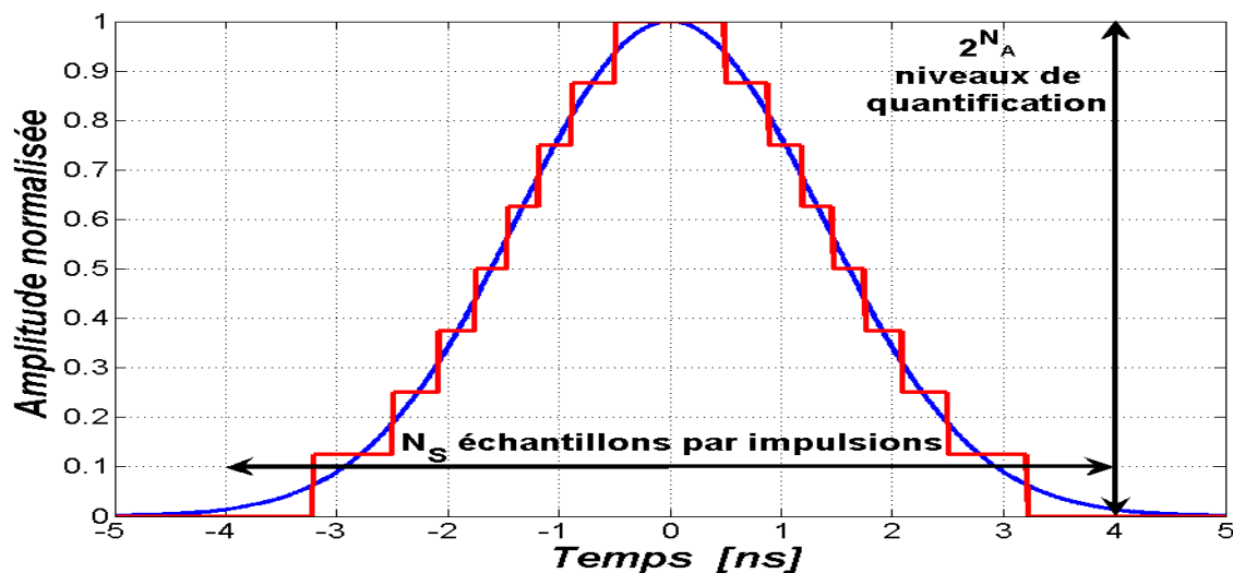
FIG. II.6: Grandeurs de quantification de l'impulsion bande de base
