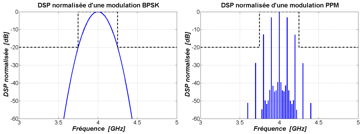
FIG. II.12: Comparaison des DSPs des modulations BPSK et PPM – RBW = 200\text{kHz}
