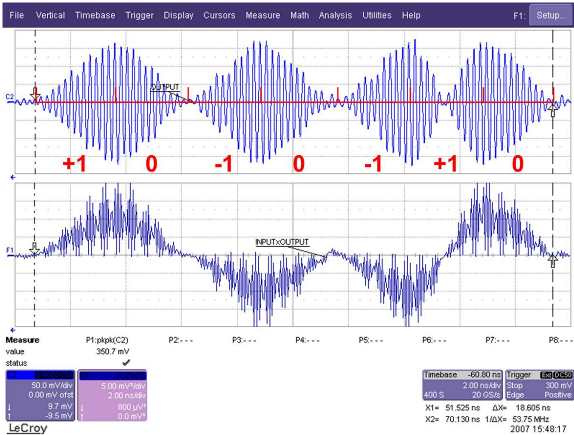
FIG. III.20: Mesure à l'oscilloscope d'un burst codé [+1\ 0\ -1\ 0\ -1\ +1\ 0] – F_{DIG} = 3\text{ GHz}
