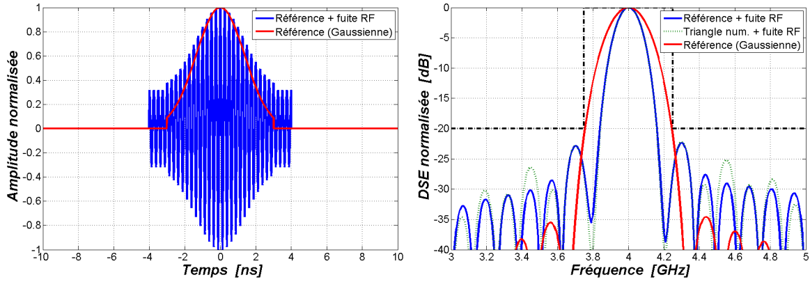
FIG. II.9: Exemple d'impulsion pour T_{OL} = 8 ns et une isolation de 10 dB
