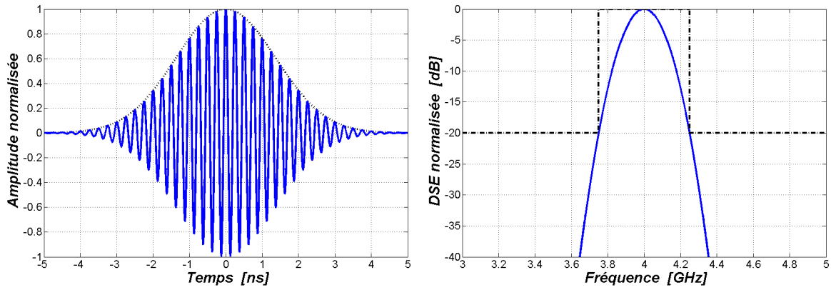
FIG. II.4: Impulsion Gaussienne transposée en fréquence – f_0 = 4 GHz et \tau = 1.366 ns
