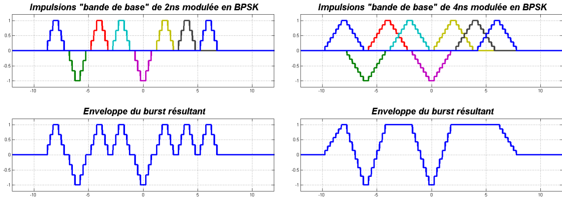
FIG. II.17: Comparaison d'un burst généré à partir d'impulsions de 2 ns et 4 ns
