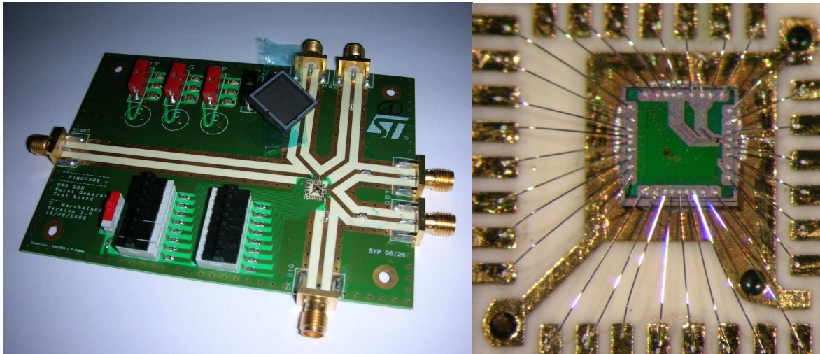
FIG. III.18: Photographies du PCB et de la puce montée sur ce dernier
