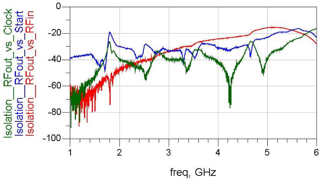
FIG. III.22: Mesure des couplages PCB des différentes entrées vers la sortie RF
