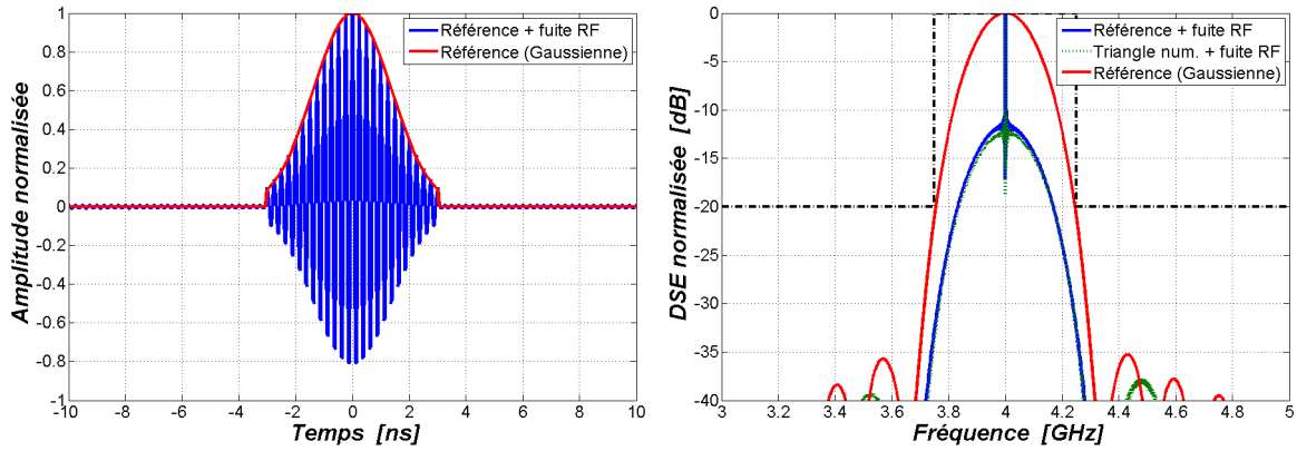
FIG. II.8: Exemple d'impulsion pour \text{PRF} = 1 \text{ MHz} et une isolation de 40 dB
