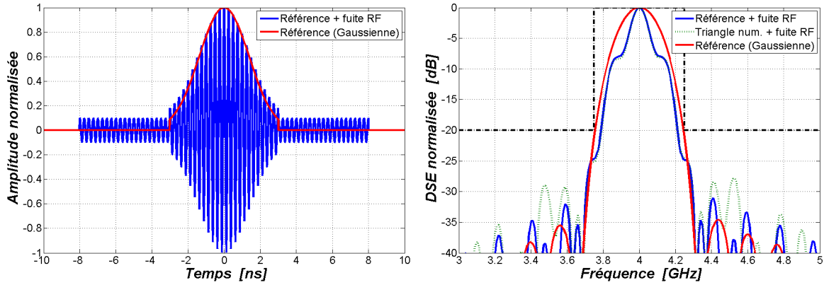
FIG. II.10: Exemple d'impulsion pour T_{OL} = 16 ns et une isolation de 20 dB
