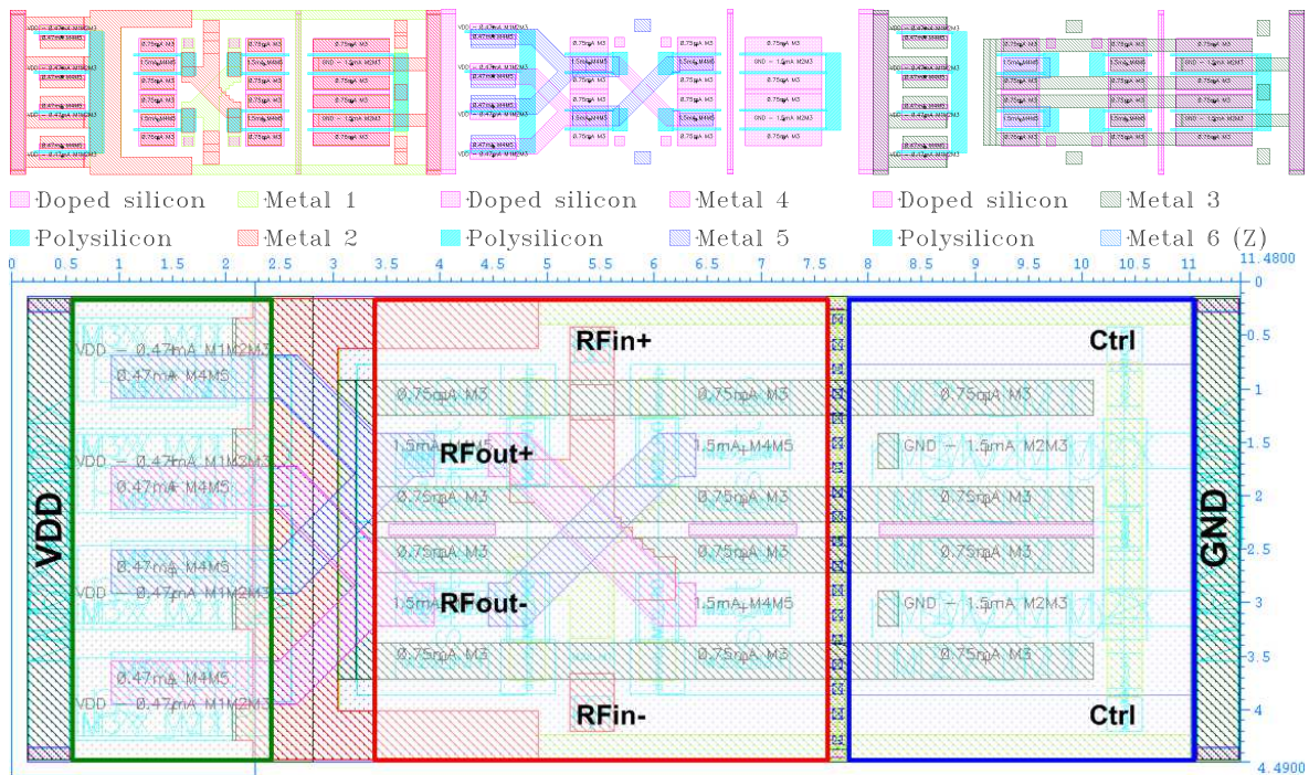
FIG. III.8: Routage des niveaux de métallisation et layout global de la cellule élémentaire
