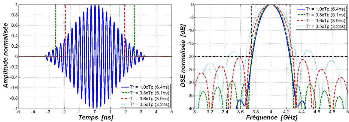
FIG. II.5: Allures de l'impulsion pour différentes troncatures
