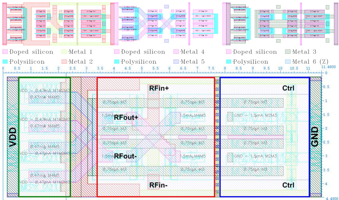
FIG. III.8: Routage des niveaux de métallisation et layout global de la cellule élémentaire
