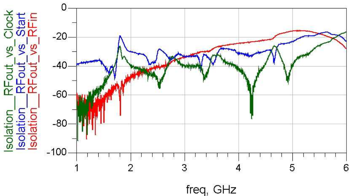
FIG. III.22: Mesure des couplages PCB des différentes entrées vers la sortie RF
