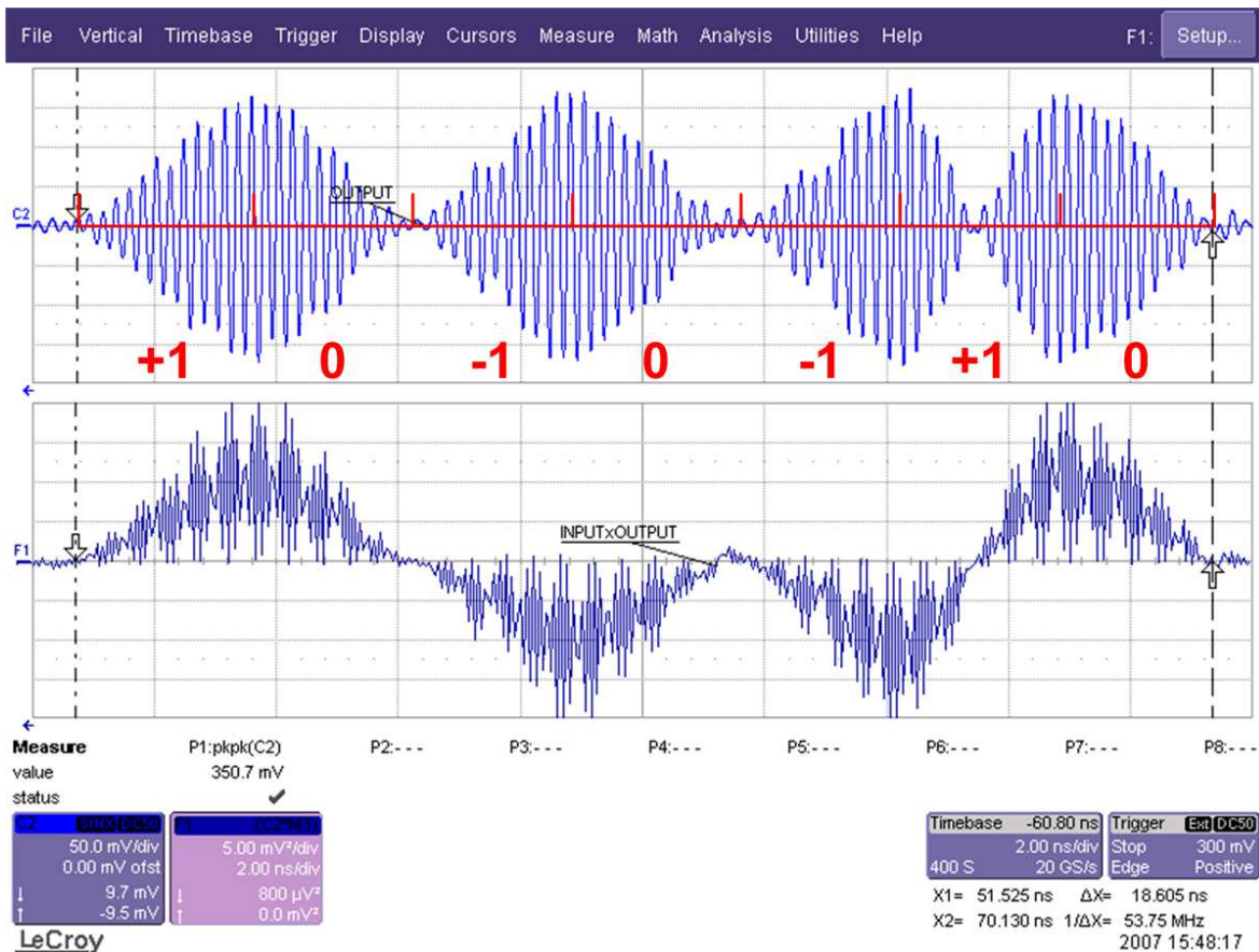
FIG. III.20: Mesure à l'oscilloscope d'un burst codé [+1 0 -1 0 -1 +1 0] – F_{DIG} = 3 GHz
