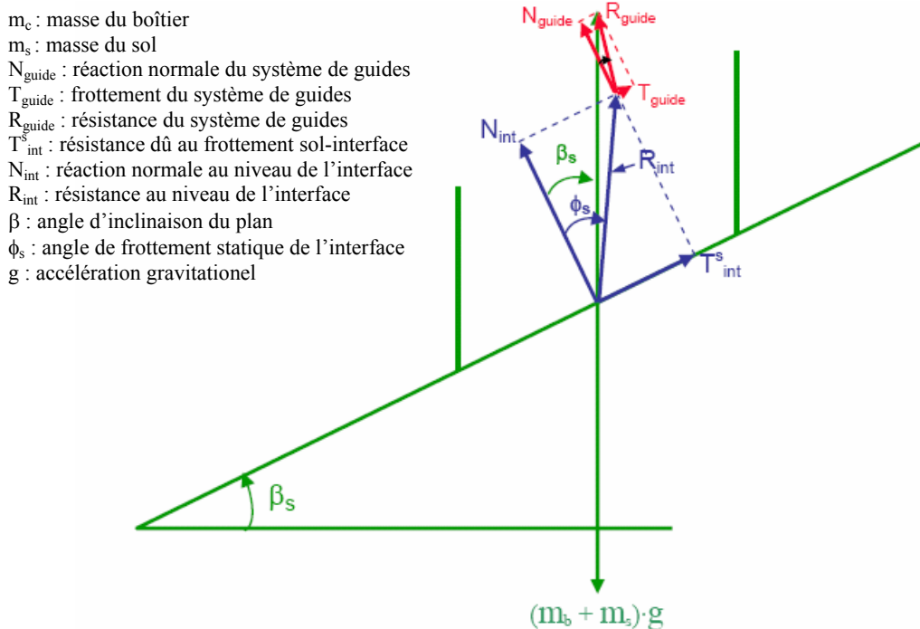
Figure 6.5. Équilibre statique limite du boîtier supérieur.
