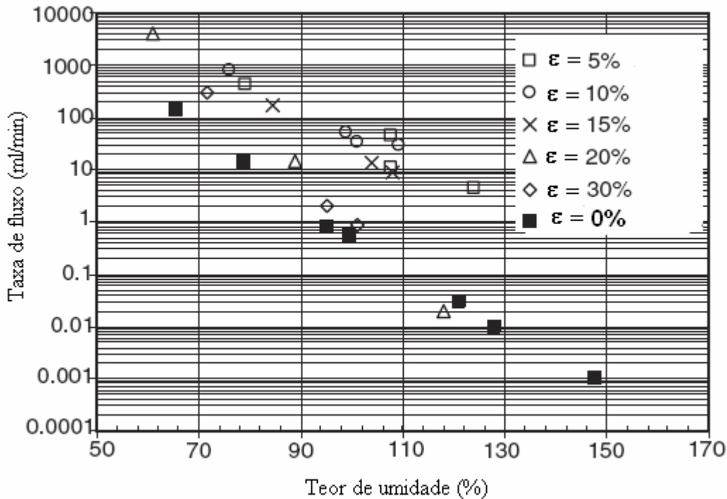
Figura 3.12. Variação da taxa de fluxo do gás azoto com o teor de umidade de amostras de GCL previamente deformadas na condição hidratada (Bouazza & Vangpaisal, 2004).
