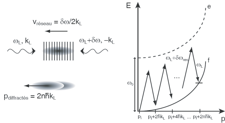
FIG. 5.13 – Diffraction de Bragg à 2n photons. A gauche : deux faisceaux laser contra-propageants créent le réseau optique sur lequel est diffractée l’onde de matière. A droite : diagramme des états d’impulsion couplés par des processus à 2n photons.
