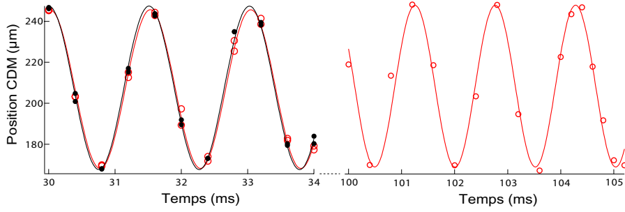
FIG. 5.7 – Oscillations dipolaires dans la direction transverse Ox en l'absence (ronds noirs \bullet ) et en présence d'un potentiel aléatoire 1D d'amplitude \gamma = 0.4 (cercles rouges \circ ). Les courbes en trait plein correspondent à un ajustement des données expérimentales avec une fonction sinusoïdale du temps.
