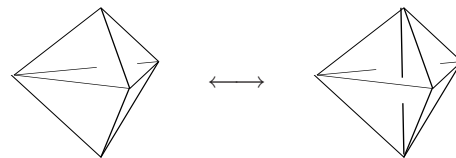
Figure 2.15: mouvement de Pachner (2-3)
