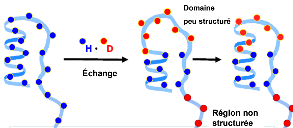
Figure 78 : Schéma des échanges H/D au niveau des protons amides d'une protéine. Les hydrogènes amides sont représentés en bleu sur la protéine hydrogénée.
