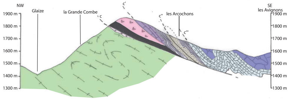
Coupe 2
