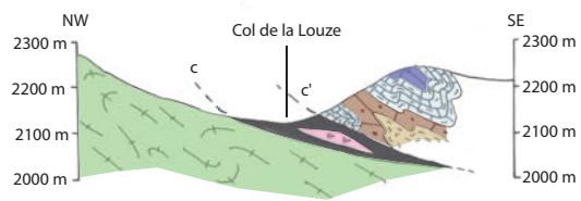
Coupe 1
