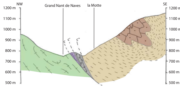
Coupe 3
