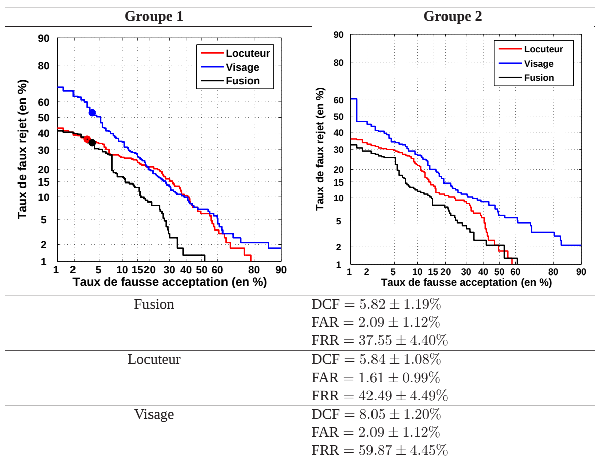
FIG. 3.14 – Performances du système locuteur+visage
