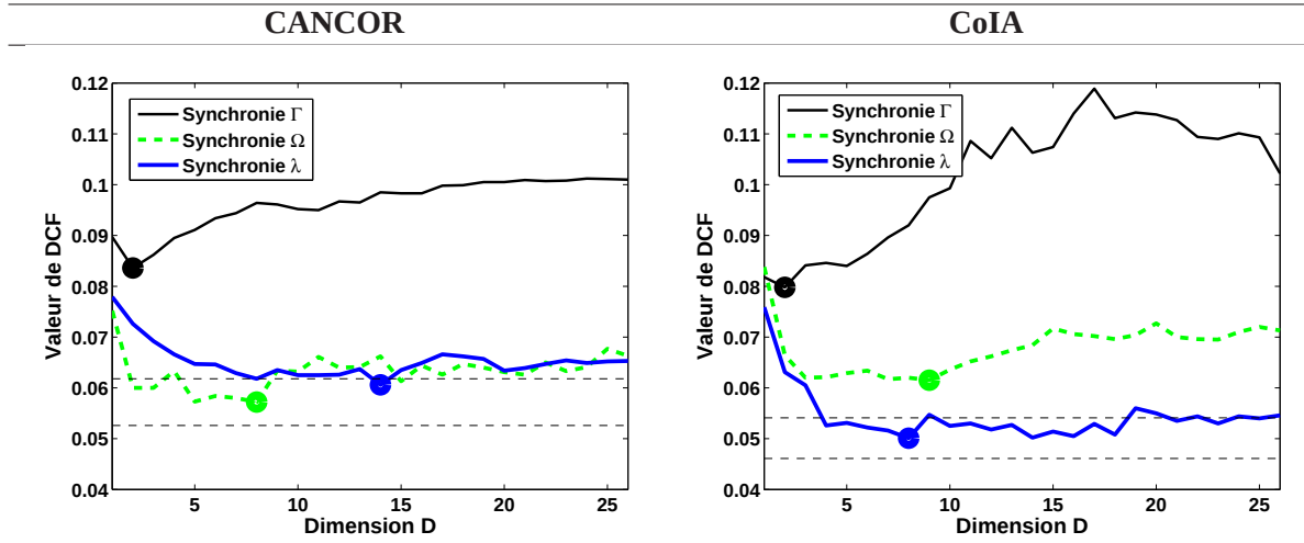
FIG. 6.9 – Comparaison des mesures basées sur CANCE et CoIA. Les points • indiquent les meilleurs systèmes pour chaque configuration. Les lignes noires horizontales en pointillés indiquent l'intervalle de confiance à 95% sur la valeur de DCF des meilleures mesures CANCE ( \Omega ) et CoIA ( \lambda ).
