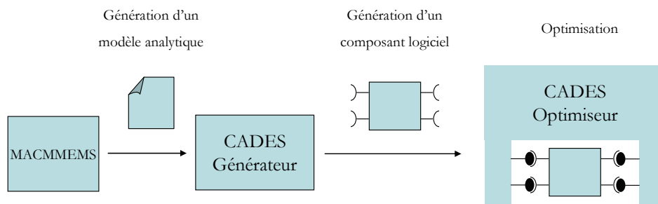
Figure 2.15 Etapes d'optimisations.
