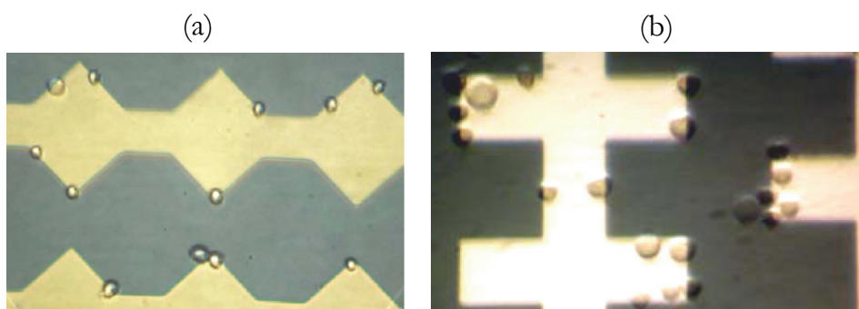
Figure 1.3 (a-b) Cellules Jurkat attirées vers le bord des électrodes sous l'effet de la diélectrophorèse positive.
