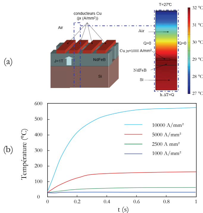
Figure 4.18 (a) Simulation de la répartition de l'échauffement produit par une densité de courant de 1 kA/mm 2 , (b) dynamique de l'évolution de la température au sein des conducteurs pour diverses valeurs de densités.
