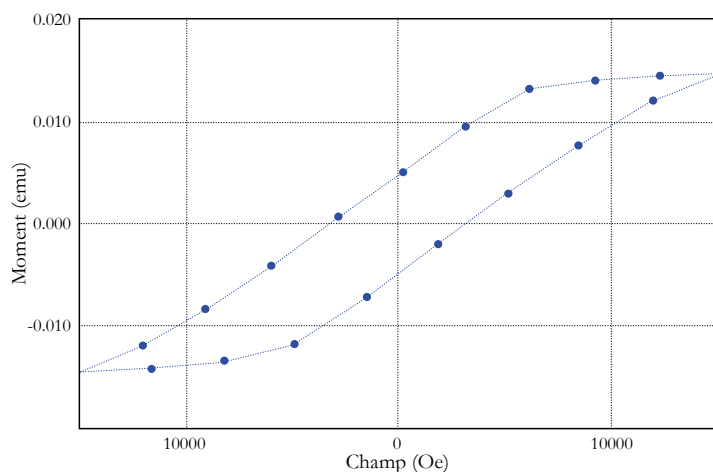
Figure 5.5 Courbe hystérésis du CoPt obtenue par VSM.
