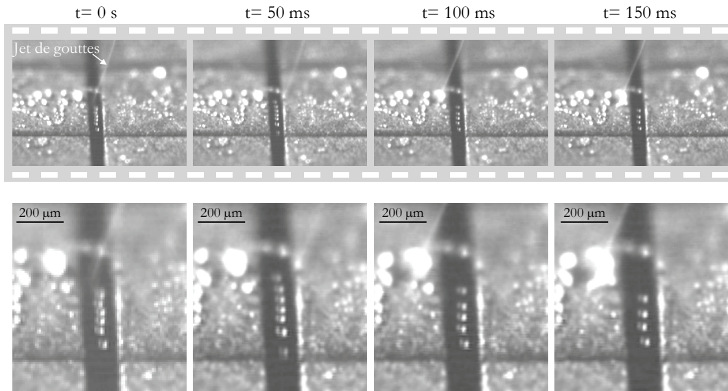
Figure 6.8 Gouttelettes qui lévitent le long d'une rainure et qui tombent au niveau du croisement.
