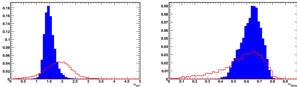
Fig. 7.26: Largeur totale de la gerbe \omega_{tot1} (à gauche) et dans trois strips \omega_{3strips} (à droite) dans le premier compartiment du calorimètre électromagnétique. Les distributions sont montrées pour des pions et pour des électrons (histogramme plein), dans le lot de données à 9 GeV. Elles sont normalisées à l'unité.
