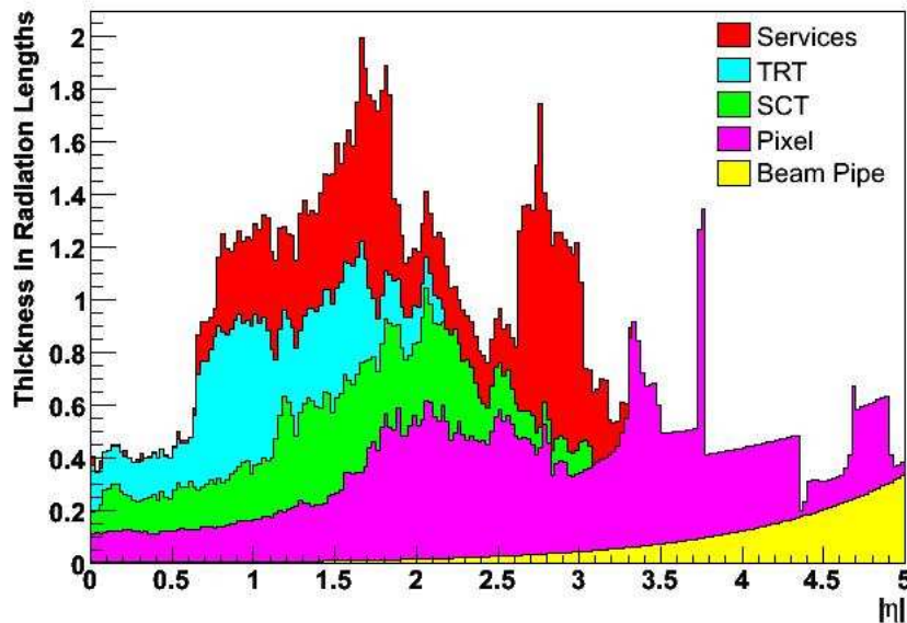
Fig. 1.5: Distribution de matière (en X_0 ) à la sortie du détecteur interne dans la géométrie dite "CSC". La distribution est montrée en fonction de \eta , intégrée en azimuth.
