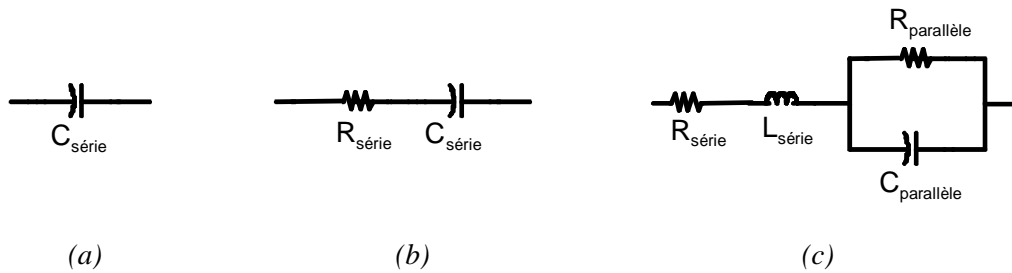
Fig. IV.2. Modèles utilisables pour l'extraction de la capacité équivalente à la structure interdite : (a) capacité série, (b) modèle R-C série et (c) modèle avec prise en compte des effets inductifs.
