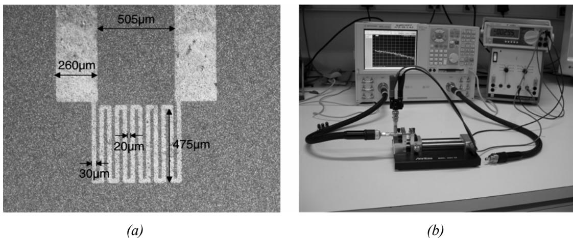
Fig. V.10. (a) Exemple de capacité interdigitée en réflexion réalisée sur \text{KTa}_{0,5}\text{Nb}_{0,5}\text{O}_3/\text{saphir} et (b) photographie du dispositif de mesure utilisé pour les caractériser.
