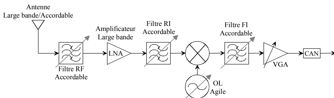
Fig. I.3. Schéma bloc d'un récepteur utilisant la radio logicielle restreinte.
