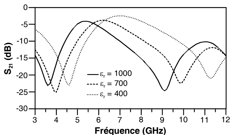
Fig. V.22. Réponse en transmission simulée d'un résonateur DBR pour différentes valeurs de permittivité du film ferroélectrique ( \epsilon_{r\text{KTN}} = 400, 700 et 1000 ).
