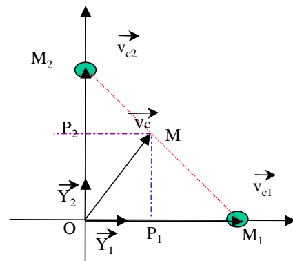
Figure 10, recherche des coordonnées barycentriques \frac{t_1}{T} et \frac{t_2}{T} de M dans le repère (M_1, M_2)
