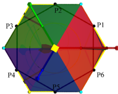
Figure 46, représentation du domaine d'excursion autorisé [P_1, P_2, P_3, P_4, P_5, P_6] pour \overrightarrow{v_c}
