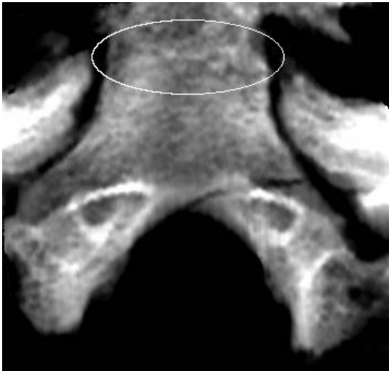
Figure 30 : radiographie de la partie basilaire du crâne de NK 2, au niveau de la synchondrose sphéno-occipitale.
