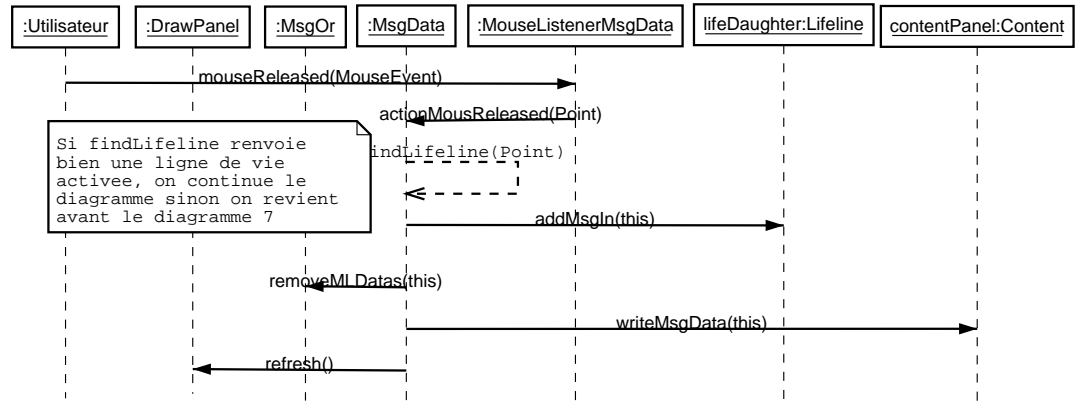
FIG. A.16 – Séquence du relâchement du bouton après l'étirement
