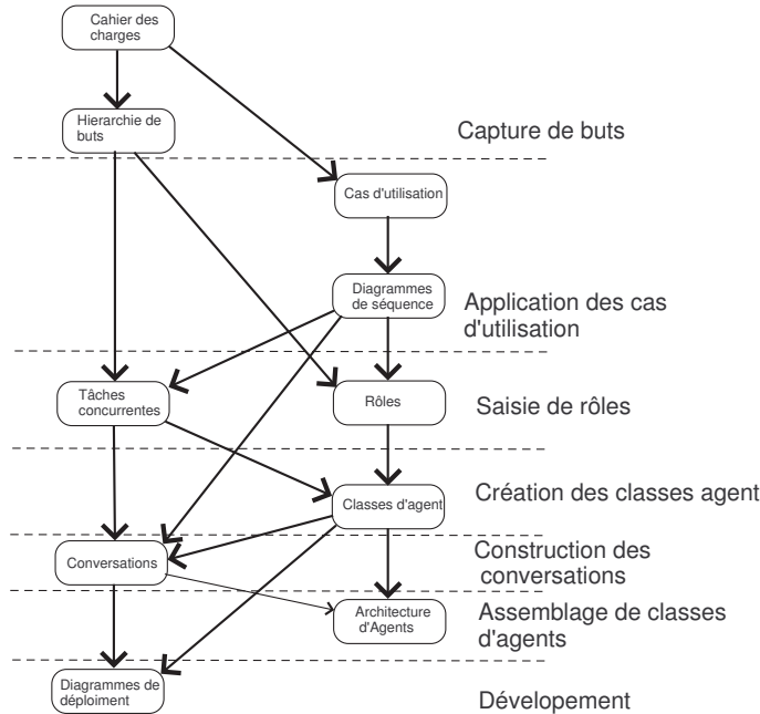
FIG. 2.5 – Schéma générale de la méthodologie MaSE
