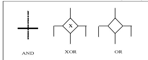
FIG. 3.9 – Diagramme AUML (XOR)
