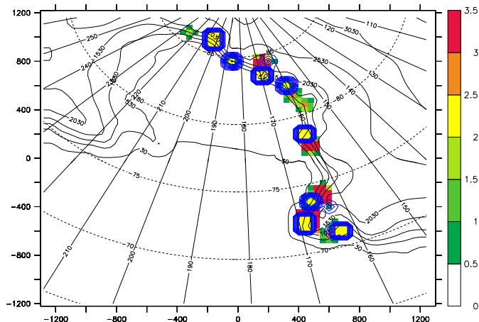
FIG. 3.6: Différence de longueur de rugosité (en m) entre une simulation dont le 1 er niveau est à 10 m et une simulation dont le 1 er niveau est à 3 m, pour \Delta x = 40 \text{ km} , h_0 = 100 \text{ m} . Les contours bleus sont les isomètres de la longueur de rugosité de la simulation dont le 1 er niveau est à 3 m.
