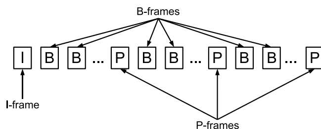
FIG. 1.4 – Structure d'un GOP
