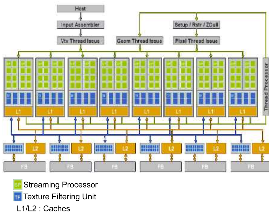
FIG. 3.7 – Diagramme blocs du GeForce 8800 GTX
