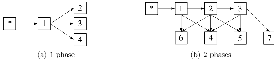
FIG. 2.11 – Schémas des dépendances pour l’estimation de mouvement avec “vector-tracing” 1 phase (a) et 2 phases (b). Les informations notées “*” viennent de l’estimation de mouvement de la dernière image du GOP précédent.
