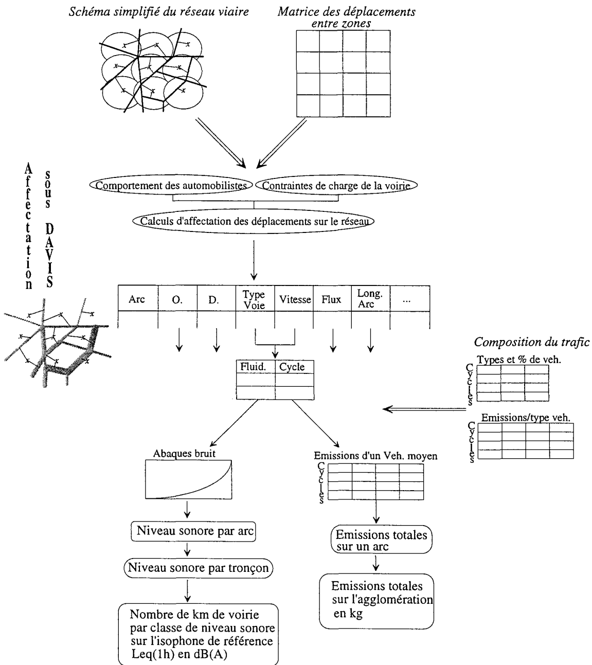
Graphique 6 : Le déroulement de la méthode de calcul des émissions polluantes et sonores du trafic routier
