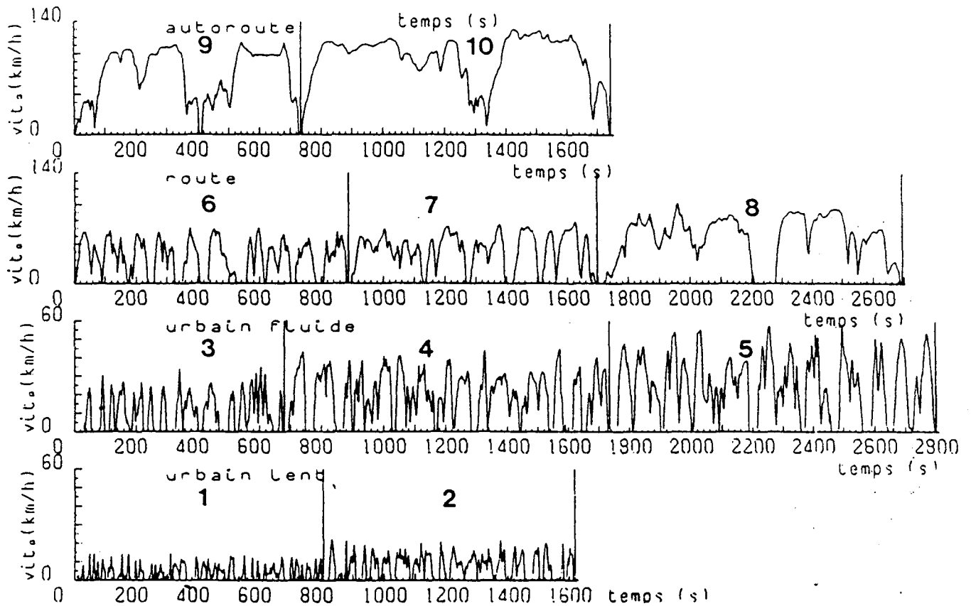
Graphique 4 : Représentation des 10 cycles de conduite INRETS à partir des vitesses instantanées 15
