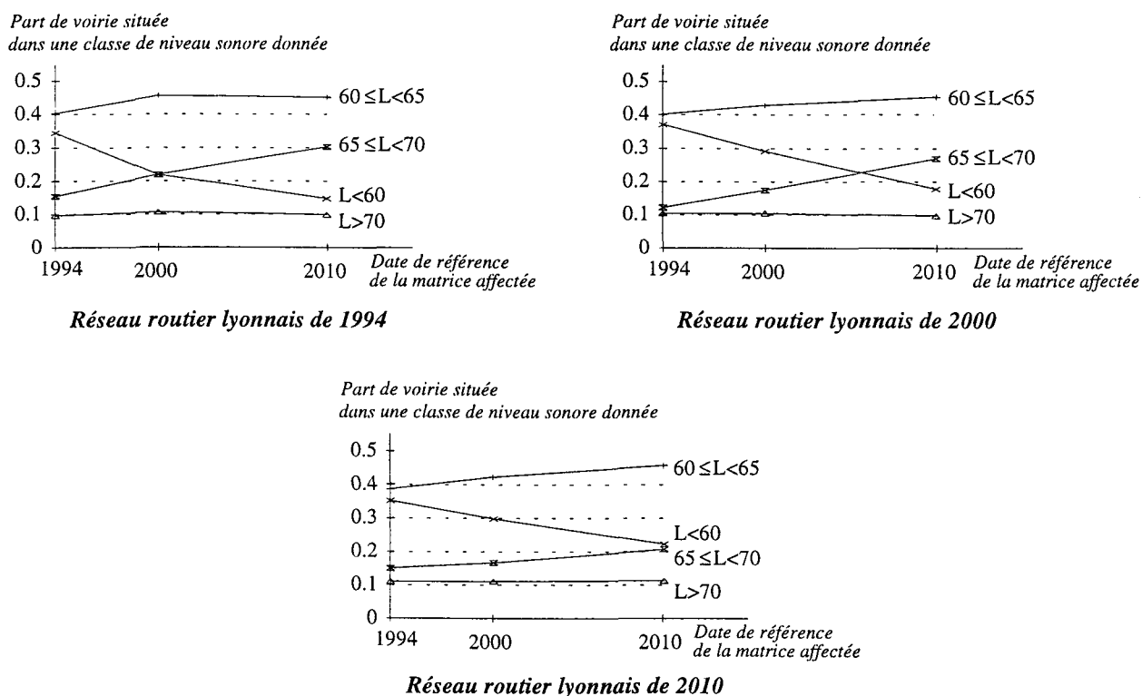
Graphique 6 : Impact de l'évolution des hypothèses d'évolution de la mobilité automobile sur les émissions sonores à réseau constant
