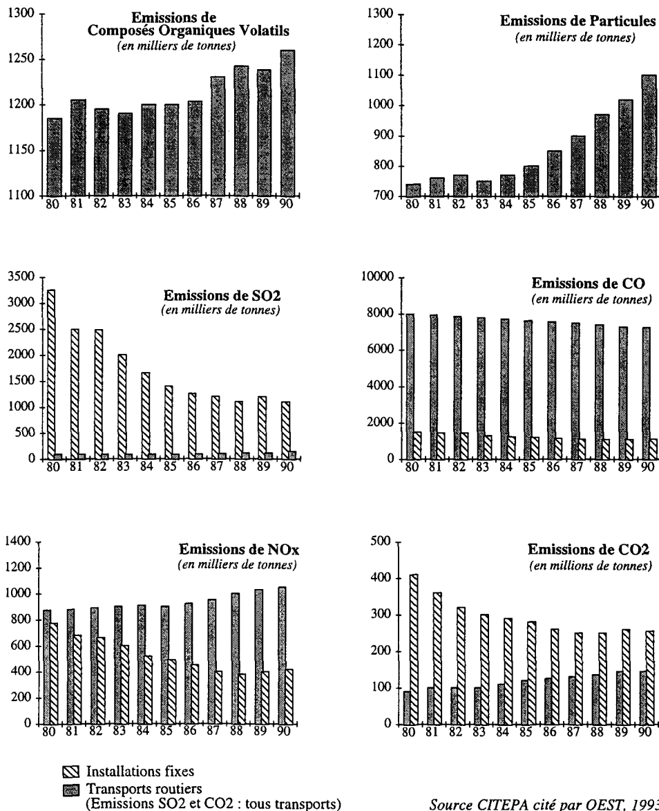
Graphique 1 : Evolutions des émissions de polluants atmosphériques par les transports routiers 10
