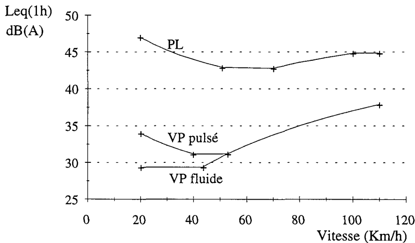
Graphique 5 : Emissions sonores d'un véhicule en conditions de circulation fluide ou pulsée
