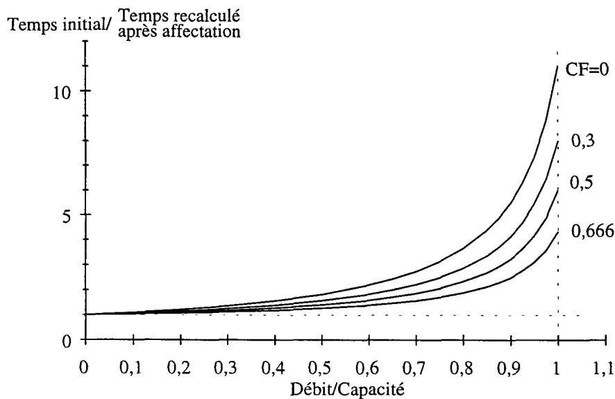
Graphique 2 : Courbes standard Coût-Débit sous DAVIS
