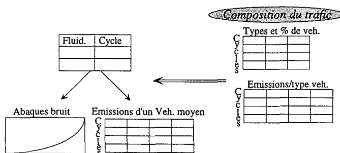
Graphique 9 : Situation des paramètres testés dans la procédure de calcul
