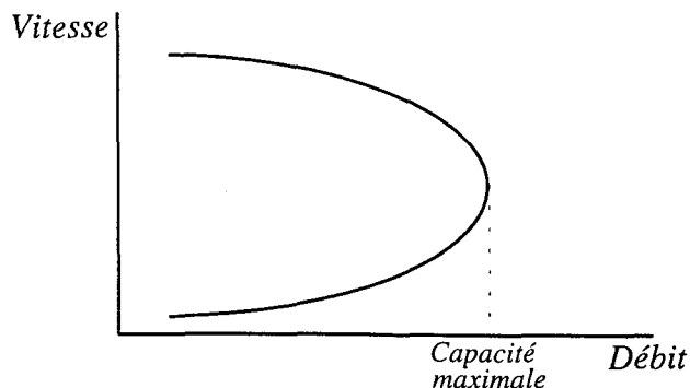
Graphique 2 : la relation entre vitesse et débit sur un axe routier
