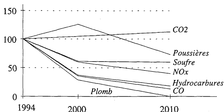
Graphique 4 : Effet de l'évolution de la composition du trafic à mobilité et réseau constants (1994) sur les émissions de polluants atmosphériques
