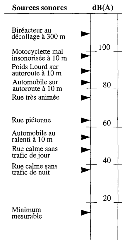
Graphique 3 : Illustration des niveaux de bruit
