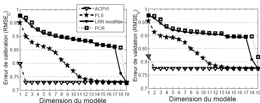
FIG. 5.9 – Erreur moyenne de calibration ( RMSE_C ) et de validation ( RMSE_V ) pour les méthodes ACPVI , régression PLS , LRR modifiée et PCR .
