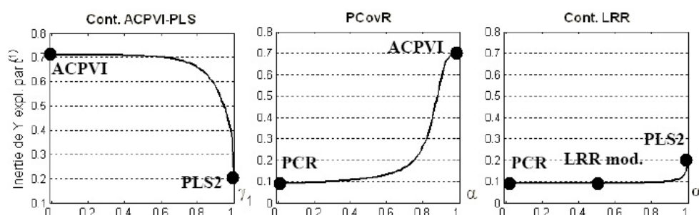
FIG. 5.4 – Comparaison des inerties de Y expliquées par la composante t^{(1)} en fonction du paramètre du continuum ( \alpha ou \gamma_1 ) pour les méthodes : continuum LRR, principal covariate regression et continuum ACPVI-PLS. Les cas particuliers de ces continuums sont aussi indiqués.
