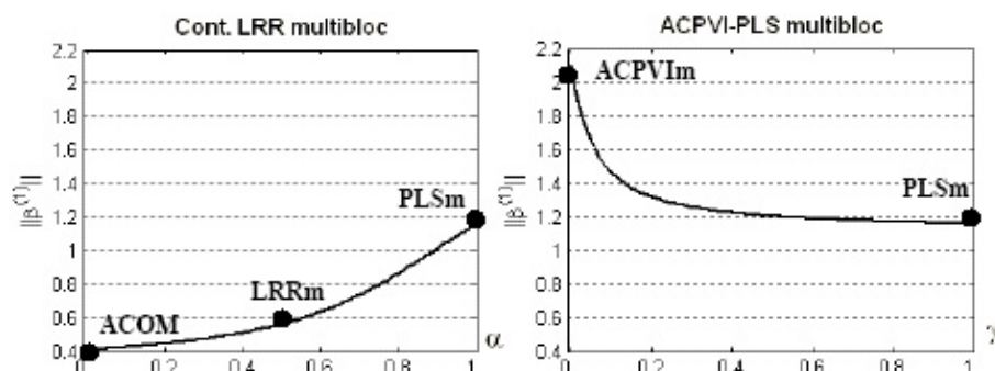
FIG. 8.9 – Comparaison de la norme du vecteur de coefficients \beta^{(1)} pour les continnum LRR multibloc et ACPVI-PLS multibloc. Les cas particuliers de ces continnum sont aussi indiqués.
