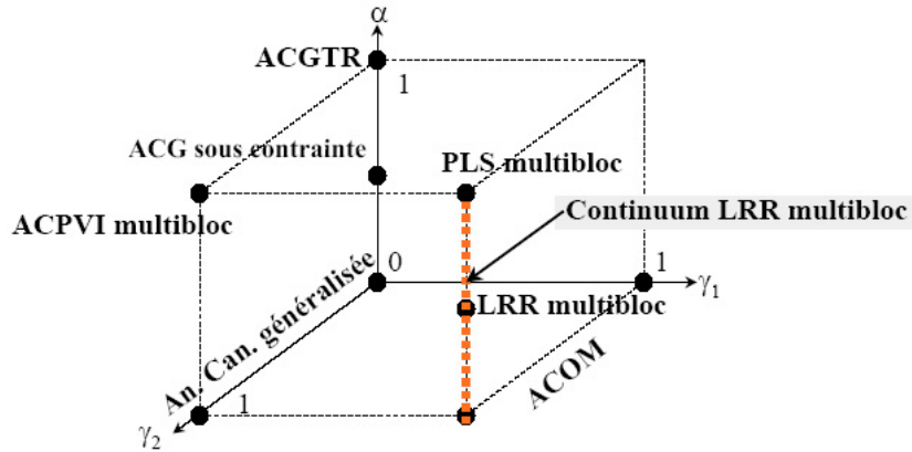
FIG. 7.2 – Illustration du domaine exploré par le continuum LRR multibloc.
