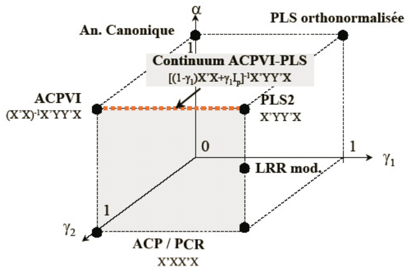
FIG. 4.6 – Illustration du domaine exploré par le continuum ACPVI – PLS.
