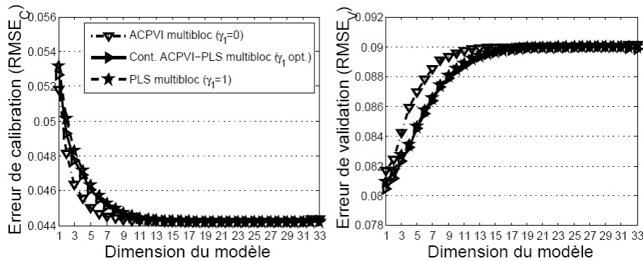
FIG. 8.12 – Erreur moyenne de calibration ( RMSE_C ) et de validation ( RMSE_V ) pour le continuum ACPVI-PLS multibloc ( \gamma_1 optimum) et ses cas particuliers : ACPVI multibloc ( \gamma_1 = 0 ) et PLS multibloc ( \gamma_1 = 1 ).
