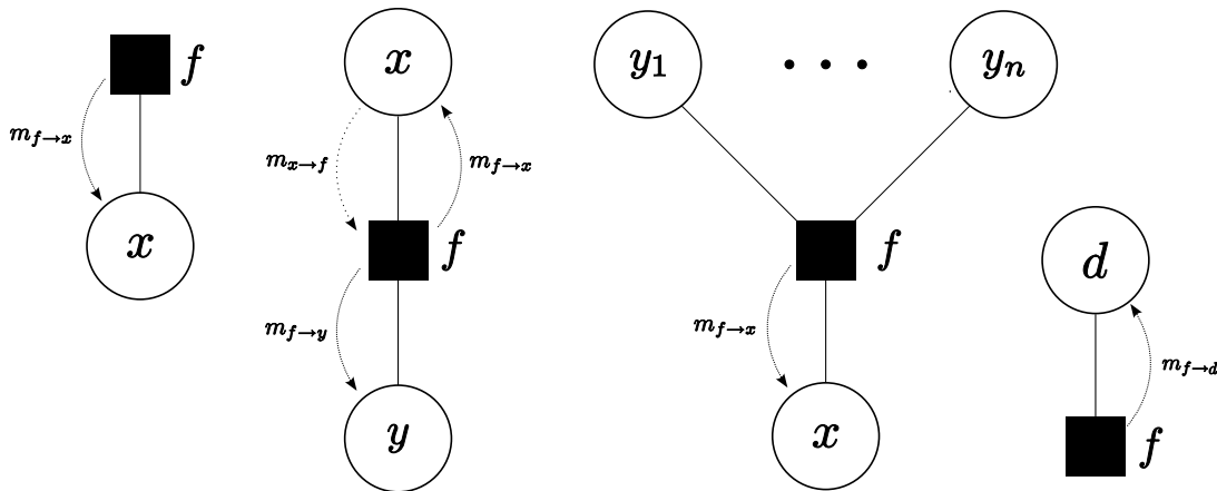
FIG. 3.9 – Les quatre types de facteurs du modèle et leurs messages. De gauche à droite : facteur d’a priori, de performance, de combinaison linéaire et de résultat. Les messages de variable à facteur ne sont pas explicites. Seul le facteur de résultat nécessite une approximation de type EP (projection).
