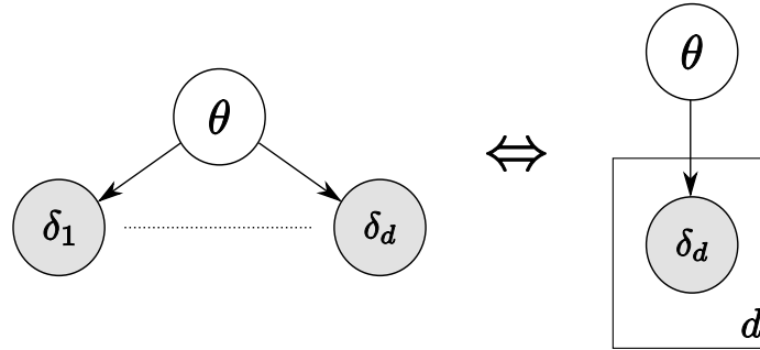
FIG. 1.2 – Réseau bayésien représentant la décomposition de la jointe pour le modèle d’une pièce. Il est courant de griser les variables observées. À droite la représentation équivalente avec une assiette ( plate ) est possible car toutes les distributions conditionnelles (sur les arcs) sont identiques. Ce modèle en étoile est appelé modèle de dépendance bayésien naïf , il est souvent employé pour ses propriétés calculatoires.
