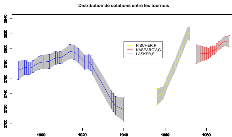
FIG. 3.18 – Interpolation des estimations des cotations pour Kasparov, Fischer et Lasker ( \mu \pm \sigma ).
