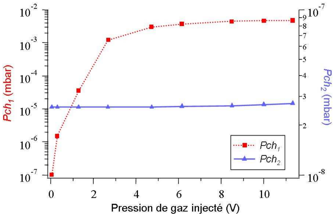
Figure IV-26- Evolution de la pression dans la première et la deuxième chambre, respectivement P_{ch1} et P_{ch2} , en fonction de la pression de gaz injecté. La correspondance volt-pression est donnée en Annexe 2.
