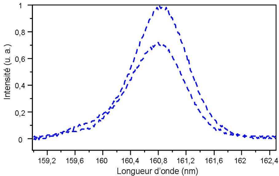
Figure VII-37- Spectres des rayonnements LELs en mode non-injecté (a, moyenné sur 10 impulsions, g_1=3,549 mm) et harmonique (b, mono-impulsion, P_g=9,5 V, 1 minute entre les deux impulsions, paramètres laser : E_{impulsion}=19 mJ et \Phi=21 mm).
