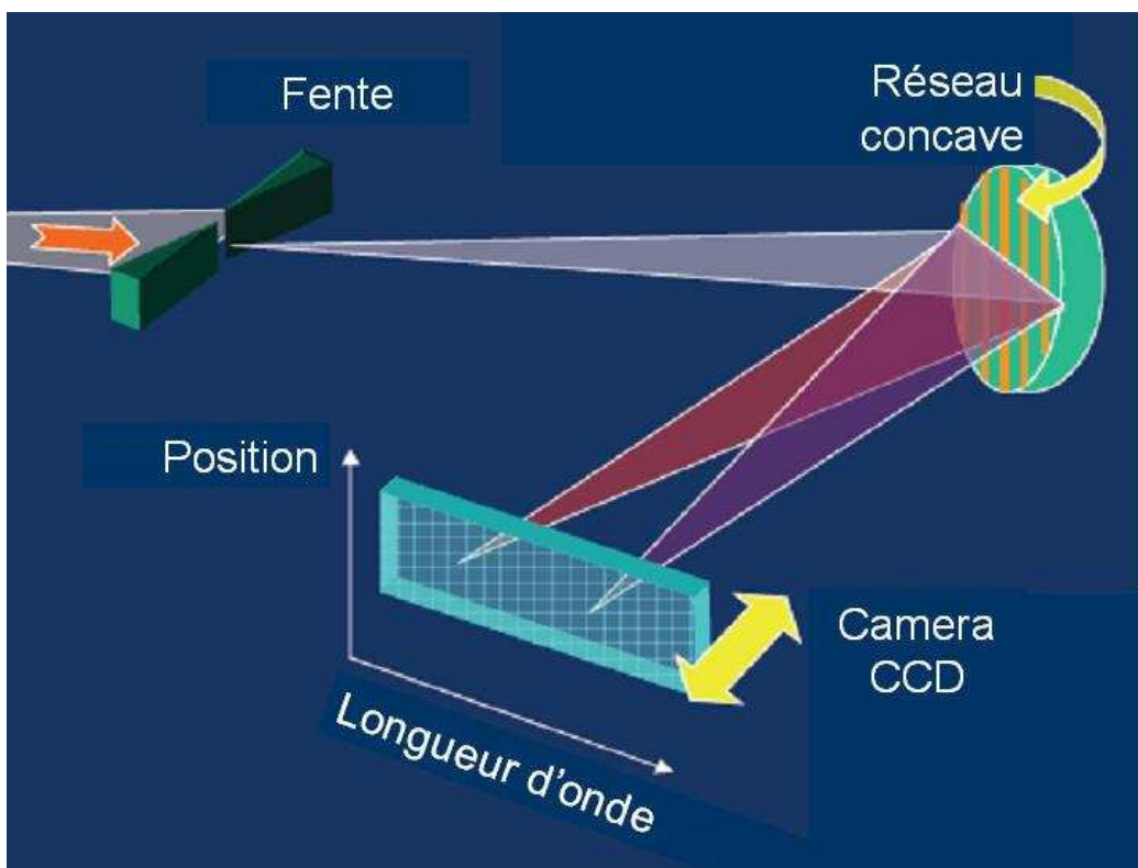
Figure IV-27- Spectromètre [170] à réseau laminaire (Shimatsu Corp. revêtement Or, de densité linéaire D_{lin}=2400 lignes/mm, et de rayon de courbure R=922 mm) de résolution spectrale ( \Delta\lambda/\lambda ) inférieure à 0,1%. Le spectromètre a été calibré, à 0,033 nm près, sur la raie 1 d'une lampe à Hélium. La caméra CCD est de la marque Princeton Instruments, modèle PI* SX 400, 1340x400 pixels de 20 \mu\text{m} de côté.
