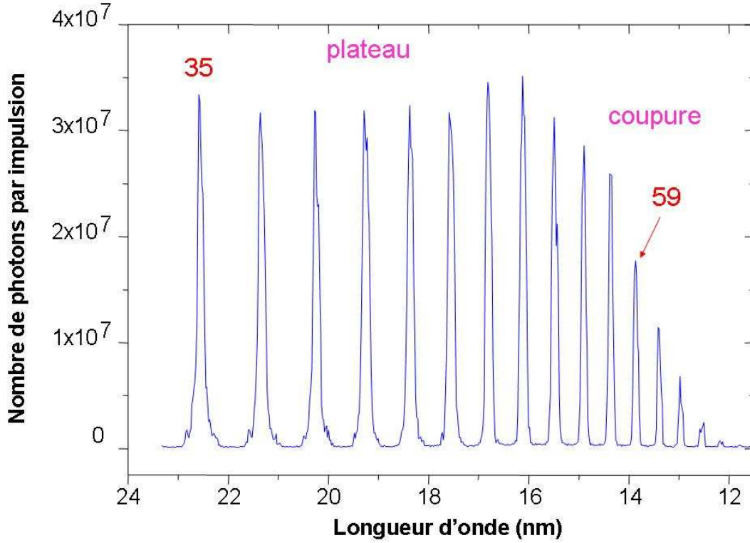
Figure III-5- Spectre classique de génération d'harmoniques d'ordre élevé, obtenu dans le Néon. Les chiffres 35 et 59 indiquent l'ordre de l'harmonique considérée.
