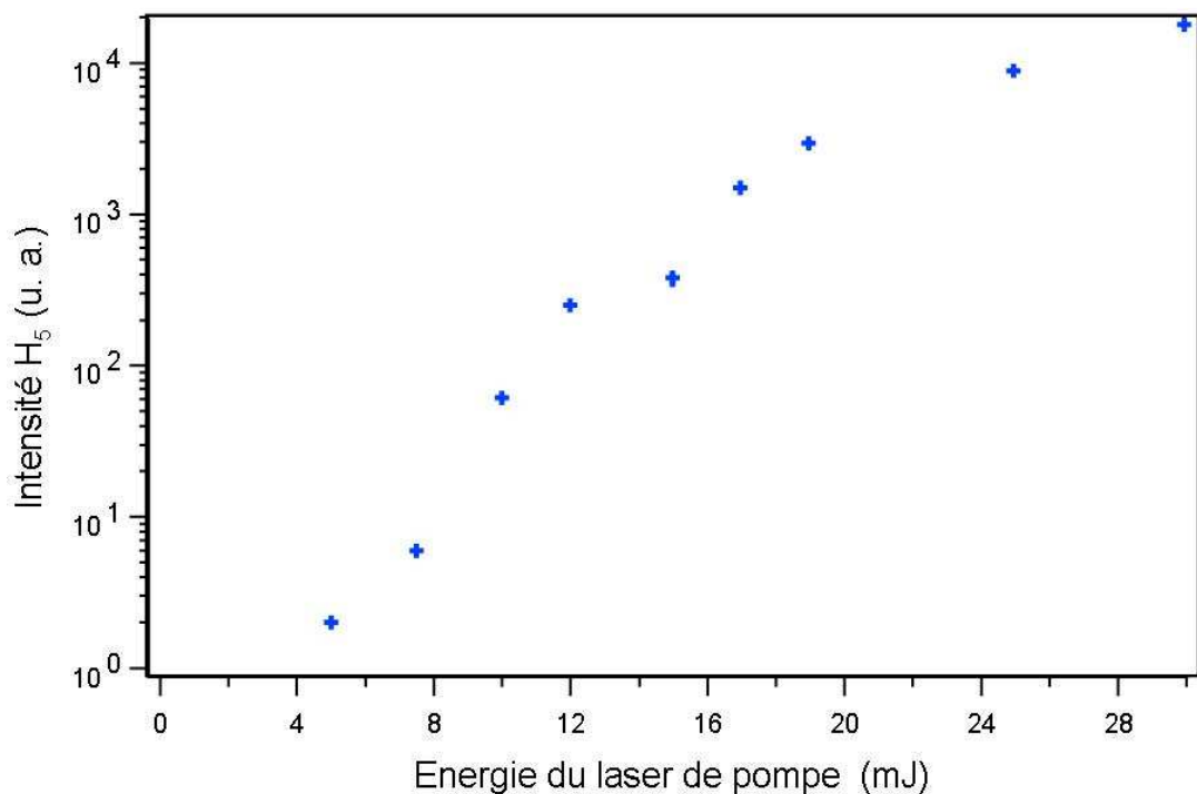
Figure V-15- Intensité de la 5 ème harmonique en fonction de l'énergie par impulsion du laser générateur. Temps d'exposition : 1 s. P_g=11 V. Paramètre laser : \Phi=21 mm. a) Echelle linéaire. b) Echelle logarithmique. Barre d'erreur de chaque mesure : \pm 23 % environ.
