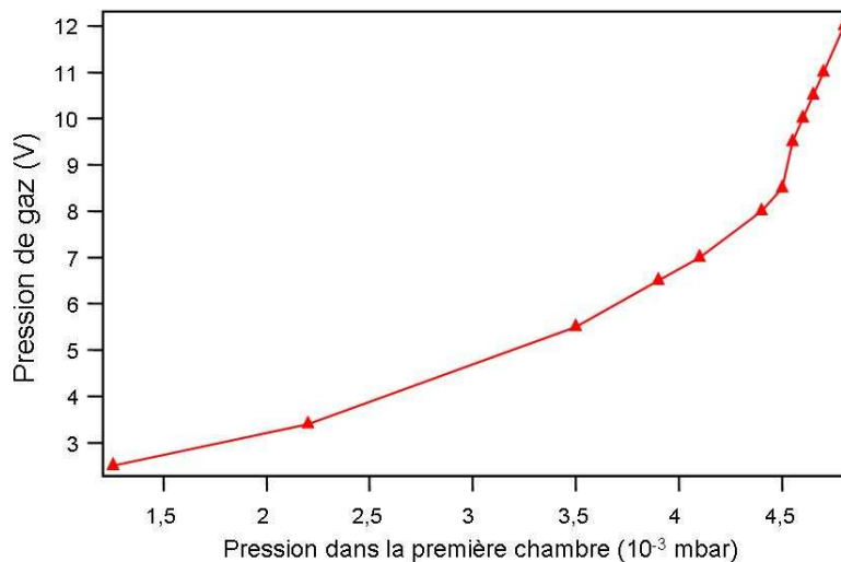
Figure VII-50- Equivalence de pression entre la valeur de pression en Volt lue sur le détecteur de gaz ( P_g ) et la pression du vide dans la première enceinte en Pascal ( P_{ch1} ).
