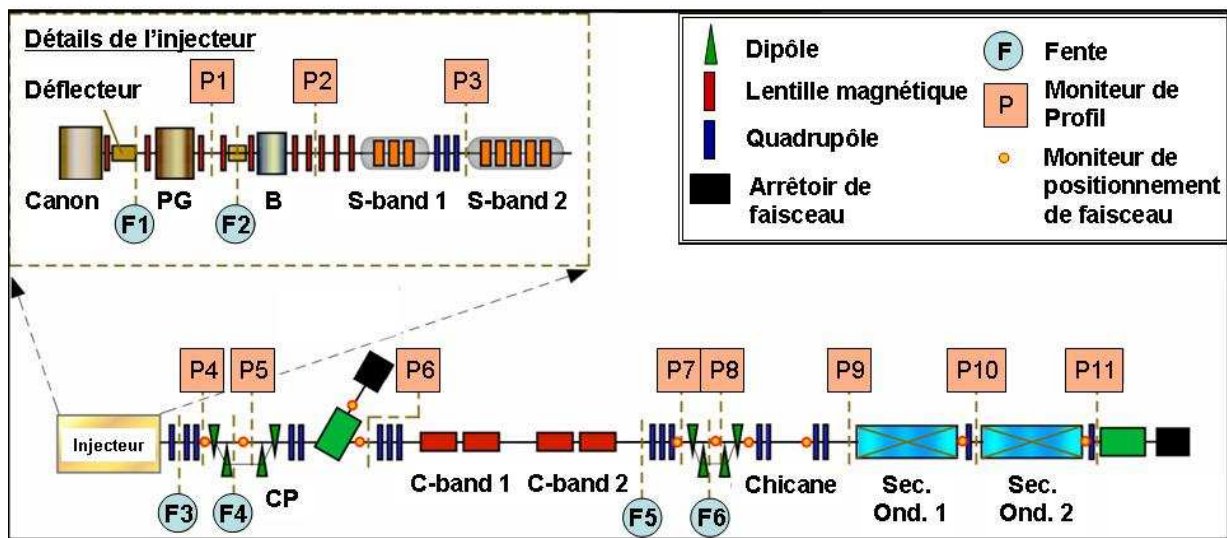
Figure IV-3- Dessin schématique du LEL du Prototype de l'accélérateur SCSS [169]. PG est utilisé pour Pré-Groupeur, B pour Booster, CP pour compression de paquets. S-band (2856 MHz) ainsi que C-band (5712 MHz) correspondent au type de section accélératrice.
