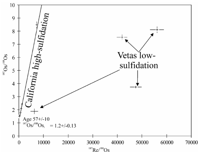
Figure 58. Diagramme isochrone pour les échantillons du gisement épithermal acide (high-sulfidation) de California. Les échantillons de l'épithermal neutre (low-sulfidation) de Vetas présentent des valeurs très dispersées et ne s'alignent pas sur l'isochrone du gisement de California (Mathur et al., 2003).
