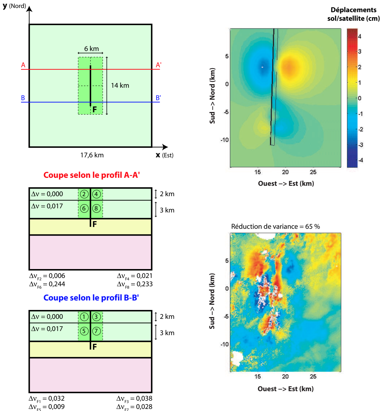
FIG. 5.8 Résultat de l'inversion avec une configuration poro-élastique à deux couches et avec une zone de faille en quatre quadrants (dix paramètres libres). (Gauche) Résultats de l'inversion et schéma de la configuration poro-élastique utilisée (voir la légende de la figure 5.4). (En haut à droite) Déplacements modélisés avec cette configuration. (En bas à droite) Interférogramme résiduel entre les déplacements observés et modélisés (voir la légende de la figure 5.1). La valeur de la réduction de variance indiquée en haut de l'interférogramme est la plus importante (Figures 5.5, 5.6 et 5.7), mais l'amélioration apportée est minime quand on la compare à la complexité de la configuration. Les déplacements modélisés sont également présentés dans la figure 5.3 (configuration 5).
