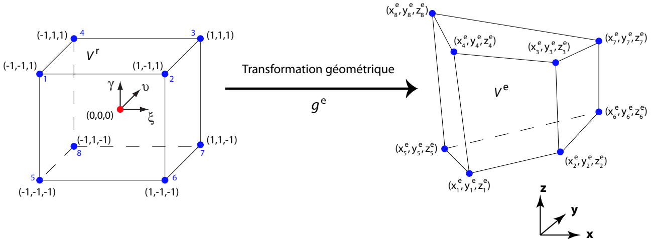
FIG. 3.9 Schéma illustrant la transformation g^e qui permet de passer de l'élément de référence de volume V^r à un élément e de volume V^e . Dans TECTON, les éléments tridimensionnels sont des hexaèdres (à droite) et l'élément de référence est un cube (à gauche) défini dans le repère (\xi, v, \gamma) d'origine O par n = 8 nœuds. Après la transformation g^e , qui s'écrit à partir des fonctions de transformation géométrique \tilde{\mathbf{N}} , ces nœuds se retrouvent dans le repère d'étude (x, y, z) avec les coordonnées (x_n^e, y_n^e, z_n^e) . Les formules à droite donnent l'expression des polynômes de transformation géométrique utilisés dans TECTON qui composent la matrice \tilde{\mathbf{N}} .
