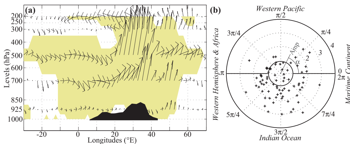
Fig. 5.2 : (a) Coupe verticale de l'atmosphère le long de l'équateur (2.5°N - 2.5°S) durant les événements pluviométriques extrêmes sur les Hautes Terres. Les anomalies significatives apparaissent en couleur (test t^2 de Hotelling, 95%). La topographie de l'Afrique équatoriale telle qu'elle apparaît dans les grilles NCEP est montrée. (b) Distribution des événements pluviométriques extrêmes (+) dans le cycle MJO (défini selon les indices RMM1 , RMM2 ). La localisation estimée de la convection active est indiquée. Le cercle intérieur délimite les jours de faible activité MJO (Amp < 0.9).
