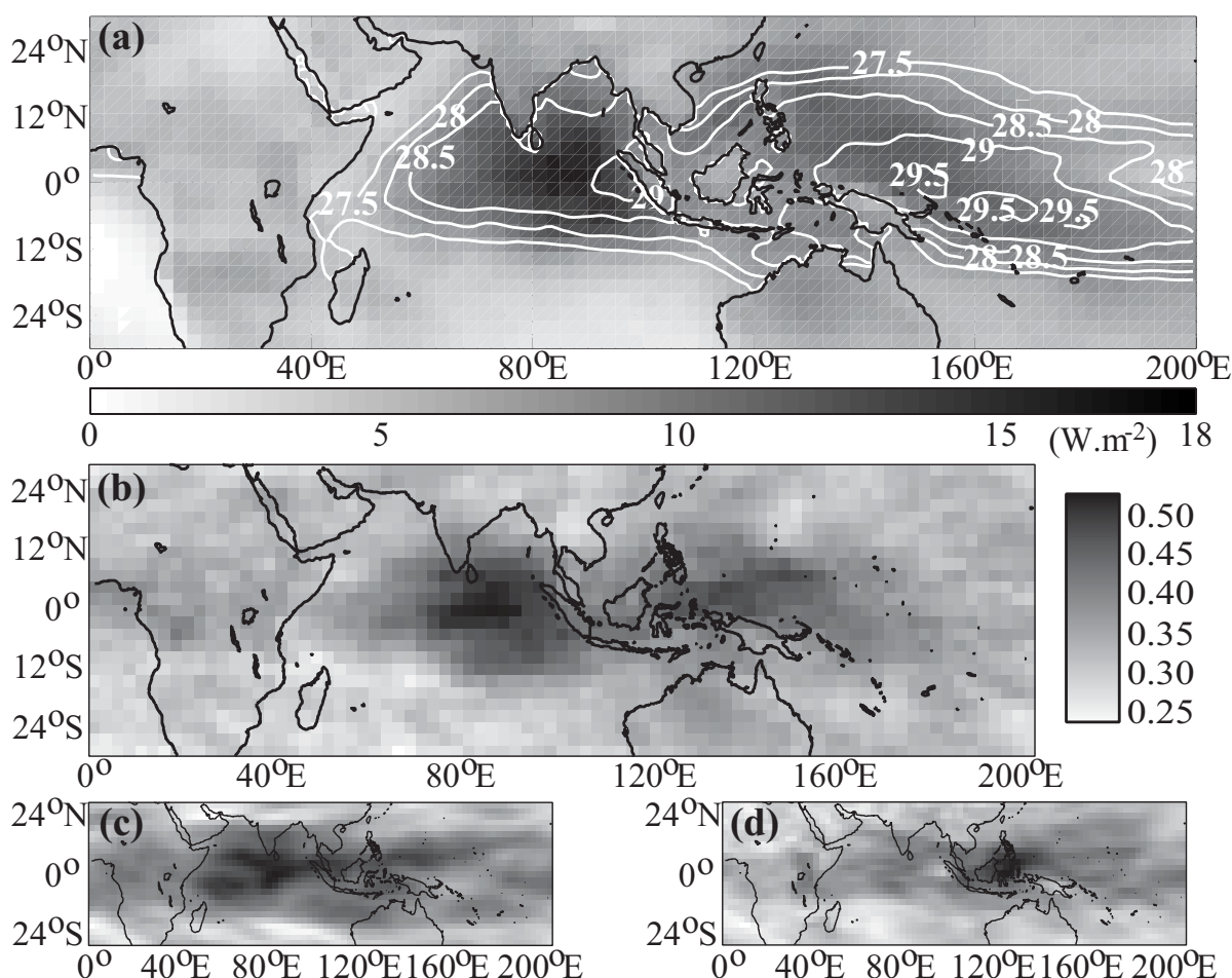
Fig. 2.25 : (a) Grisés : amplitude du mode moyen de la Figure 2.24 dans l'OLR ( \text{W.m}^{-2} ). Contours : températures de surface de la mer moyennées sur la période 1979-2005. La première isotherme est à 27.5^{\circ}\text{C} , puis l'équidistante entre deux isothermes est de 0.5^{\circ}\text{C} . (b) Cohérence de l'OLR sur la période 1979-2005 : part de la variance totale de l'OLR dans la fenêtre mobile de 120 jours expliquée en moyenne par les modes locaux. Une cohérence de 0.4 s'interprète comme 40% de variance commune en moyenne entre l'OLR et les modes locaux extraits sur la période considérée. (c) Comme (b) mais pour U200. (d) Comme (b) mais pour U850.
