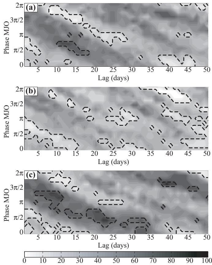
Fig. 5.44 : Comme pour la Figure 5.40 mais pour la probabilité de dépasser la valeur du cycle annuel pendant les années La Niña (%).
