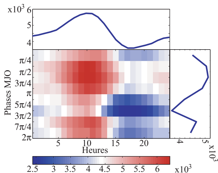
Fig. 5.35 : Comme pour la Figure 5.34, mais pour les Hautes Terres Orientales ( 3^{\circ}\text{S} - 0^{\circ} , 34.5^{\circ}\text{E} - 35.5^{\circ}\text{E} ).
