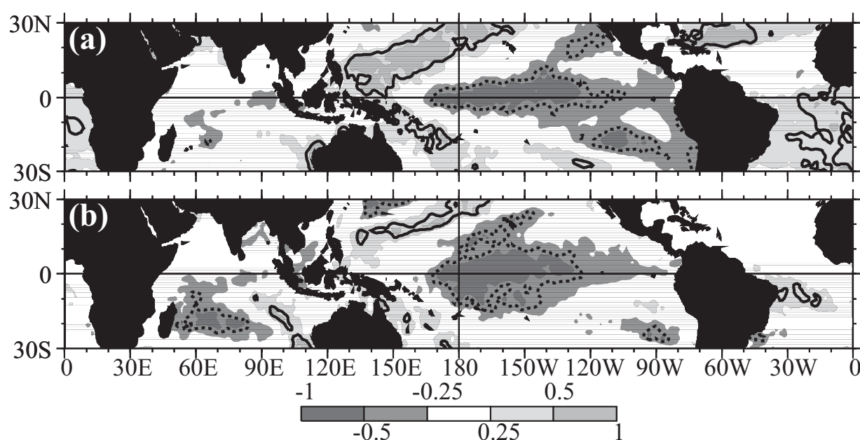
Fig. 3.4 : Corrélations entre la période moyenne de la MJO moyennée sur les 3 mois de MAM (a) et OND (b), et les TSM moyennes durant les mêmes saisons. La valeur des grisés est donnée par la légende. Les contours solides (resp. pointillés) indiquent les corrélations positives (resp. négatives) qui dépassent le seuil de significativité de 95%.
