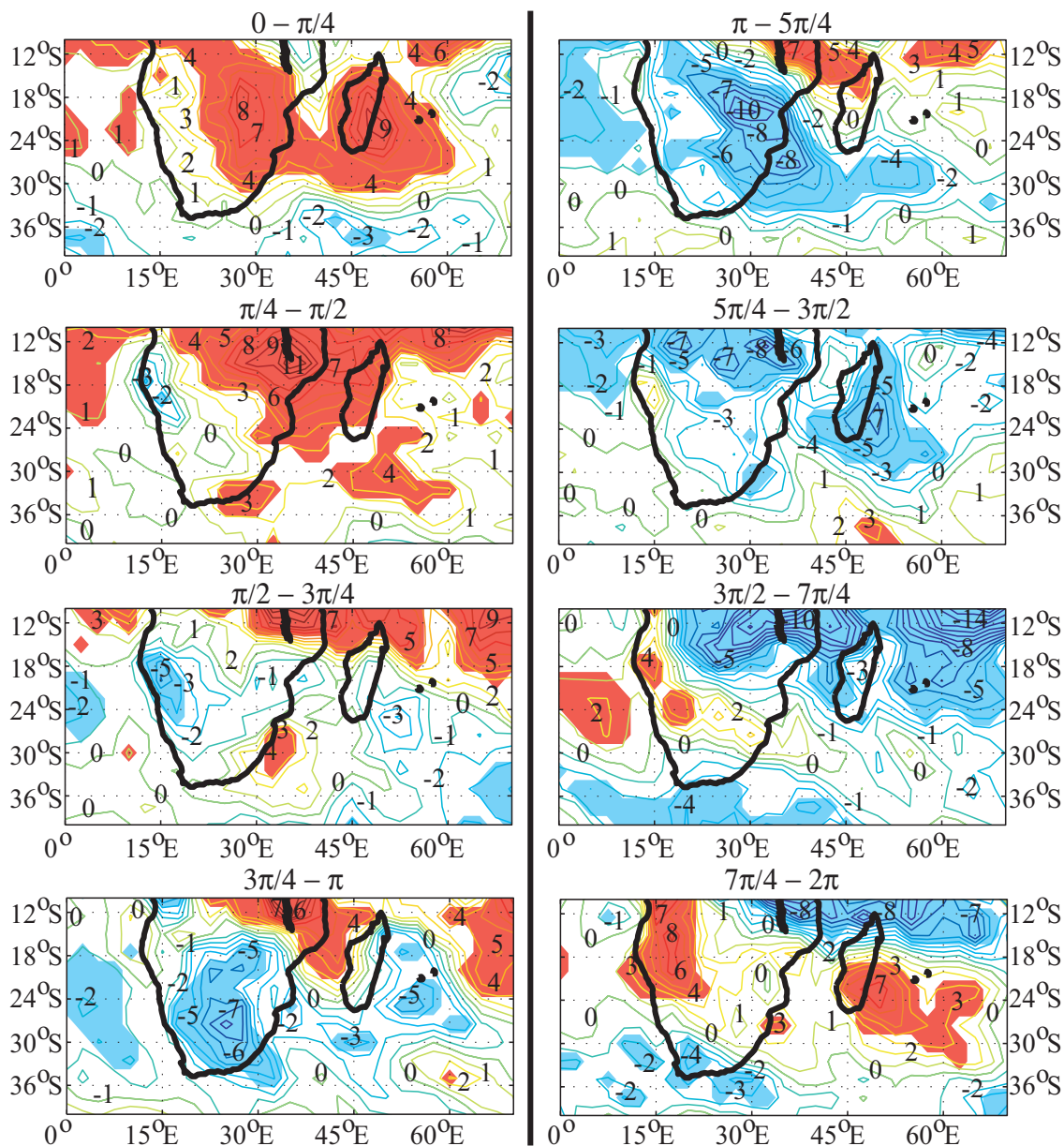
Fig. 4.14 : Cartes composites des anomalies d'OLR ( \text{W.m}^{-2} ), calculées après retrait du cycle annuel, sur l'Afrique Australe durant la période ONDJFMA 1974-1999. L'équidistance des isolignes est de 1 \text{ W.m}^{-2} . Les aplats bleus (resp. rouges) indiquent les anomalies négatives (resp. positives) qui sont significatives au seuil de 95% selon un t-test.
