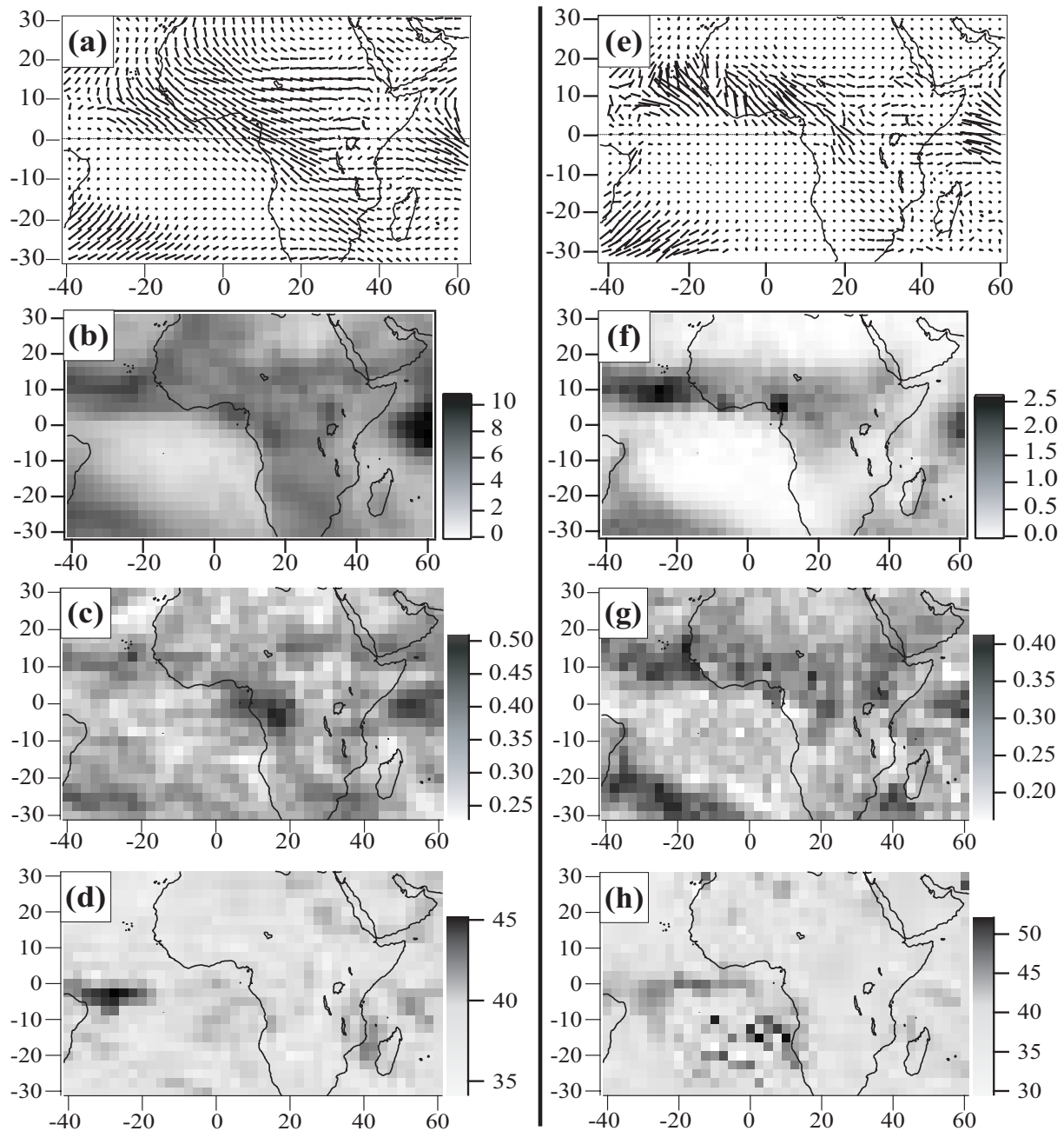
Fig. 4.40 : Mode moyen sur l'Afrique, période JAS 1979-2001. (a) Mode propagatif moyen dans l'OLR. (b) Amplitude moyenne de l'OLR ( \text{W.m}^{-2} ). (c) Cohérence de l'OLR. (d) Période moyenne des modes locaux pour chaque point de grille. (e-h) Comme (a-d) mais pour CMAP ( \text{mm.jour}^{-1} ).
