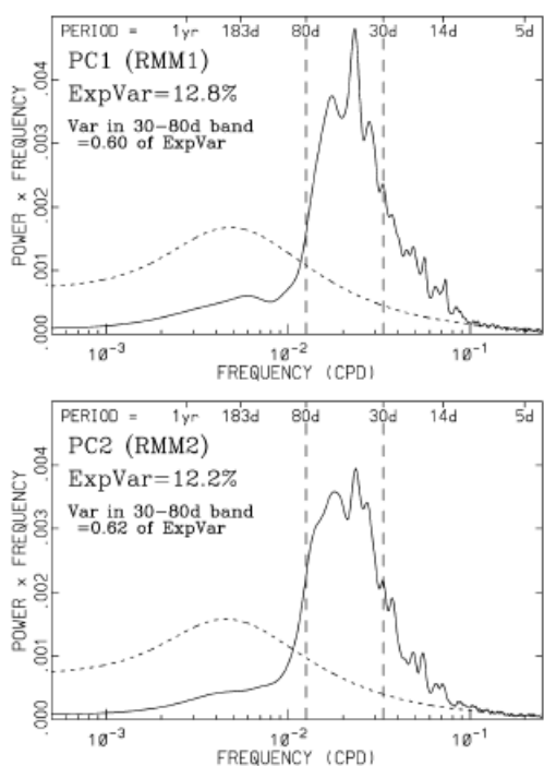
Fig. 2.5 : Analyse en spectre de puissance de RMM1 et RMM2, calculée sur la période 1974-2003. La surface sous les courbes de puissance est égale à la variance, pour chaque fréquence du spectre. La superficie totale sous chaque courbe de puissance égale la part de variance totale expliquée par la CP correspondante. La fraction de variance expliquée dans la gamme de fréquence 30-80 jours est indiquée sur les figures. Les courbes pointillées indiquent le seuil de significativité à 95% calculé selon un procédé de bruit rouge qui prend en compte l'autocorrélation de rang 1 des séries.
