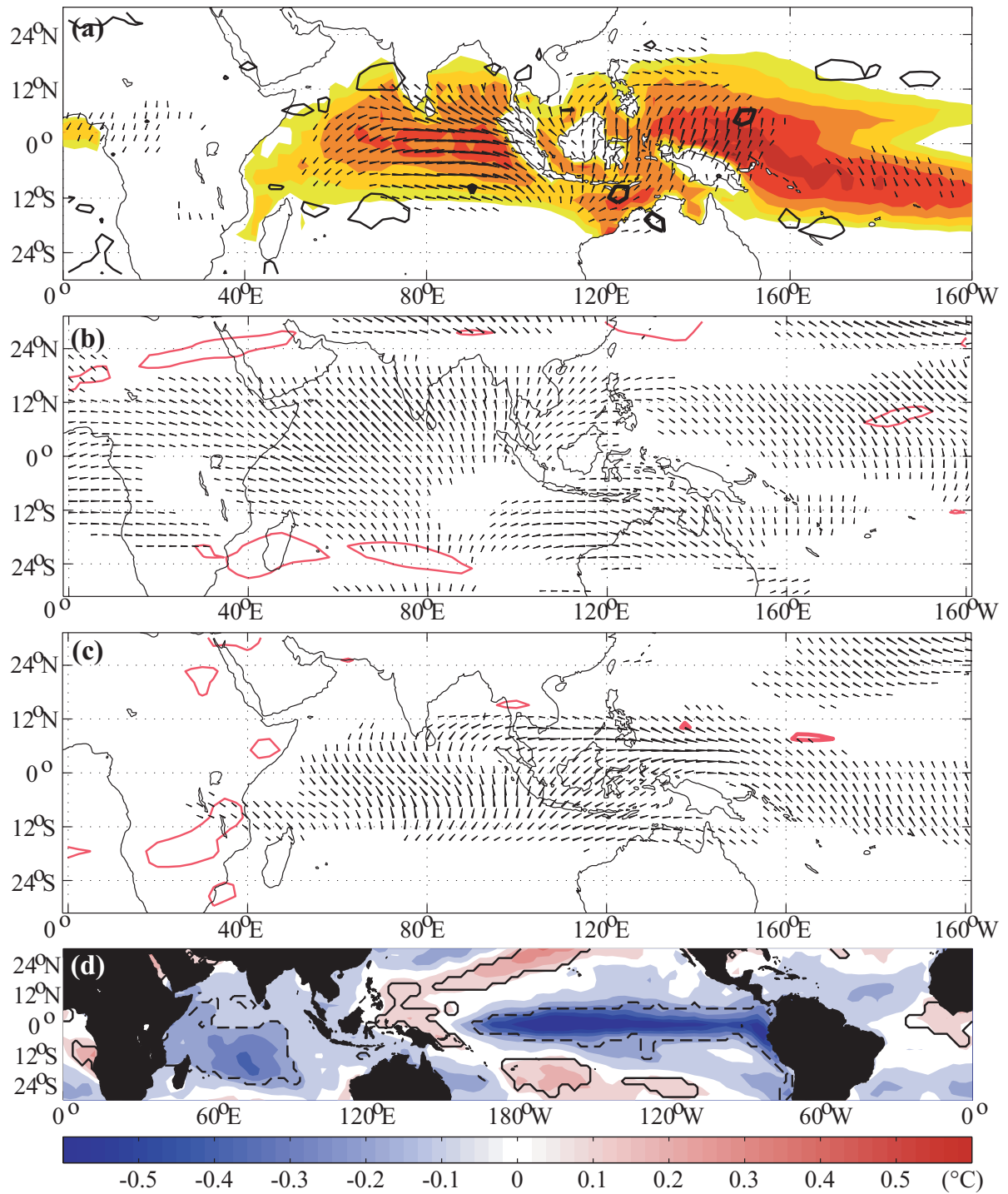
Fig. 3.21 : Comme pour la Figure 3.14 mais pour le type 8 (23 modes locaux).
