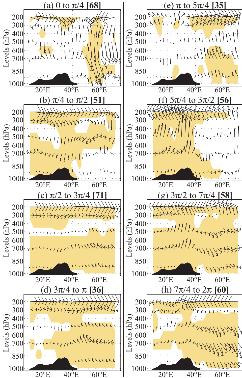
Fig. 4.9 : Coupes verticales à l'équateur ( 2.5^{\circ}\text{N} - 2.5^{\circ}\text{S} ) des anomalies verticales ( \omega , -1 \times \text{Pa.s}^{-1} ) et zonales ( U , \text{m.s}^{-1} ) du vent, après retrait du cycle annuel, pour chaque phase MJO. Les aplats indiquent les anomalies significatives au seuil de 95% selon un test t^2 de Hotelling. Les profils noirs correspondent à la topographie de l'Afrique Equatoriale telle qu'elle apparaît dans les mailles du modèle NCEP. Le nombre de pentades incluses dans chaque huitième de phase est indiqué sur la figure (leur total correspondant aux 435 pentades d'amplitude supérieure à 0.9 sur la période MAM+OND 1979-1995).
