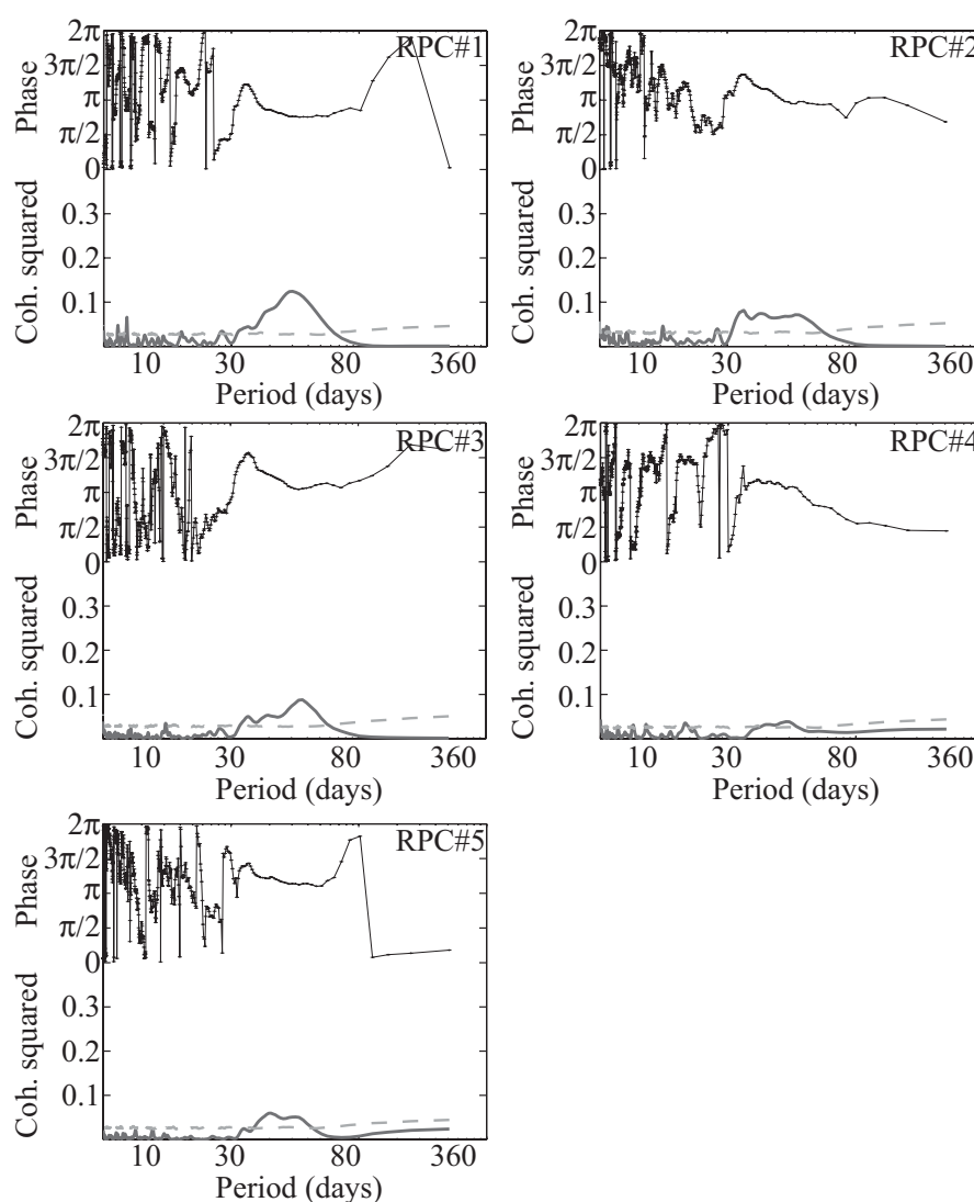
Fig. 4.20 : Analyses crossspectrales des indices régionaux normalisés des pluies sud-africaines et de l'indice RMM1 de Wheeler & Hendon (2004). Toutes les analyses sont appliquées sur la période ONDJFMA 1974-1999, les autres mois ont été complétés 0. Significativité testée et représentée comme pour la Figure 4.19. Ligne noire continue avec signes + : relation de phase (en radians).
