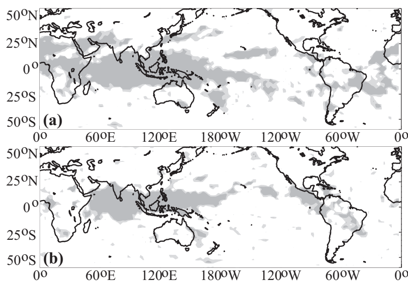
Fig. 2.12 : (a) Analyse de variance entre les phases MJO (identiques à la Figure 2.9) et les anomalies d'OLR après retrait du cycle annuel, calculée sur tous les jours d'amplitude MJO modérée à forte ( A \geq 0.9 ) de la période novembre-avril 1979-2005. Les aires apparaissant en gris clair (resp. gris foncé) dénotent une discrimination des valeurs quotidiennes d'OLR par les phases MJO significative au seuil de 95% (resp. 99%) selon le test de Fisher-Snedecor. (b) Comme pour (a) mais pour la saison mai-octobre.
