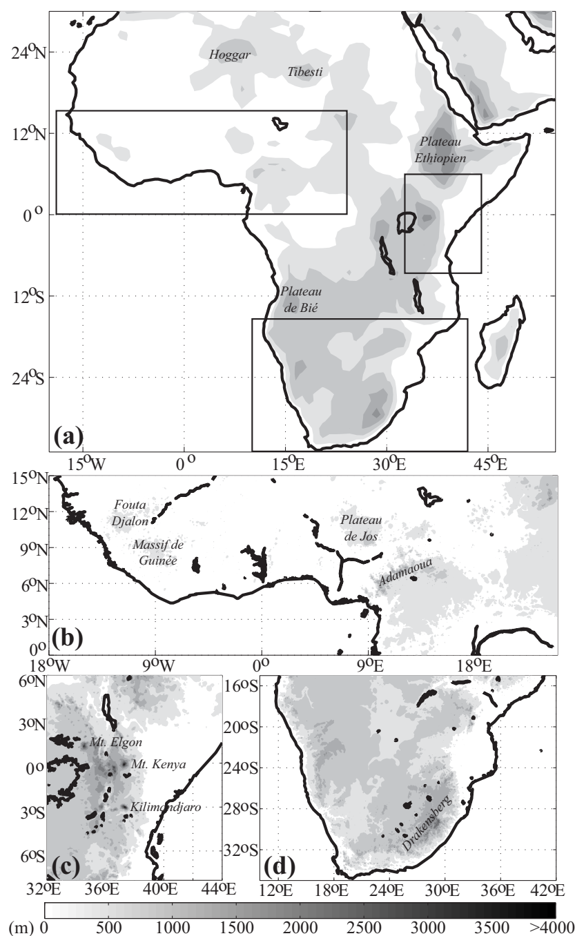
Fig. 1.5 : (a) Topographie de l'Afrique (modèle numérique de terrain de 1° x 1°). (b) Topographie de l'Afrique de l'Ouest (MNT de 5' x 5'). (c) Comme (b) mais pour l'Afrique de l'Est. (d) Comme (b) mais pour l'Afrique Australe. La valeur des grisés est donnée par la légende.
