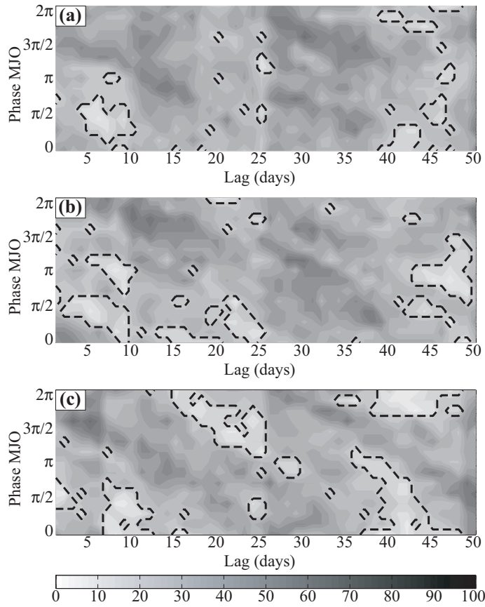
Fig. 5.43 : Comme pour la Figure 5.40 mais pour la probabilité de dépasser la valeur du cycle annuel (%).
