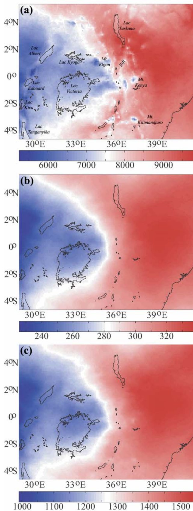
Fig. 5.27 : Champs moyens (radiance, W.m -2 .sr -1 ) des canaux MSG IR10.8 (a), WV6.2 (b) et WV7.3 (c), MAM 2005.
