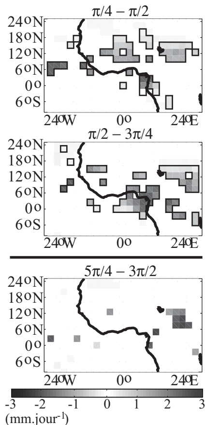
Fig. 4.32 : Anomalies de pluies (mm.jour -1 ) selon les estimations CMAP pour les phases MJO \pi/4-3\pi/4 et 5\pi/4-3\pi/2 , période JAS 1979-2005. La valeur des grisés est donnée par la légende. Les points de grille qui apparaissent en blanc ne sont pas significatifs selon un test de Student au seuil de 95%. Les anomalies négatives ont été entourées par des contours noirs.
