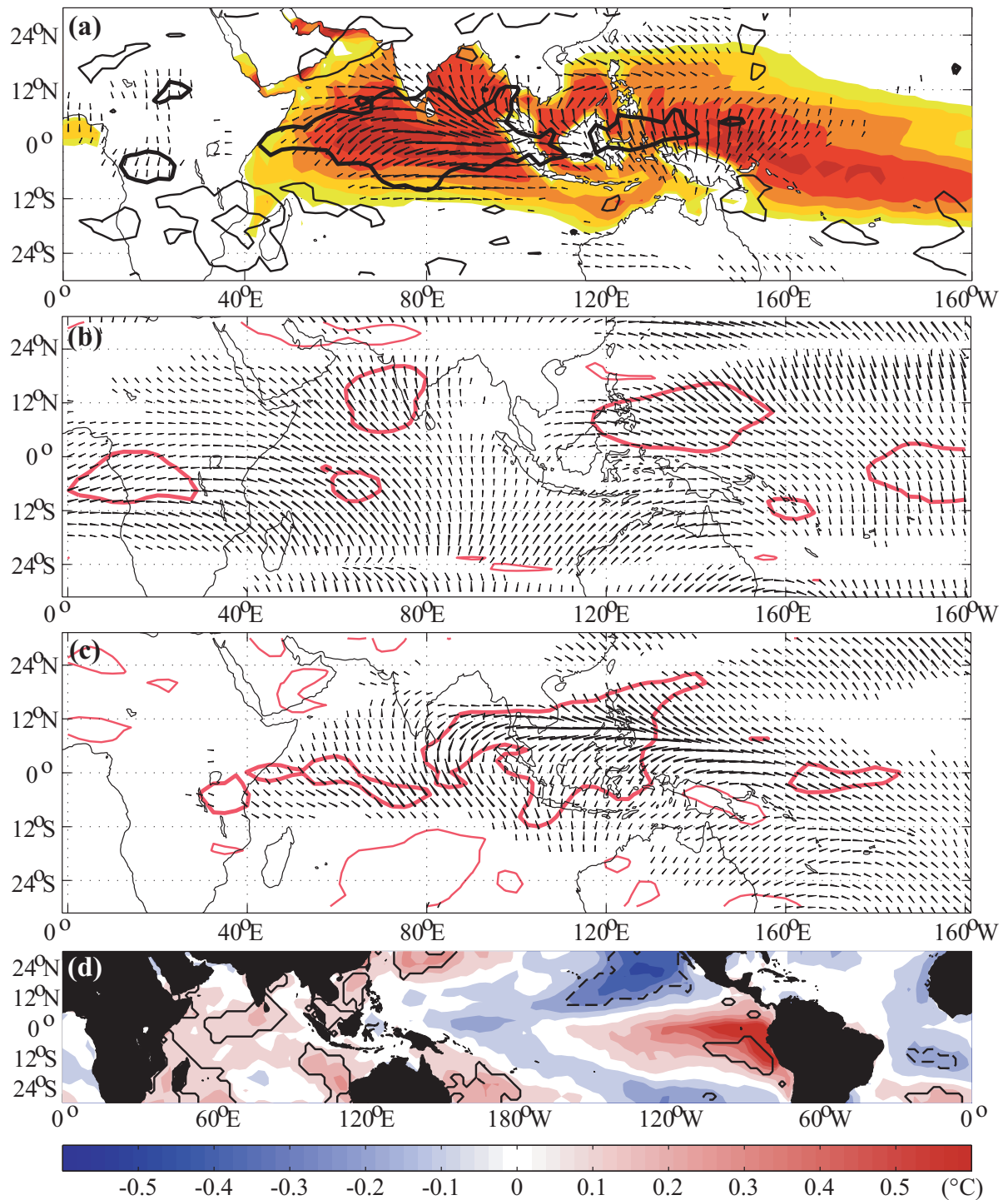
Fig. 3.16 : Comme pour la Figure 3.14 mais pour le type 3 (15 modes locaux).
