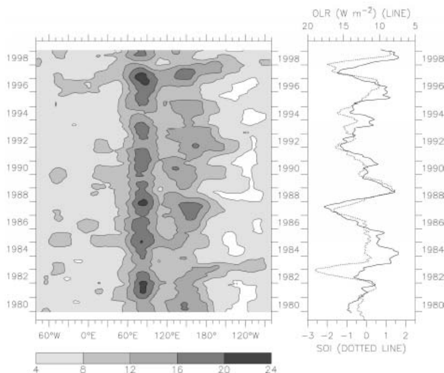
Fig. 2.3 : (Gauche) Amplitude de la racine carrée de l'OLR élevé au carré ( (W.m^{-2})^2 ) puis filtré par une moyenne mobile de un an. Les valeurs ont été calculées le long de l'équateur ( 5^{\circ}N - 5^{\circ}S ) sur la période 1980-1998. (Droite) Ligne continue : valeur moyenne de l'amplitude de l'OLR moyenné spatialement sur le centre du Pacifique ( 5^{\circ}N - 5^{\circ}S , 150^{\circ}E - 180^{\circ}E ). Ligne pointillée : valeur correspondante de l'indice SOI.
