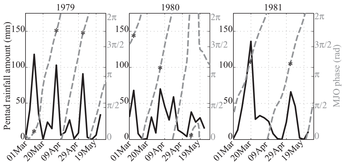
Fig. 4.4 : Cumuls pluviométriques pentadaires à Kisumu (Kenya, indice W : ligne continue, axe de gauche) et phase MJO correspondante selon les indices MJO (RMM1, RMM2) (ligne pointillée, axe de droite) pour les Long Rains de 1979, 1980 et 1981. Les astérisques dénotent les phases MJO du pic de pluie.
