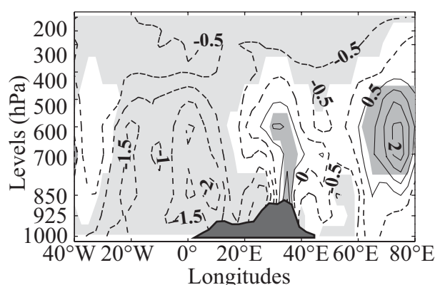
Fig. 5.10 : Différence d'énergie statique humide le long de l'équateur ( 2.5^{\circ}\text{N} - 2.5^{\circ}\text{S} ) entre les années à " r^2 élevé" et les années à " r^2 faible" (définies dans la Table 5.5), par rapport à l'indice W, et pendant la phase MJO 5\pi/4-7\pi/4 . Les différences significatives positives (resp. négatives) selon un test de Student au seuil de 95% apparaissent en gris foncé (resp. gris clair).
