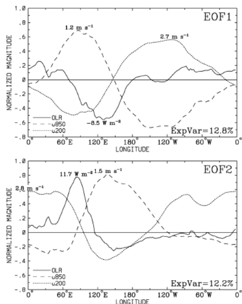
Fig. 2.4 : Structures spatiales des deux premières CP des champs combinés U850, U200 et OLR, tels que décrits dans la section 2.2.1.
