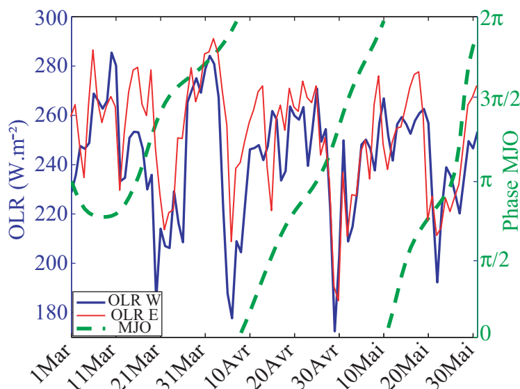
Fig. 5.19 : Séries temporelles d'OLR ( \text{W.m}^{-2} ), MAM 2005, moyennées sur les points de grille des indices régionaux E et W de la Figure 4.3 (axe des ordonnées de gauche). La phase MJO correspondante apparaît en pointillés (axe des ordonnées de droite).
