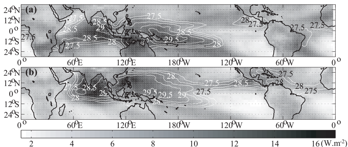
Fig. 2.2 : (a) Grisé : écart-type du champ OLR filtré en bande passante 30-60 jours ( \text{W.m}^{-2} , cf. légende pour les niveaux de gris), période novembre-avril 1979-2005. Contours : TSM moyennes au-dessus du seuil de 27.5°C durant la même période. L'écart entre 2 isothermes successives est de 0.5°C. (b) Comme (a) mais pour la saison mai-octobre.
