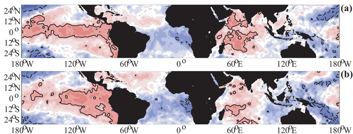
Fig. 5.9 : (a) Comme pour la Figure 5.8a mais avec les TSM de juin. (b) Comme pour la Figure 5.8a mais avec les TSM de juillet.
