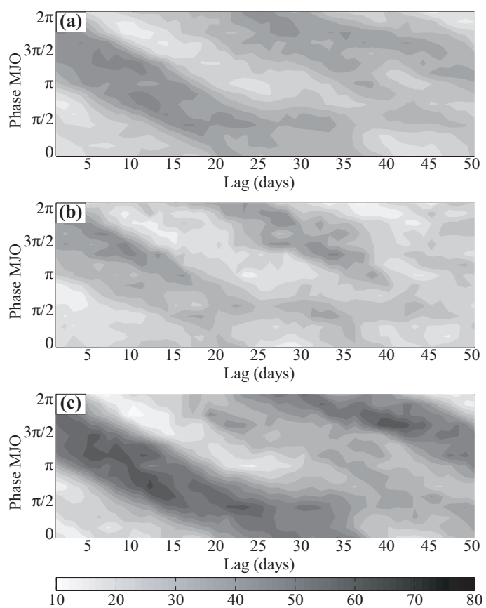
Fig. 5.47 : Comme pour la Figure 5.40 mais pour le pourcentage de stations dépassant la valeur du cycle annuel (%) pendant les années La Niña.
