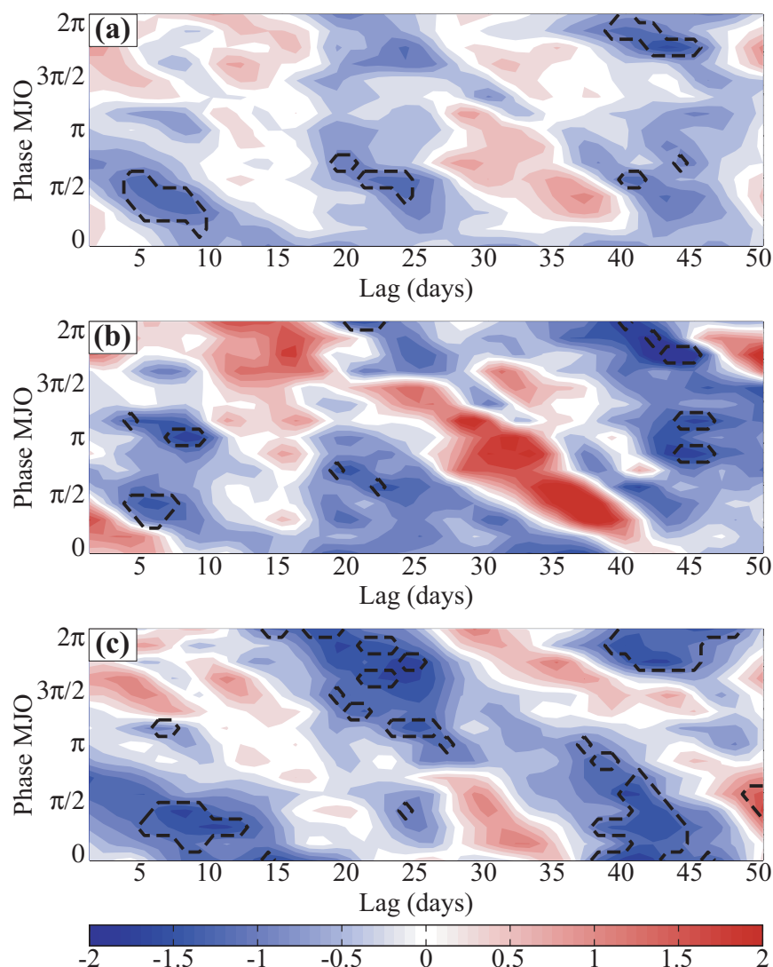
Fig. 5.40 : Diagramme croisant phase MJO extraite et anomalies désaisonnalisées de précipitations ( \text{mm.jour}^{-1} ) filtrées en passe-bas 10 jours, en fonction du lag, pour les années El Niño et (a) pour la région d'Afrique de l'Est, (b) pour l'indice E, (c) pour l'indice W. Les anomalies significativement différentes de la valeur du cycle annuel (t-test, 95%) ont été entourées d'une ligne noire pointillée.
