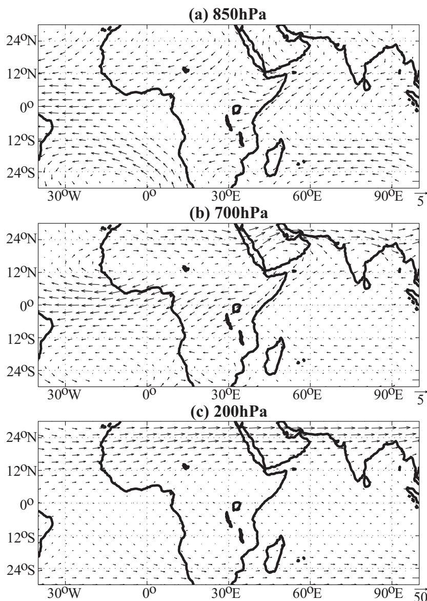
Fig. 1.8 : Circulation atmosphérique annuelle moyenne ( \text{m.s}^{-1} ) selon les réanalyses NCEP2 sur la période novembre - avril 1979-2005, (a) à 850hPa, (b) à 700hPa, (c) à 200hPa.
