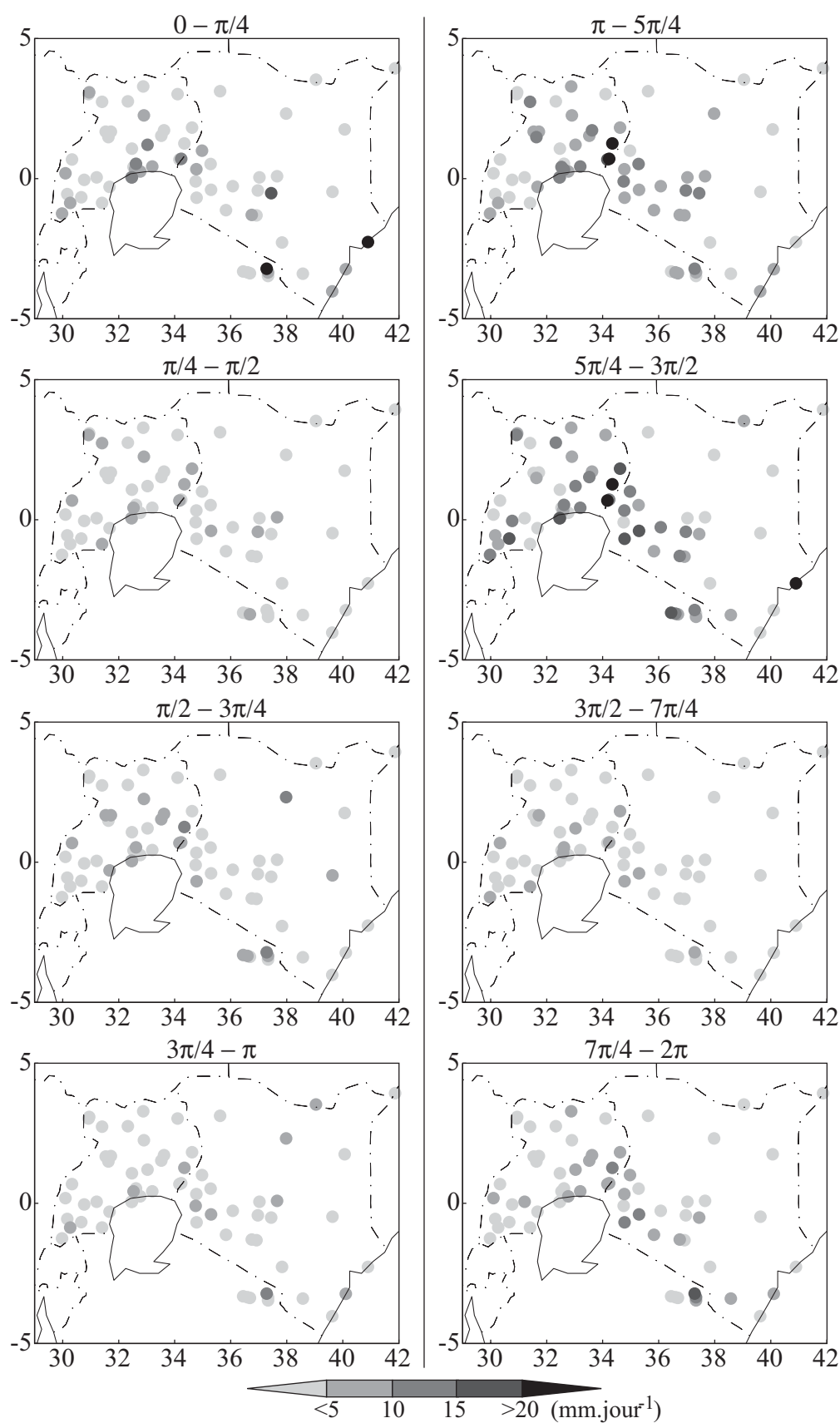
Fig. 5.21 : Analyse composite des relevés pluviométriques d'Afrique de l'Est au cours du cycle MJO ( \text{mm.jour}^{-1} ). L'échelle des grisés donne la valeur moyenne des cumuls journaliers, pour chaque pluviomètre et pour chaque phase MJO.
