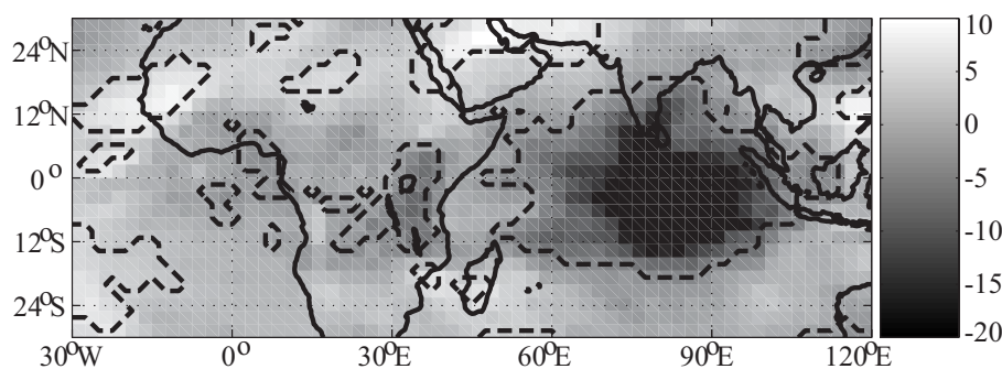
Fig. 4.11 : Anomalies moyennes d'OLR, après retrait du cycle annuel, durant la phase MJO 3\pi/2 - 7\pi/4 . Les pointillés indiquent les anomalies significatives (t-test, 95%).
