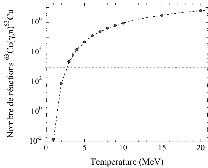
FIG. 5.17 – Evolution du nombre de réactions {}^{63}\text{Cu}(\gamma, n){}^{62}\text{Cu} induites dans un échantillon intégral en fonction de la température de la distribution des électrons. On considère un nombre d'électrons extrapolé à énergie nulle de 2.10^9 \text{ MeV}^{-1} .
