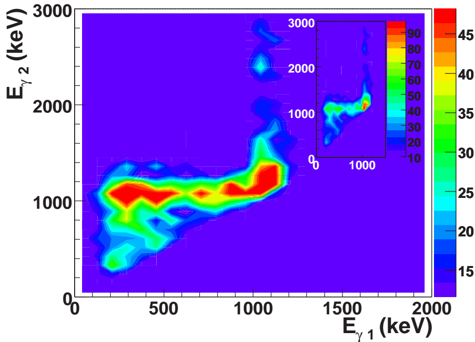
FIG. 7.14 – Spectres coïncidences du ^{38}\text{Si} . Seules les valeurs du nombre minimal et maximal de coïncidences diffèrent entre la figure en insert et celle exposée en grand. Le minimum est fixé à 10 pour les deux. Le maximum est arbitrairement porté à 48 dans la figure principale. Cette condition permet de mieux visualiser les autres coïncidences.
