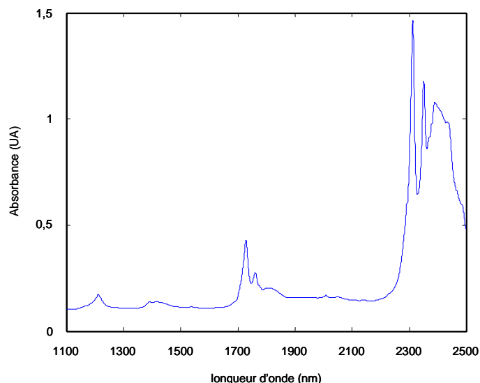
Figure 23 : Spectre PIR d'un film de PE de 210 µm
