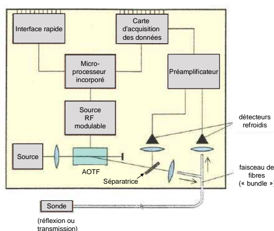
Figure 37 : Schéma d'un spectromètre AOTF type
