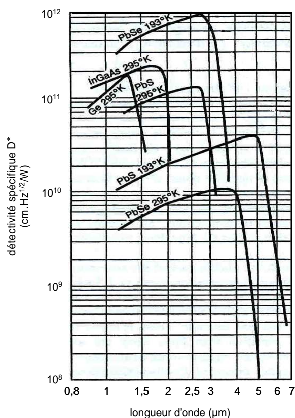
Figure 38 : Détectivité spécifique des principaux détecteurs proche infrarouge [72]
