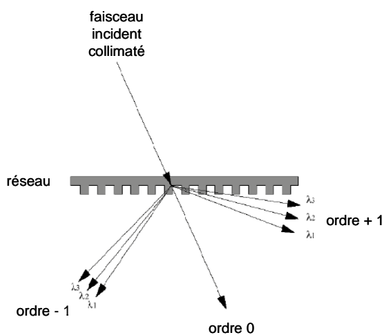
Figure 31 : Principe d'un réseau de diffraction en transmission
