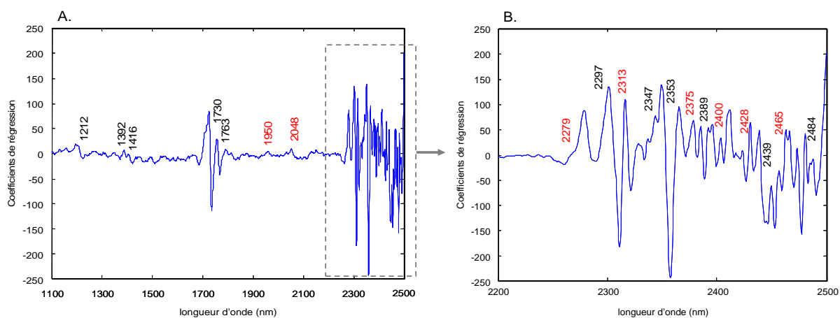
Figure 152 : Coefficients de régression du modèle prédictif du PE dans le tricouche PP-nylon-PE : A. entre 1100 et 2500 nm et B. entre 2200 et 2500 nm
