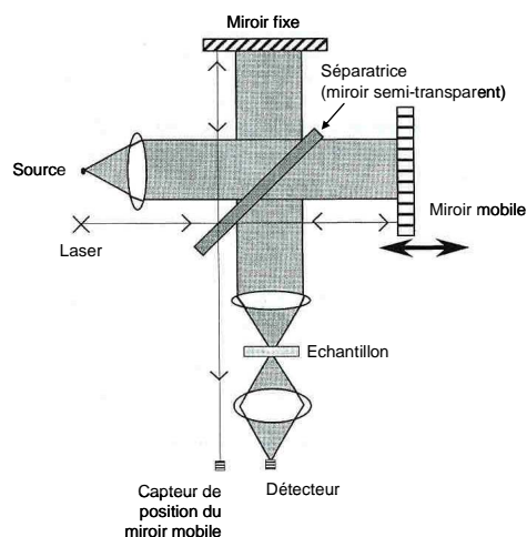
Figure 34 : Spectromètre PIR à transformée de Fourier basé sur le principe de l'interféromètre de Michelson [65]
