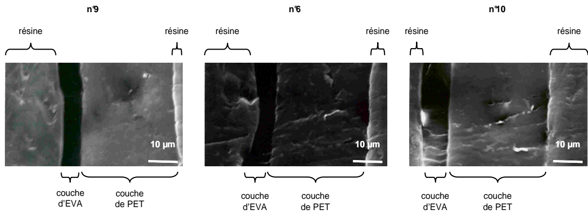
Figure 131 : Images MEB de trois échantillons particuliers
