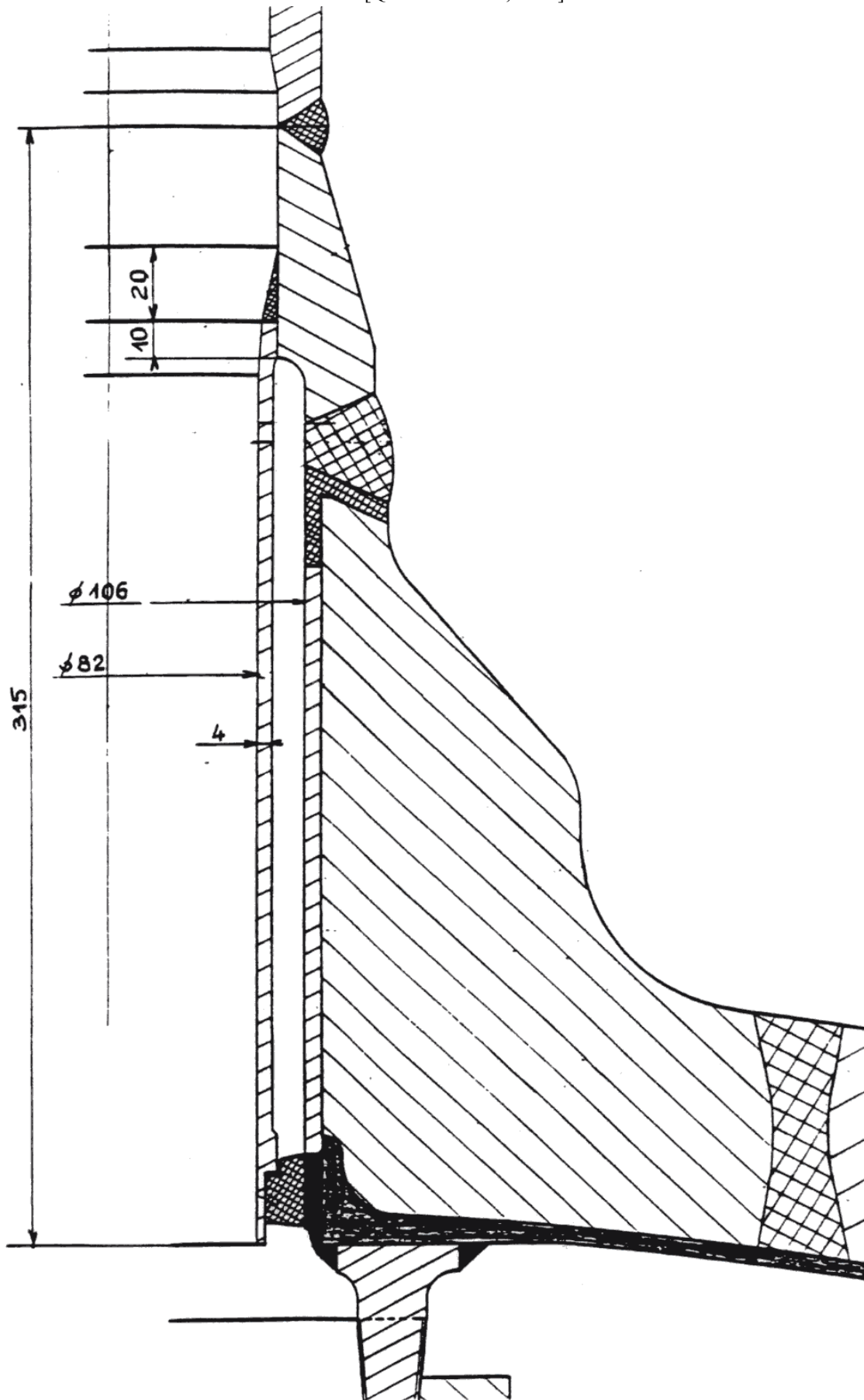
Schéma de la manchette thermique d'aspersion du pressuriseur Soudure circulaire - Tranches CP1 à CP4 [Quere et Michel, 1987]
