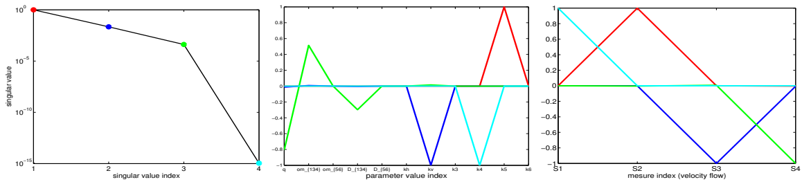
FIG. 7.15 – Date t_3 = 300\,000 ans - maillage fin
