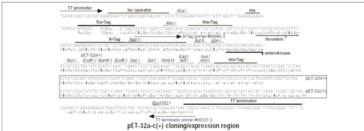
Carte du vecteur restriction du vecteur pET-32 utilisé pour le clonage et l'expression de protéines fusionnées à la thioredoxine.
