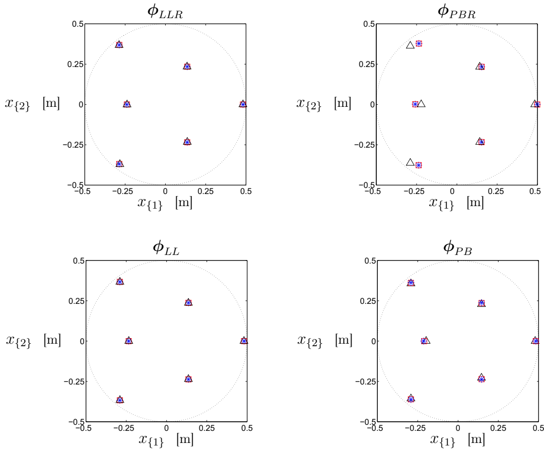
FIG. 5.3 – Protocoles optimaux pour les quatre jeux de fonctions de régression et n = 6 : (*) \sigma_e^2 = 4 \cdot 10^{-6} , ( \square ) \sigma_e^2 = 10^{-2} , ( \circ ) \sigma_e^2 = 4 \cdot 10^{-4} \text{ m}^2/\text{s}^2 .
