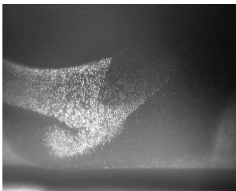
(e) Vortex.
