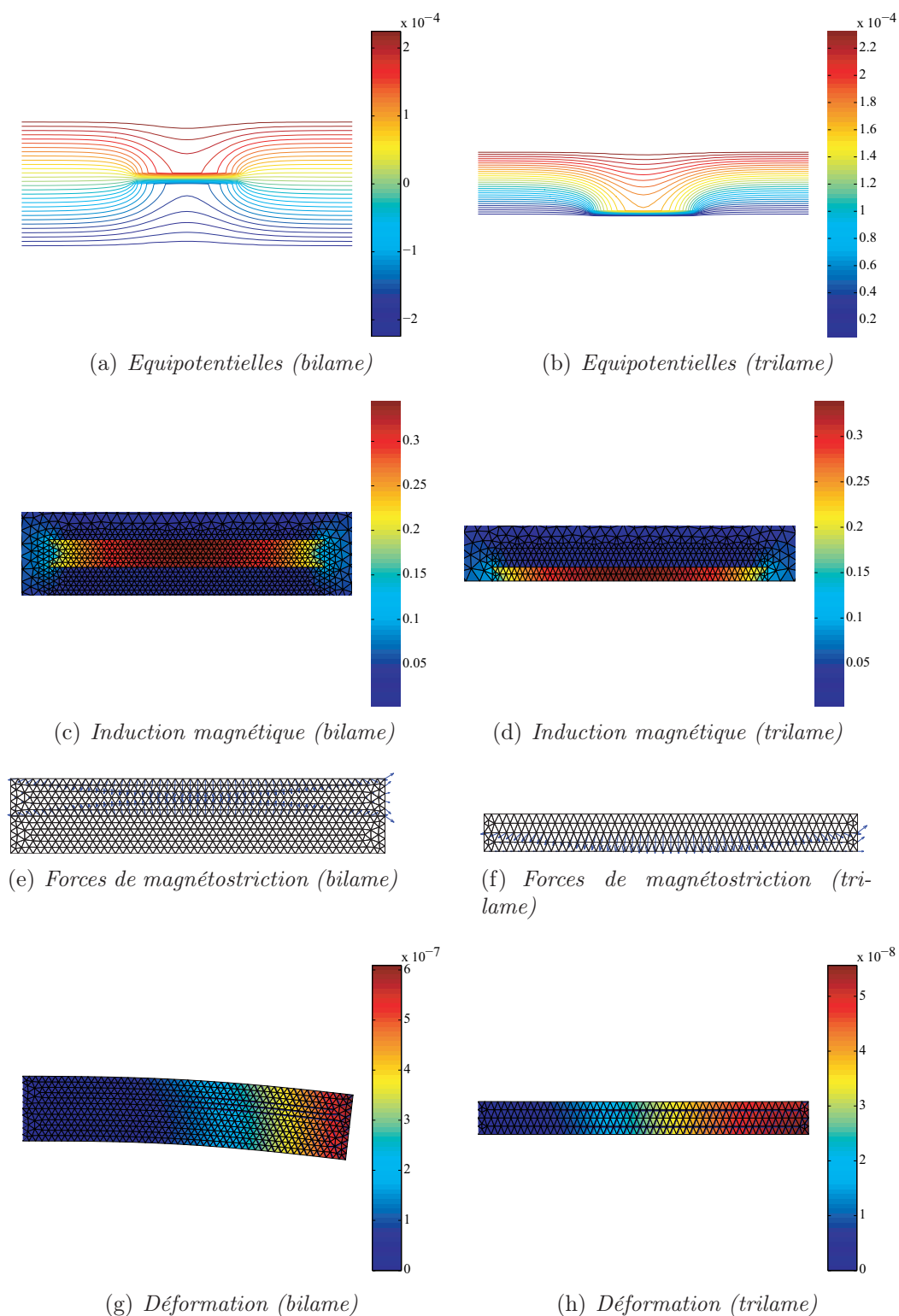
Figure 4.15 – Distribution des équipotentielle ( A ), de l'induction magnétique, des forces de magnétostriction et de la déformée totale
