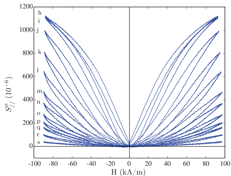
Figure 2.29 – Influence d'une contrainte de compression sur la mesure de la déformation de magnétostriction d'un barreau de Terfenol-D, comportement hystérique ( h = 9,6 \text{ MPa} i = 11,7 \text{ MPa} j = 19,6 \text{ MPa} k = 26,3 \text{ MPa} l = 33,1 \text{ MPa} m = 39,1 \text{ MPa} n = 44,3 \text{ MPa} o = 52,3 \text{ MPa} p = 58,7 \text{ MPa} q = 65,3 \text{ MPa} r = 83,5 \text{ MPa} s = 122,1 \text{ MPa} )
