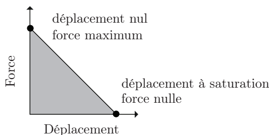
Figure 2.27 – Ligne typique de chargement mécanique quasi-statique
