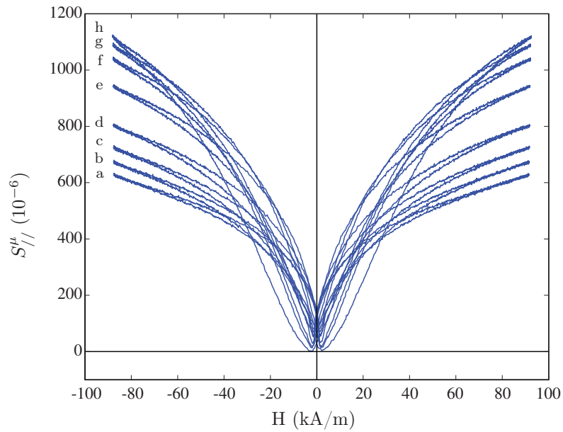
Figure 2.28 – Influence d'une contrainte de compression sur la mesure de la déformation de magnétostriction d'un barreau de Terfenol-D, comportement hystérique ( a = 0 \text{ MPa} b = 0,4 \text{ MPa} c = 0,6 \text{ MPa} d = 1,2 \text{ MPa} e = 2,7 \text{ MPa} f = 4,6 \text{ MPa} g = 6,2 \text{ MPa} h = 9,6 \text{ MPa} )
