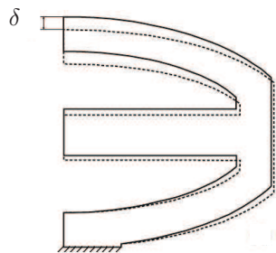
Figure 4.2 – Déplacement \delta à une excitation magnétique
