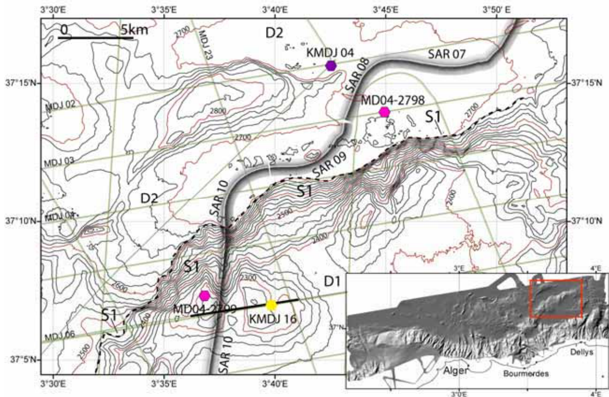
Figure III-55 : Carte bathymétrique montrant l'escarpement S1, la localisation des profils SAR 07, 08, 09 et 10, ainsi que la localisation des carottes disponibles dans cette zone : MD04-2799 et KMDJ 16 en haut de pente et KMDJ 04 et MD04-2798 dans le bassin D2.
