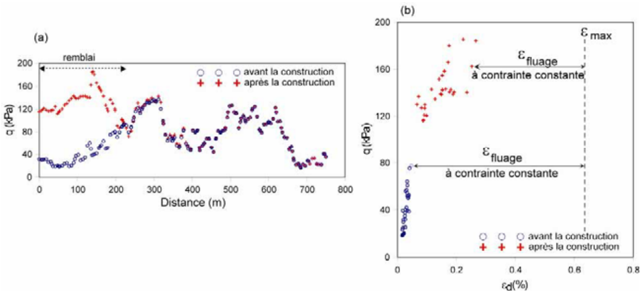
Figure IV-48: (a) Déviateur des contraintes (q) avant et après la construction sur la plateforme de l'aéroport le long de la surface de glissement de 1979 et (b) Déviateur des contraintes vs déformation le long de la surface de glissement de 1979.
