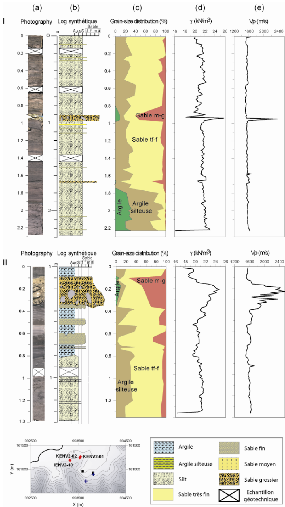
Figure IV-30 : Description et mesures réalisées sur les carottes I-KENV2-01 et II-KENV2-02 avec (a) la photographie, (b) le log synthétique, (c) les courbes de granulométrie, (d) mesure du poids volumique et (e) mesures de Vp.
