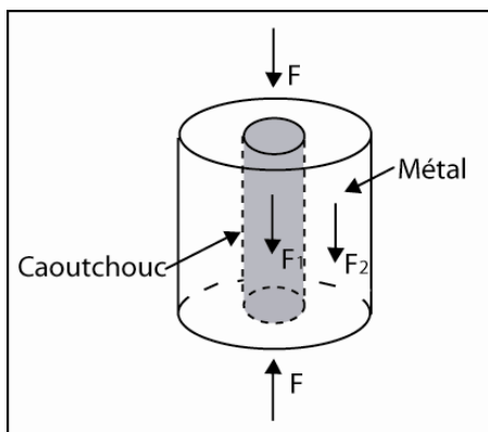
Figure I-2: Exemple de la répartition des contraintes (d'après Schlosser, 2003).
