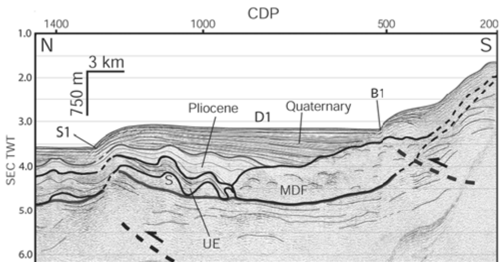
Figure III-23 : Profil sismique 6 traces, migré en temps (localisation ligne A sur la figure III-22). S - sel ; MDF - Cône détritique messinien ; UE - évaporites supérieures (toit à 5.3 Ma) ; S1 et B1 - ruptures de pente. Lignes en pointillés correspondent à des failles inverses (traduit d'après Déverchère et al., 2005).
