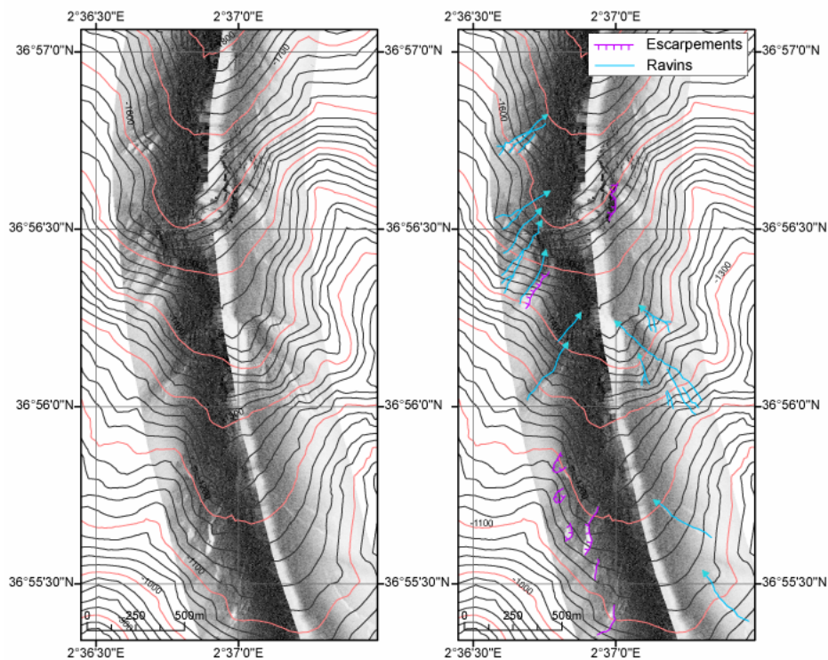
Figure III-83 : Image SAR 21 montrant la partie haute de la pente continentale au large du Banc de Khayr al Din avec (a) image SAR brute et (b) image SAR interprétée.
