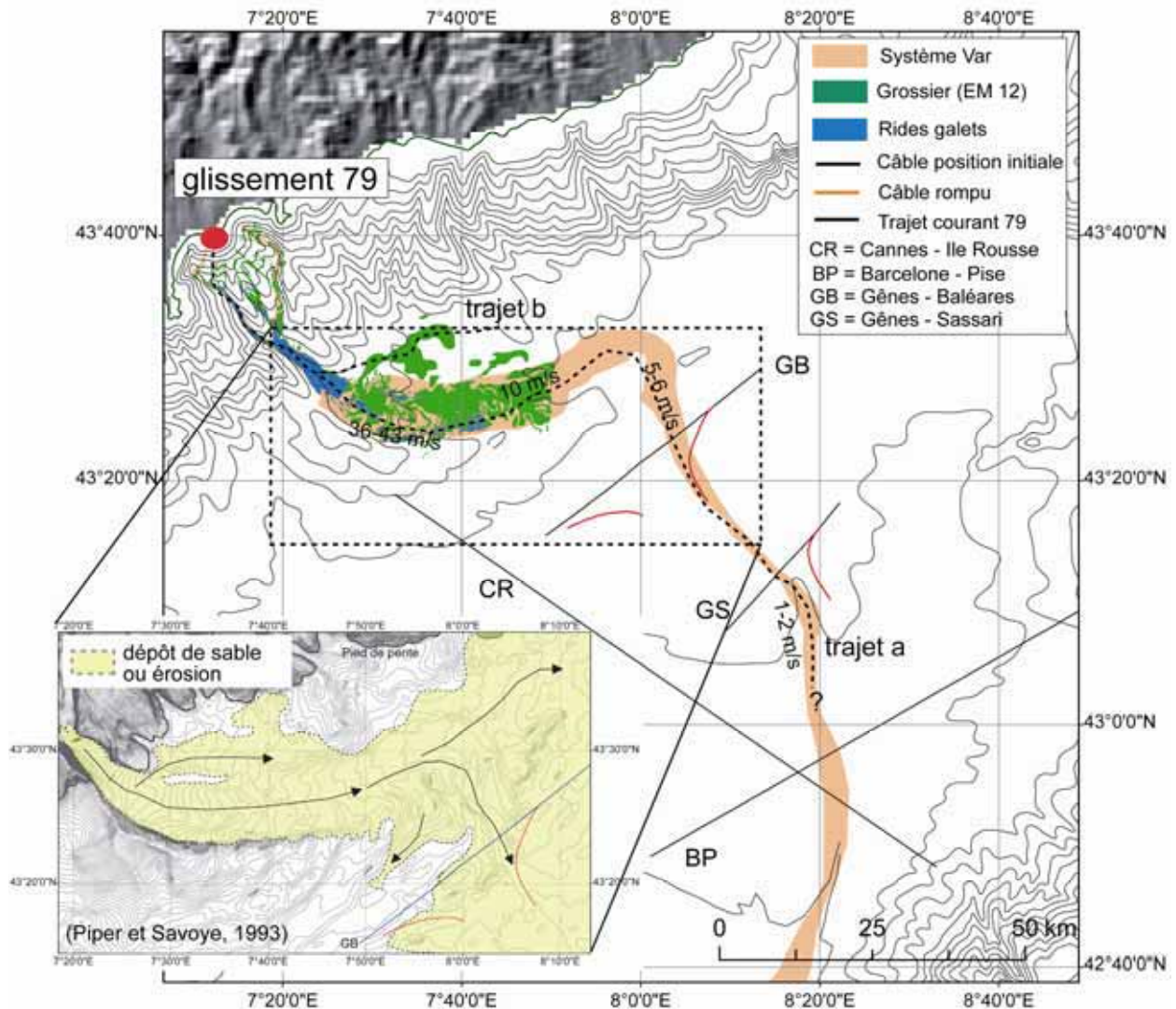
Figure IV-11 : Carte bathymétrique générale de la Baie des Angers montrant le trajet du courant turbiditique de 1979, les câbles de télécommunication (Genneveux et al., 1980) qui passent dans la zone, les estimations des vitesses du courant (Mulder et al., 1997). Zone bleu = rides des galets mis en évidence à partir de données SAR et zone verte - dépôts grossiers à partir de l'interprétation de l'imagerie EM 12 (SIG Var, IFREMER). Zoom : carte montrant la distribution du niveau de sable et des évidences d'érosion à partir de carottages et l'interprétation des profils Boomer (d'après Piper et Savoye, 1993) (Mercator, WGS 1984).
