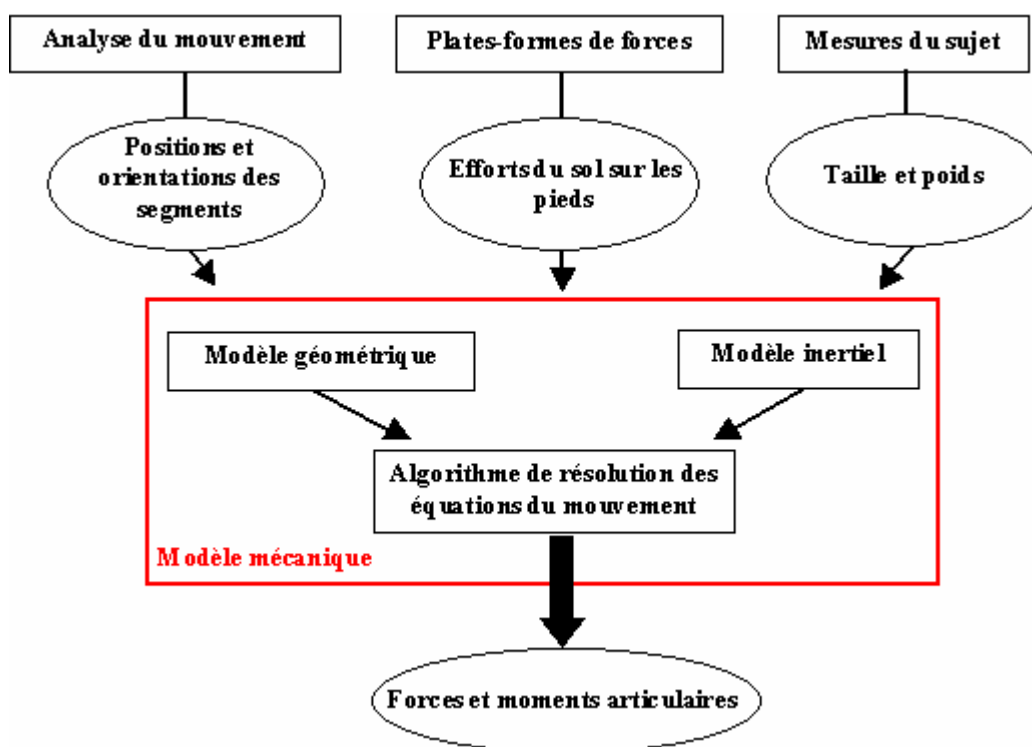
Figure IV.5 : Schéma de principe du calcul des forces et des moments articulaires.
