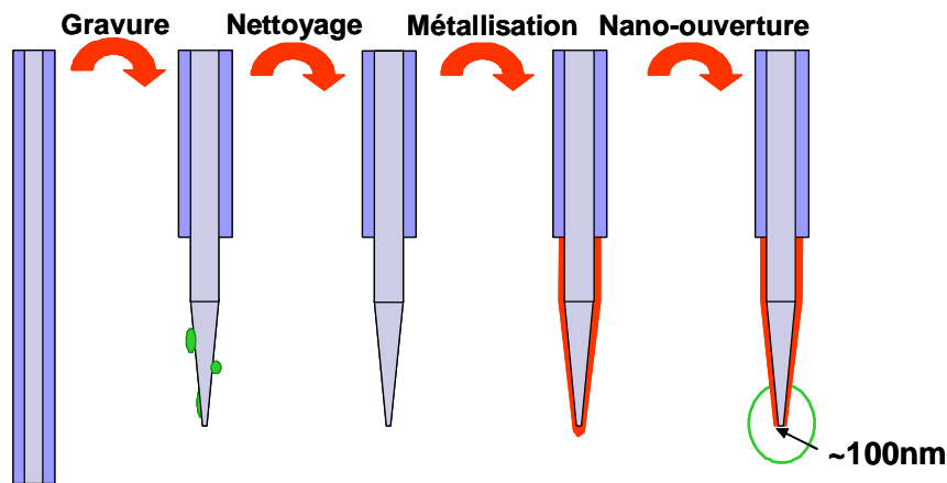
Fig. III.1 : Procédé IMN de fabrication des nano-sondes en 4 étapes [1-3].
