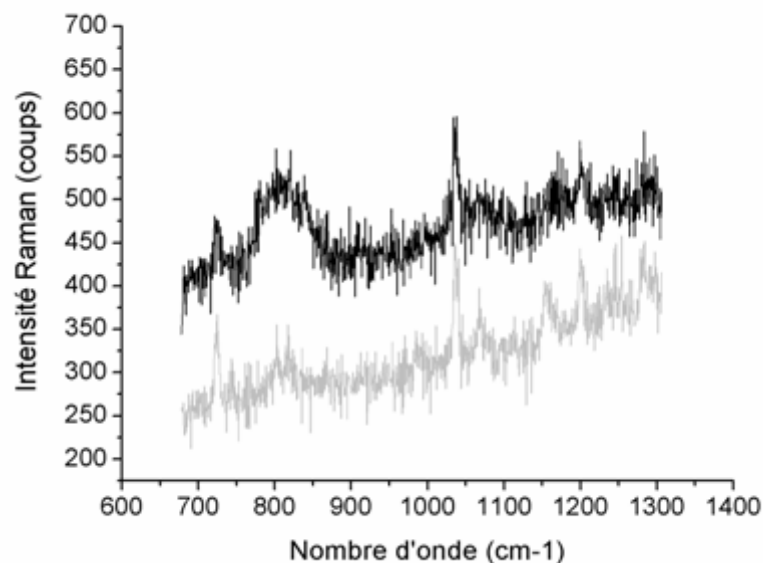
Fig. V.23 : Spectres Raman du tétrahydronaphtalène collectés par le micro-capteur pour deux longueurs de fibres différentes, 3 mètres courbe noire, 1 mètre courbe grise ( \lambda= 514,5 nm, P=300 mW, t=300 s).
