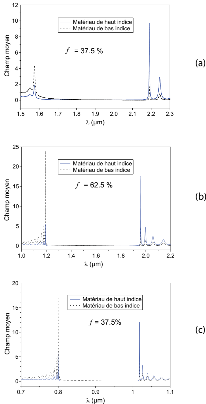
Fig. 2.9 – Spectre de l'intensité du champ E.M. moyen dans un des matériau d'un cristal photonique 1D de 20 paires de couches avec ( n_1 = 1.6 ) et ( n_2 = 3.5 ) et une période de \Lambda = 0.32 \mu\text{m} : (a) Au voisinage de la première bande interdite pour un facteur de remplissage du matériau de bas indice f = 0.37 , (b) Au voisinage la première bande interdite pour un facteur de remplissage du matériau de bas indice f = 0.62 , (c) Au voisinage la deuxième bande interdite pour un facteur de remplissage du matériau de bas indice f = 0.37 .
