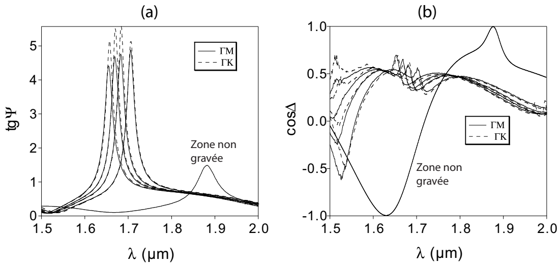
Fig. 3.17 – Mesures ellipsométriques \text{tg}\Psi (a) et \cos\Delta (b) effectuées sur 4 CPs gravés dans un même substrat pour \theta = 75^\circ et dans les 2 directions de haut symétrie du cristal \Gamma M (traits pleins) et \Gamma K (pointillés).
