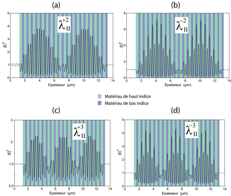
Fig. 2.8 – Distribution de l'intensité du champ E.M dans un cristal photonique 1D de 20 paires de couches d'épaisseurs optiques ( \lambda_0/4 ) et ( \lambda_0/2 ) au voisinage de la 1 re bande interdite, avec \lambda_0 = 1 \mu\text{m} et \Delta n = \frac{n_2}{n_1} = 1.42 : (a) et (b) Aux 2 es maximums de transmission de part et d'autre de la 2 e bande interdite. (c) et (d) Aux 3 es maximums de transmission de part et d'autre de la 2 e bande interdite.
