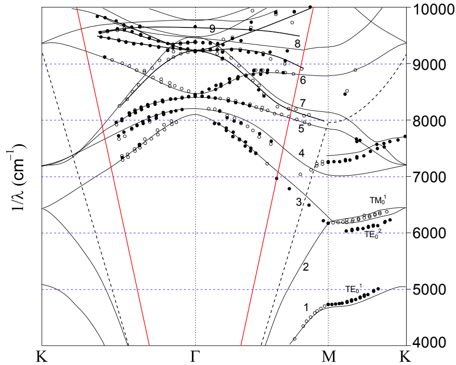
Fig. 4.16 – Diagramme de dispersion complet du CP_1 obtenu expérimentalement pour les deux polarisations p (cercles pleins) et s (cercles vides), et pour les directions de haut symétrie \mathbf{\Gamma M} , \mathbf{\Gamma K} et \mathbf{MK} entre 4000 < 1/\lambda < 10000 \text{ cm}^{-1} . Les courbes sont déployés tenant compte de la symétrie venant des nouvelles conditions aux limites. Les courbes en trait continu représentent les courbes théoriques et les bandes sont numérotés à partir du point \mathbf{\Gamma} . [Photonic band structure for CP_1 from transmission and reflection measurements for p (full circles) and s (empty circles) polarizations for frequency between 4000 < 1/\lambda < 10000 \text{ cm}^{-1} . Theoretical (lines) and experimental (points) unfolded dispersion curves in the \mathbf{\Gamma K} , \mathbf{\Gamma M} and \mathbf{MK} directions, taking into account the symmetries coming out from boundary conditions. Bands are labelled according to their frequency at the \mathbf{\Gamma} point.]
