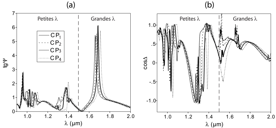
Fig. 3.16 – Mesures ellipsométriques \text{tg}\Psi (a) et \cos\Delta (b) effectuées de 0.9 à 2 \mu\text{m} sur 4 CPs gravés dans un même substrat pour \theta = 75^\circ et dans la direction \Gamma K .
