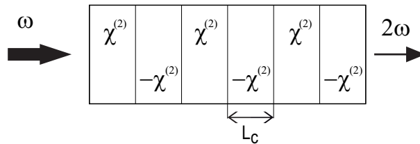
Fig. 1.18 – Cristal photonique non linéaire à une dimension où le QAP est réalisé par inversion du signe de \chi^{(2)} pour chaque longueur de cohérence L_C . [Non linear one-dimensional photonic crystal of \chi^{(2)} . quasi-phase matching is achieved by inversion of the \chi^{(2)} sign for each coherence length.]
