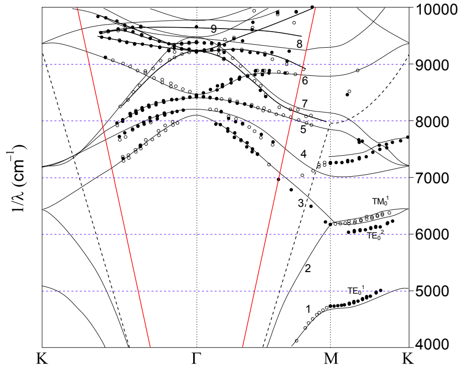
Fig. 4.16 – Diagramme de dispersion complet du CP_1 obtenu expérimentalement pour les deux polarisations p (cercles pleins) et s (cercles vides), et pour les directions de haut symétrie \mathbf{\Gamma M} , \mathbf{\Gamma K} et \mathbf{MK} entre 4000 < 1/\lambda < 10000 \text{ cm}^{-1} . Les courbes sont déployés tenant compte de la symétrie venant des nouvelles conditions aux limites. Les courbes en trait continu représentent les courbes théoriques et les bandes sont numérotés à partir du point \mathbf{\Gamma} . [Photonic band structure for CP_1 from transmission and reflection measurements for p (full circles) and s (empty circles) polarizations for frequency between 4000 < 1/\lambda < 10000 \text{ cm}^{-1} . Theoretical (lines) and experimental (points) unfolded dispersion curves in the \mathbf{\Gamma K} , \mathbf{\Gamma M} and \mathbf{MK} directions, taking into account the symmetries coming out from boundary conditions. Bands are labelled according to their frequency at the \mathbf{\Gamma} point.]
