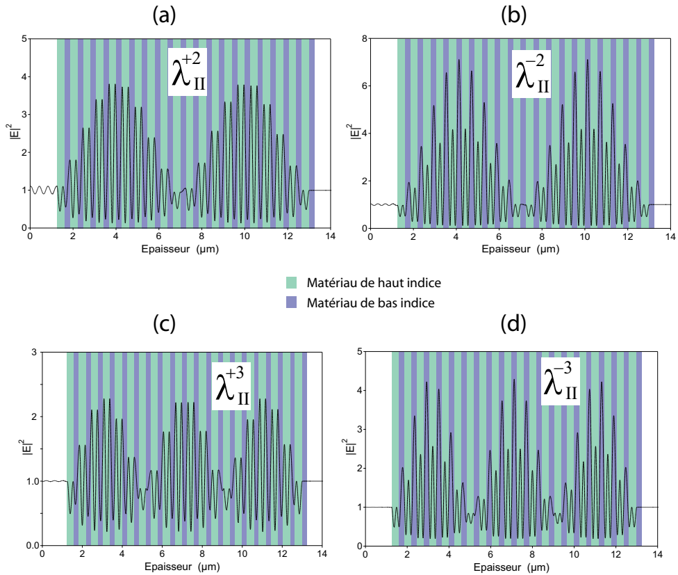
Fig. 2.8 – Distribution de l'intensité du champ E.M dans un cristal photonique 1D de 20 paires de couches d'épaisseurs optiques (\lambda_0/4) et (\lambda_0/2) au voisinage de la 1 re bande interdite, avec \lambda_0 = 1 \mu\text{m} et \Delta n = \frac{n_2}{n_1} = 1.42 : (a) et (b) Aux 2 es maximums de transmission de part et d'autre de la 2 e bande interdite. (c) et (d) Aux 3 es maximums de transmission de part et d'autre de la 2 e bande interdite.
