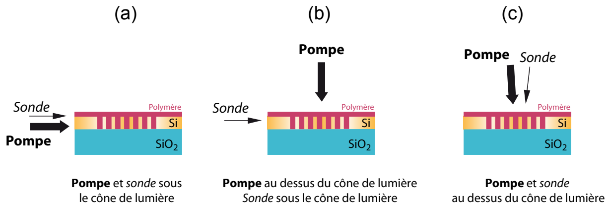
Fig. 4.23 – Configurations schématiques des manipulations pompe/sonde dans des CPs 2D en SOI doublement résonnants. [ Schematic pump/probe configurations in 2D photonic crystals made in SOI substrate. ]
