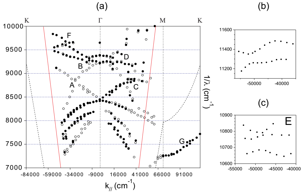
Fig. 4.22 – (a) : Structure de bandes photonique du CP_1 entre 7000 < \frac{1}{\lambda} < 10000 cm^{-1} pour les deux polarisations p et s mesurée à partir des spectres de transmission et de réflexion montrant les points de croisement et anti-croisement entre . (b) (c) :Détail des courbes de dispersions sur des points d’anti-croisement obtenu par l’identification des résonances de Fano sur des spectres de tg\Psi obtenus par ellipsometrie spectroscopique .
