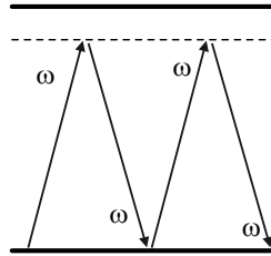
Fig. 1.3 – Diagramme quantique associé à l'effet Kerr optique. Deux photons lasers sont absorbés et deux autres émis, laissant l'énergie du milieu non linéaire inchangée.
