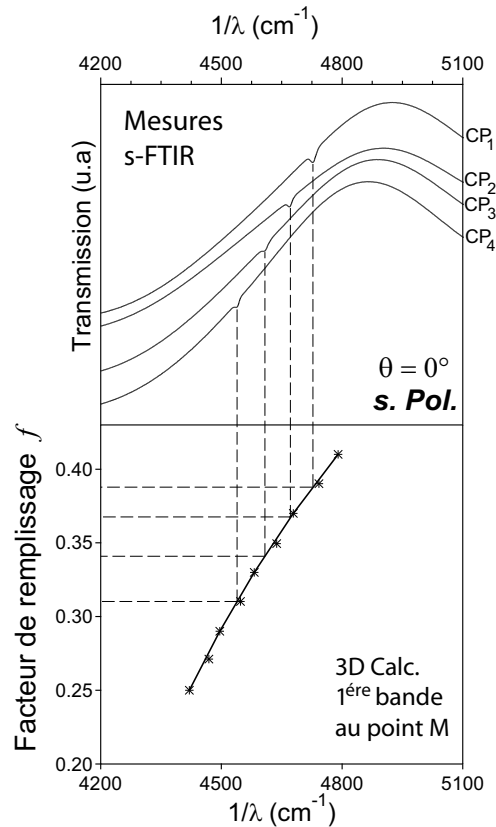
Fig. 4.19 – Spectres de transmission aux grandes longueurs d’onde obtenus entre 4200 < \frac{1}{\lambda} < 5100 \text{ cm}^{-1} avec la s-FTIR pour une polarisation s et pour \theta = 0^\circ . On voit l’apparition de la résonance de Fano pour les 4 CPs (figure d’en haut). Figure d’en bas : Calcul de la position en fréquence des modes guidés autour du point M en fonction du facteur de remplissage f . [Transmission spectra at large wavelength for frequency between 4200 < \frac{1}{\lambda} < 5100 \text{ cm}^{-1} obtained by s-FTIR measurements for s-polarization and for \theta = 0^\circ . We See the appearance of Fano resonance within the 4 CPs (figure of in top). Figure in bottom : Calculation of the frequency position of guides modes around the M point by variation of the filling factor f .]
