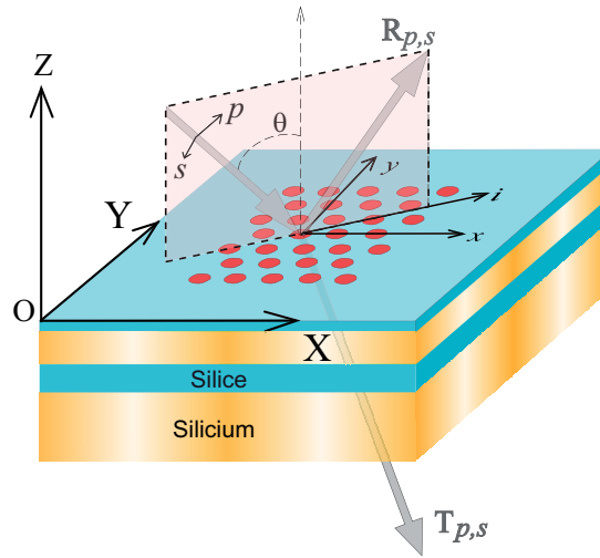
Fig. 3.15 – Description de la géométrie du cristal photonique utilisée en E.S et spectrométrie FTIR. Le cristal photonique est dans le plan (X, Y) . Le vecteur d'onde incident k(\omega) et l'axe Z normal à la surface du cristal photonique définissent le plan d'incidence.
