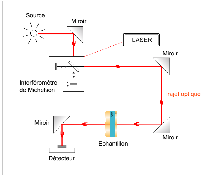
Fig. 3.11 – Principe du spectromètre FTIR (Nicolet Nexus 870). [Spectrometer FTIR principle (Nicolet Nexus 870).]
