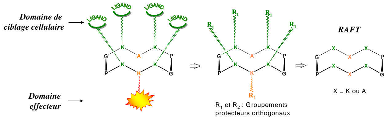
Figure 21 : Schéma du RAFT utilisé pour la vectorisation en cancérologie.
