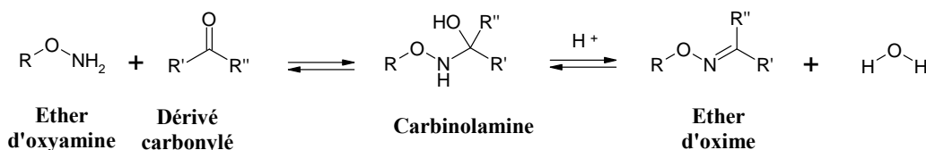
Figure 47 : Mécanisme de formation de la liaison éther d'oxime.
