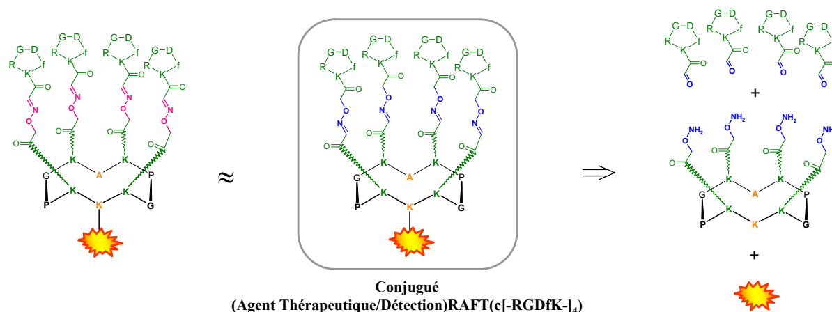
Figure 22 : Schéma de la construction des conjugués RAFT(c[-RGDfK-] 4 ).
