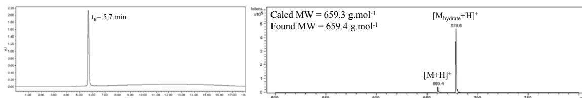
Figure 45 : Chromatogramme CLHP et spectre de masse ESI du composé 36 .
