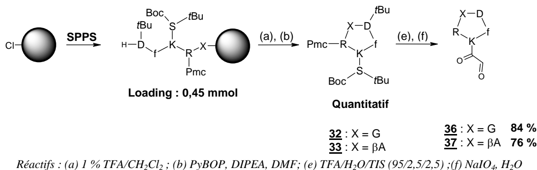
Figure 46 : Schéma de la voie de synthèse optimisée de c[-RXDfK(CO-CHO)-].
