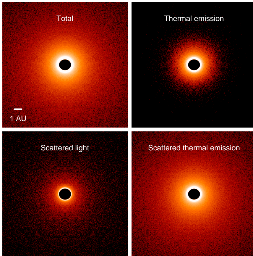
FIG. 69. Images simulées pour le meilleur modèle ajustant les visibilités et la photométrie obtenues en séparant les différentes contributions à l'intensité. De gauche à droite, de haut en bas : carte de l'intensité totale, de l'émission thermique uniquement, de l'émission diffusée, et de l'émission thermique diffusée.
