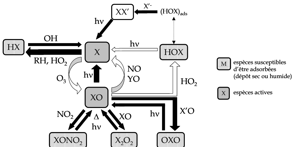
Figure I-5 : schéma simplifié des réactions entre espèces halogénées actives et réservoirs en atmosphère marine (X = Br, Cl) d'après Platt et Hönninger [2002]
