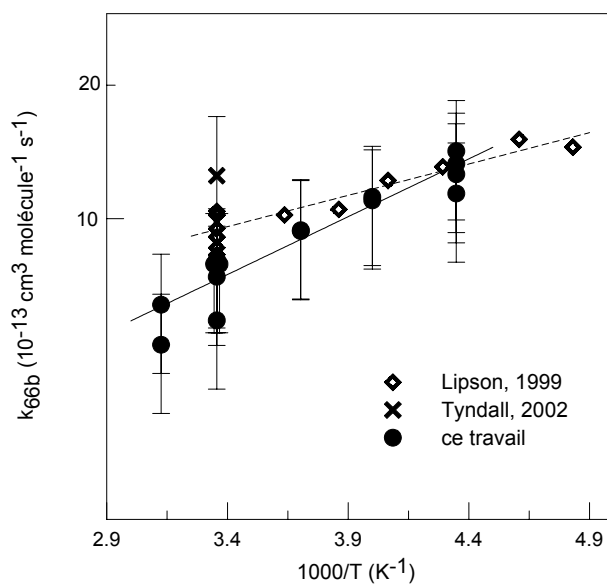
Figure III-45 : réaction \text{ClO} + \text{OH} \rightarrow \text{HCl} + \text{O}_2 comparaison avec la littérature
