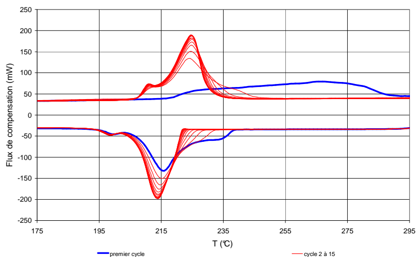
Figure 3.42 : Flux de compensation vs température pour des composites à base de \text{KNO}_3/\text{NaNO}_3 et de graphite naturel rebroyé mis en forme par le SGL ayant subi 15 cycles de refroidissement) et de réchauffement à 5^\circ\text{C}/\text{min} .
