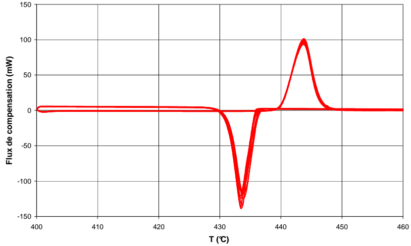
Figure 3.50 : Flux de compensation vs température pour le binaire \text{NaCl/MgCl}_2 mélangé à 10% de SFG150 ayant subi 20 cycles de refroidissement et de réchauffement à 20^\circ\text{C}/\text{min} .
