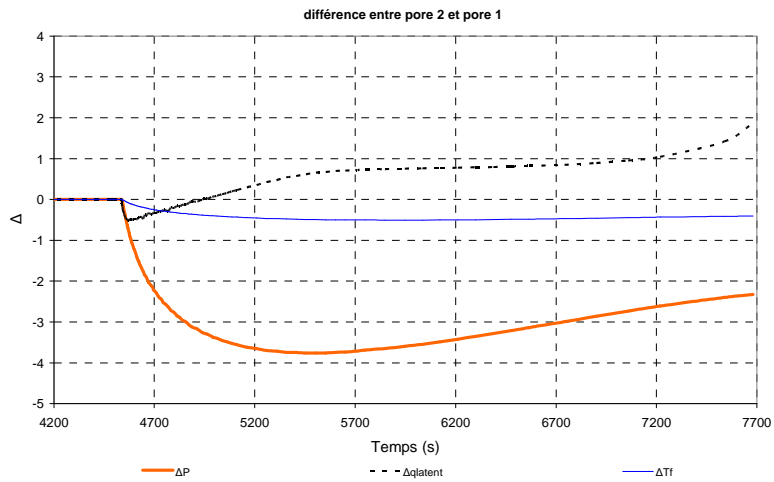
(a) différence de pression, de température de fusion et de flux de chaleur latente entre le pore 2 et le pore 1.
