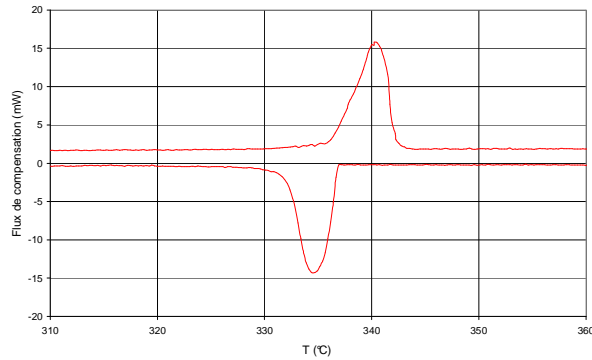
(a) KNO_3
