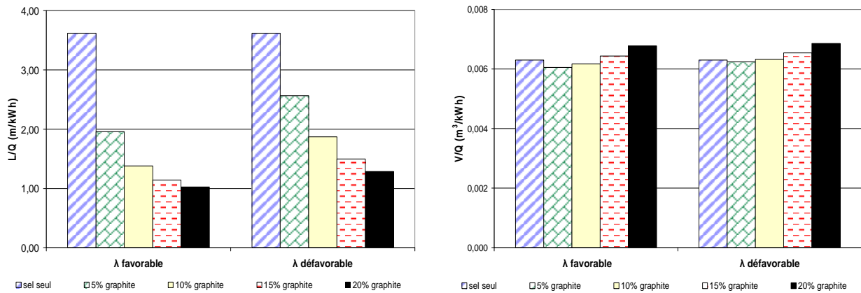
Figure 1.27 : Dimensions de l'échangeur (gauche) et du système de stockage (droite) en fonction de la conductivité thermique des composites et du pourcentage de graphite pour une capacité de 100kWh, un temps de charge de deux heures et une température de travail de 600°C .
