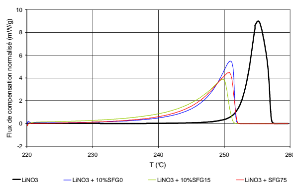
Figure 3.24 : Influence de la quantité de graphite sur la cinétique de fusion du \text{LiNO}_3 .
