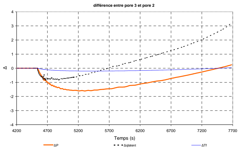
(b) différence de pression, de température de fusion et de flux de chaleur latente entre le pore 3 et le pore 2.
