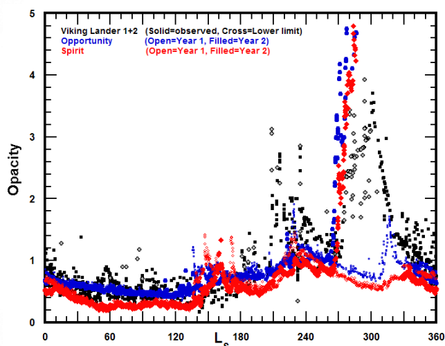
2.3.b Atténuation enregistrée au sol [Clancy et al., 2000]
