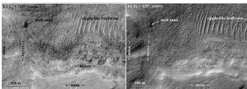
Fig. 2.14. Une surface changeante ? [Fenton, 2005] Image MOC (a) E0200791 (b) E1400275 {332.24°W ; 45.67°S}
