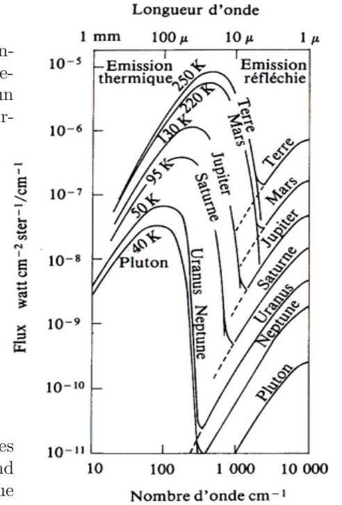
Fig. 4.5. Spectres thermiques et réfléchis des planètes
