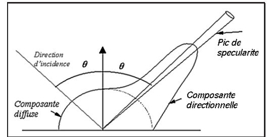
Fig. 5.8. Décomposition du lobe de diffusion (voir aussi Fig. 4.1.b)
