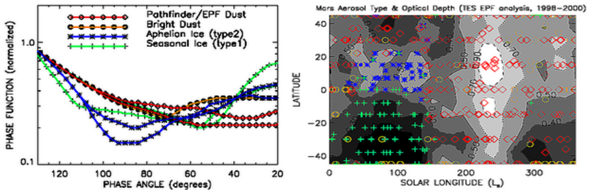
2.6.a Fonction de phase pour différents types d'aérosols. 2.6.b Répartition latitudinale et type d'aérosols saisonnières
