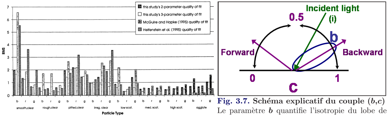
Fig. 3.6. Comparaison entre les modèles : Le résidu dépend des particules [Hartman et al., 1996]
