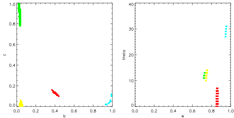
Fig. 3.8. Distribution des paramètres de Hapke vis à vis des angles d'émergence Impact d'une différence de \pm 1^\circ . Le paramètre c est mal contraint pour le point Green, de même que le paramètre \bar{\theta} pour le point Red.
