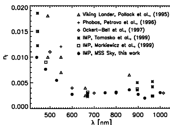
4.7.b Indice de réfraction imaginaire [Markiewicz et al., 2002]
