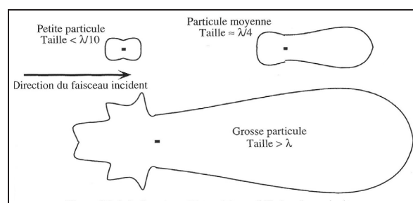
Fig. 3.9. Indicatrices d'intensités des particules [Meysonnette and Lepine, 2001]
