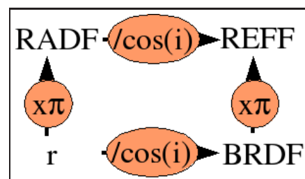
Fig. 2.8. Relation entre les différentes définitions de réflectances
