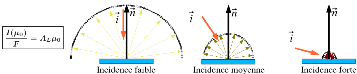
Fig. 5.1. Modèle de Lambert : Variation des réflectances en fonction de l'incidence
