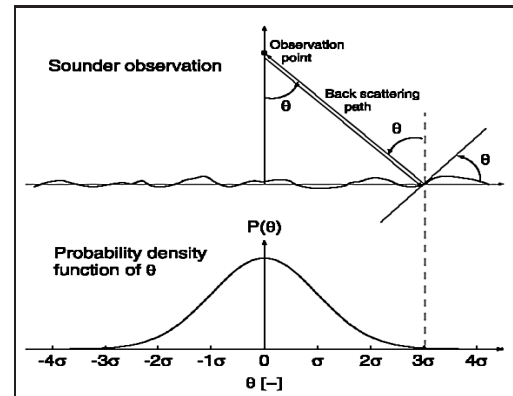
Fig. 5.9. Proportion spéculaire restante [Kobayashi and Ono, 2006].
