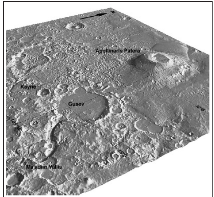
Fig. 1.1. Gusev et ses alentours [Greeley et al., 2003] Image 'ombrée' générée à partir des données MOLA .
