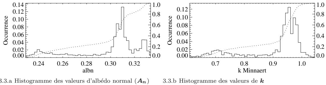
Fig. 3.3. Distribution des valeurs des paramètres de Minnaert
