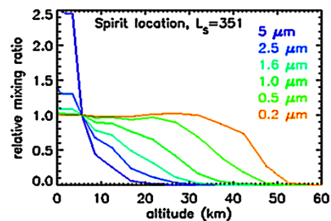
Fig. 2.4. Distribution de taille avec l'altitude mesurée conjointement par MGS et Spirit [Wolff et al., 2006].
