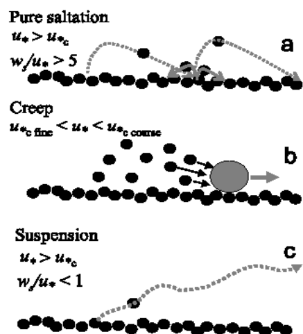
2.16.a Modes de transport éolien
