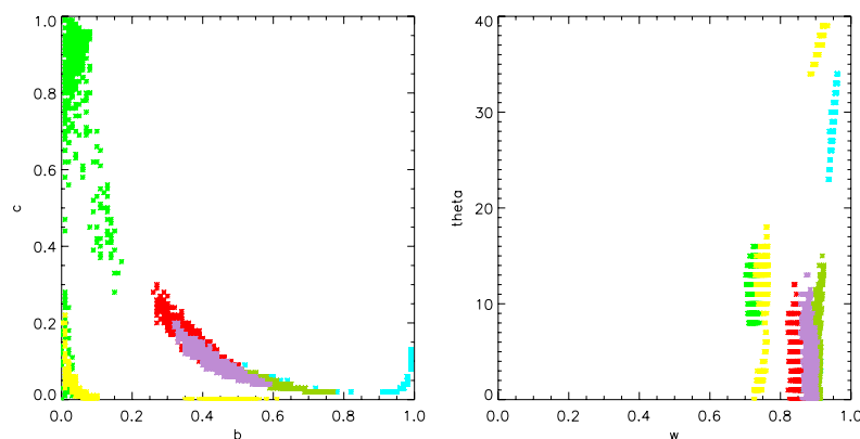
Fig. 3.7. Distribution des paramètres de Hapke vis à vis de la réflectance Impact sur l'inversion d'une différence minimale de réflectance (RADF) de 0.005
