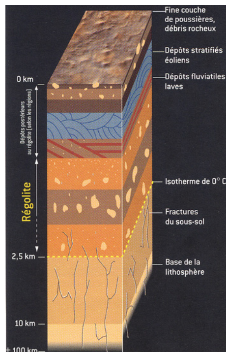
Fig. 2.10. Structure présumée du sous sol de Mars [Forget et al., 2003].
