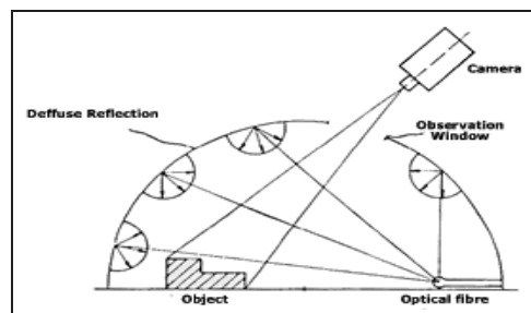
Fig. 2.10. Méthode de mesure : R_{hd}
