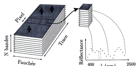
Fig. 1.2. Imagerie hyperspectrale : les images sont acquises simultanément pour plusieurs canaux spectraux
