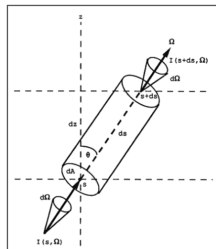
Fig. 4.8. Cylindre élémentaire
