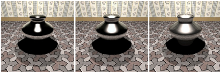
Fig. 5.2. Étalement sur une sphère du lobe de spécularité pour n= 10,50,100
