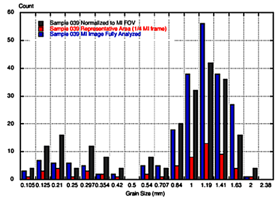
Fig. 1.9. Distribution en taille des particules à la surface : MI sol : 39bleu/rouge/gris : surface totale /25% du centre/normalisé
