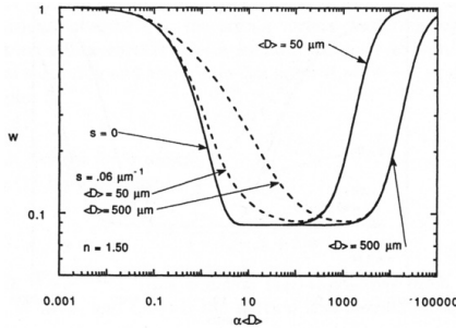
Fig. 3.2. Zone de diffusion de w
