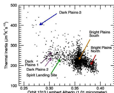
1.2.b Albédo et inertie thermique
