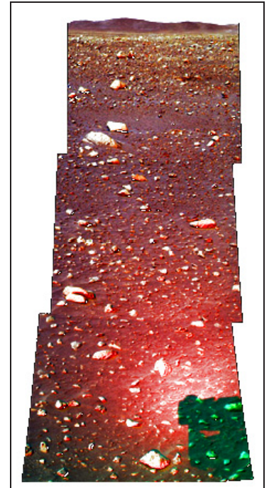
Fig. 4.18. Effet d'opposition autour de l'ombre du mât du rover Spirit
