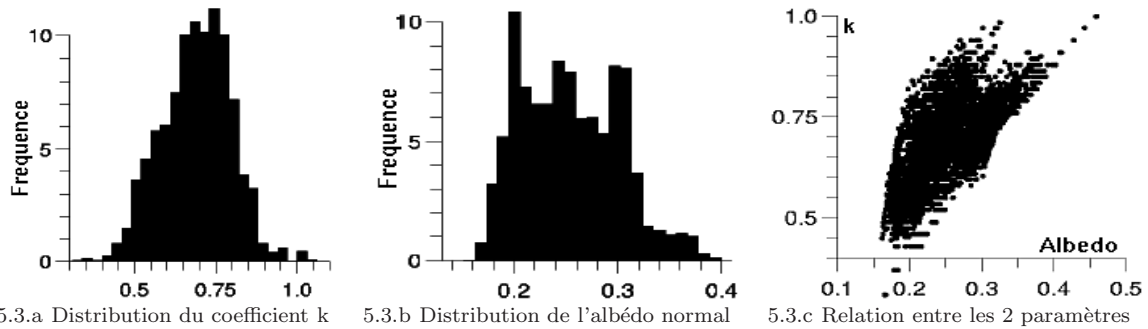
Fig. 5.3. Paramètres de Minnaert retrouvés pour la planète Mars \lambda = 0.73\mu\text{m} observations au Pic du Midi (1988) [de Grenier and Pinet, 1995, Pinet and Rosemberg, 2001].
