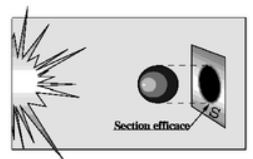
Fig. 4. Représentation d'une section efficace
