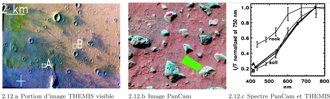
Fig. 2.12. Diversité spectrale orbitale et in situ [Lichtenberg et al., 2006]. (a) Portion d'image THEMIS visible V10792003 dans la zone d'atterrissage de Spirit (croix blanche) en utilisant les filtres 425, 540 et 654nm. L'incidence est de 75°. [McConnochie et al., 2006] (b) Image PanCam pour les unités 'rock' et 'soil'. L'image est composée des filtres 750, 530 et 480 nm. (c) Spectre I/F PanCam et THEMIS (ligne épaisse) normalisé à 750nm des zones précédentes.
