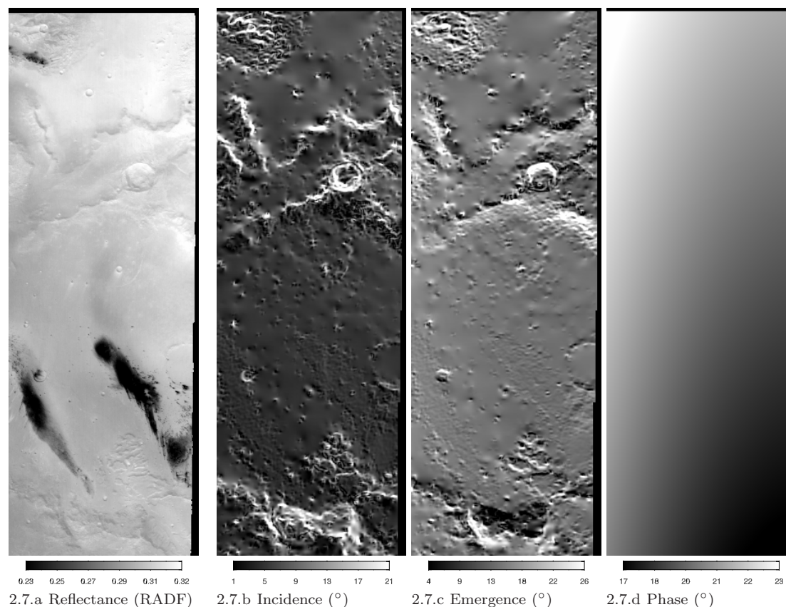
Fig. 2.7. Données pour la configuration 2271p1
