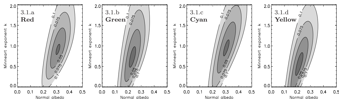
Fig. 3.1. Calcul des scores dans tout l'espace des paramètres (méthode directe) : la couleur gris foncé correspond à un écart en RADF de 0.025.
